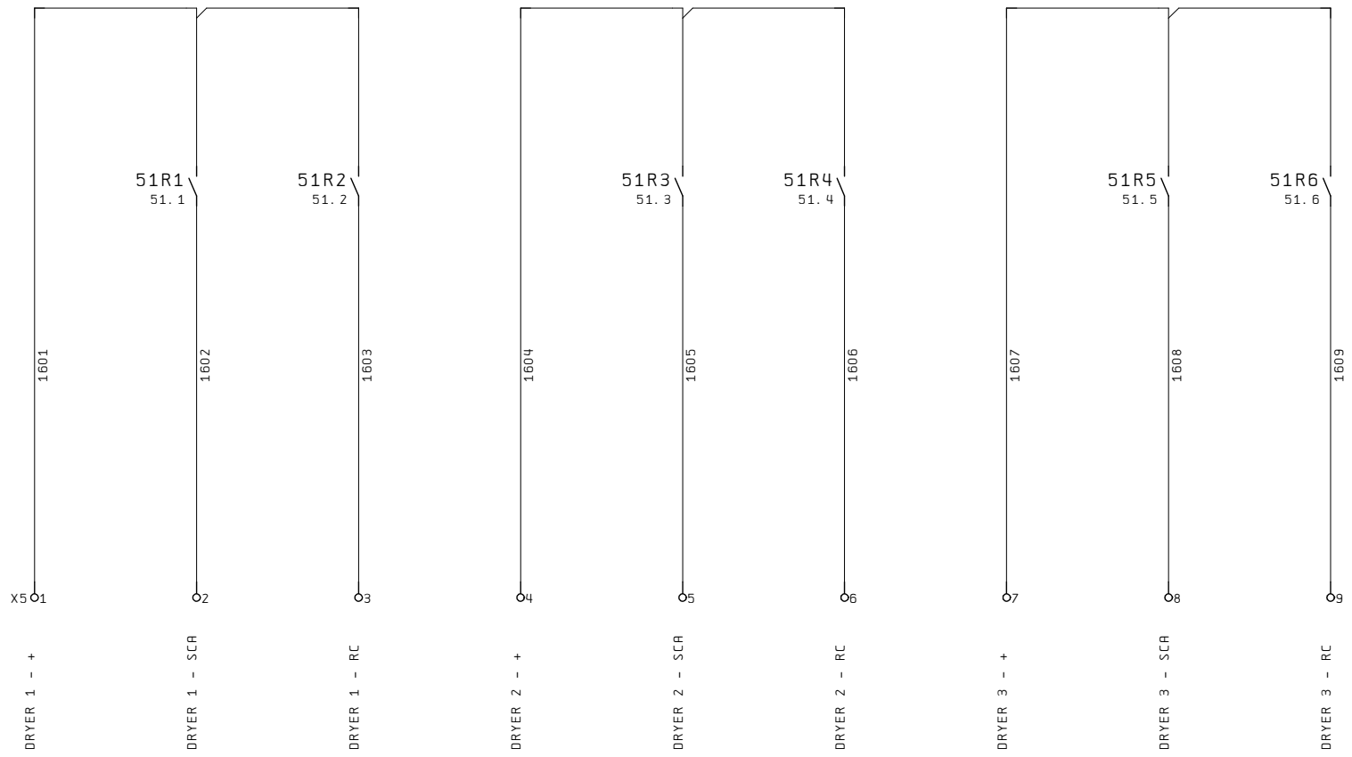
DRYER 1 004601JK001
