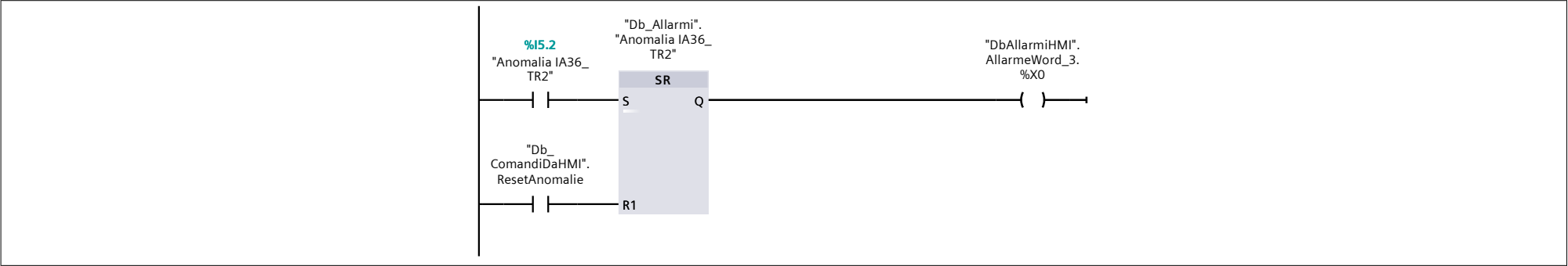
Segmento 52: INTERSCAMNIO - TERMICO MOTORE elevatore interscambio ok sup
