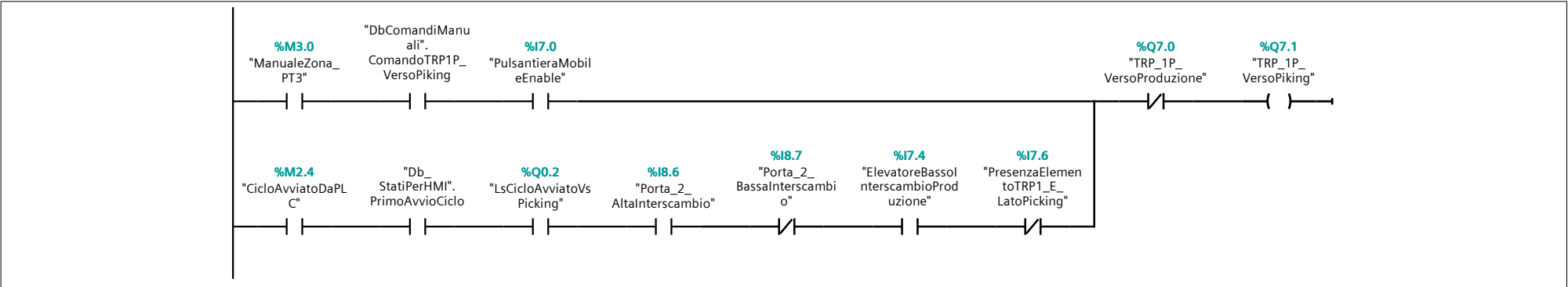
Segmento 8: Rotazione TRP-1P Verso Produz.
