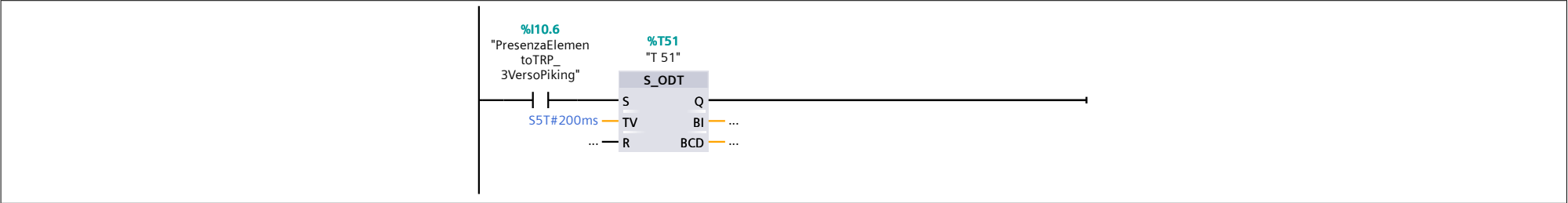
Segmento 7: Rotazione Indietro TRP-4 Frigo
