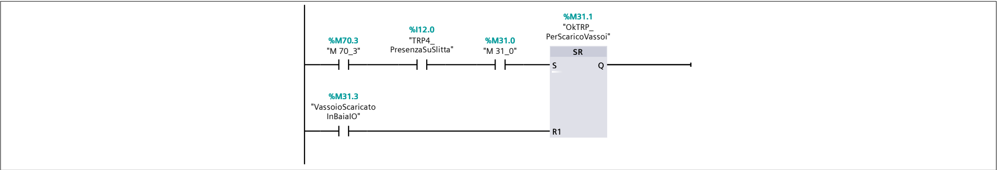
Segmento 4: Aus. Transito vassoio in Scarico
