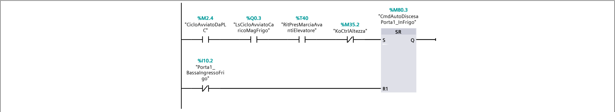
Segmento 6: Comando automatico - Discesa Porta 1 Trasf. da Frigo
