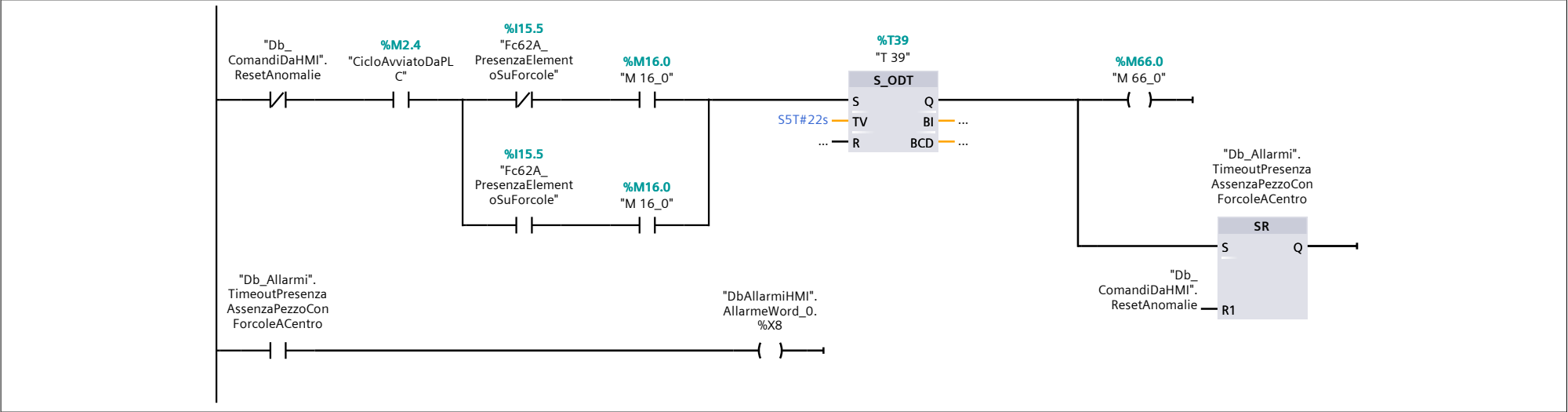
Segmento 10: Time-Out presenza elevat. Piking
