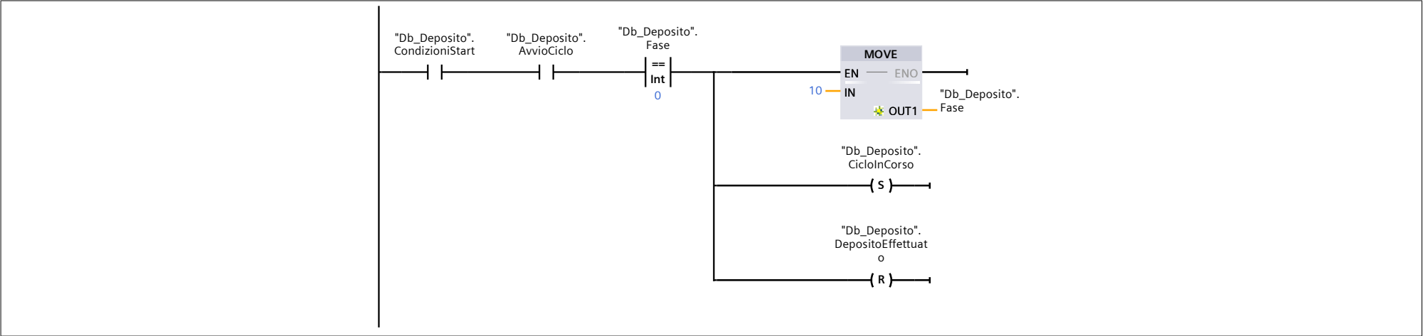
Segmento 10: Fase 10: posizionamento asse z in posizione di deposito
