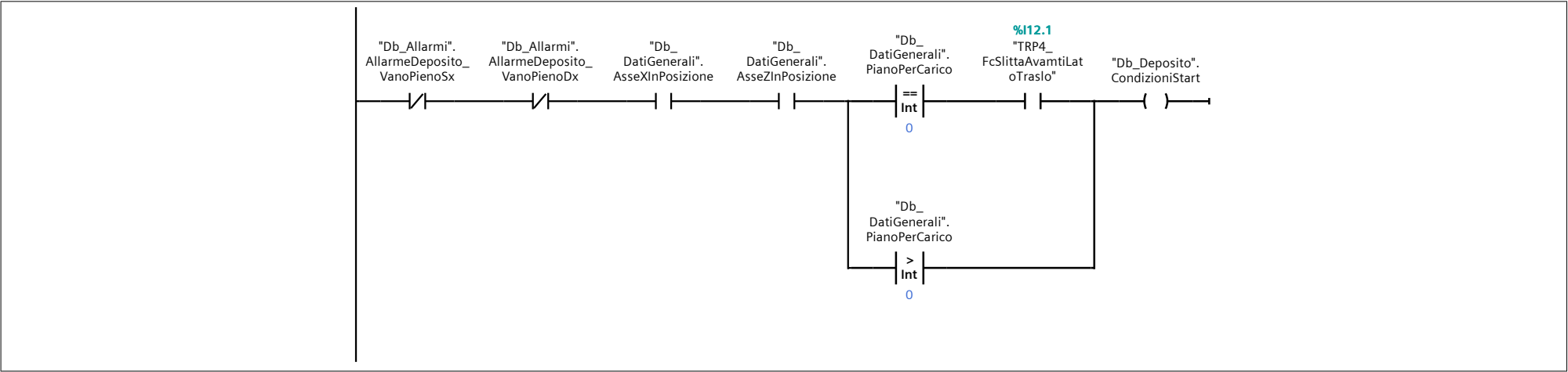
Segmento 9: Fase 0: Home Position; Avvio ciclo di posizionamento
