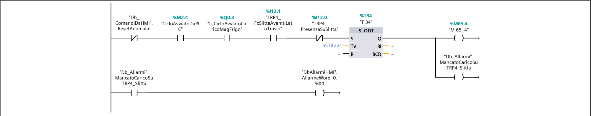
Segmento 6: Time-Out Mancato Scarico su TRP4
