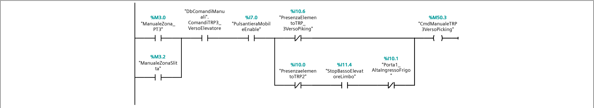
Segmento 9: transito da elevatore a trp2
