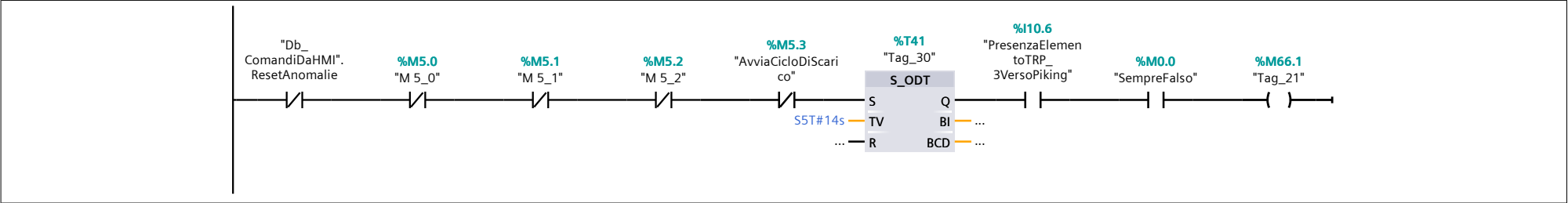
Segmento 11: Time-Out presenza elevat. Piking
