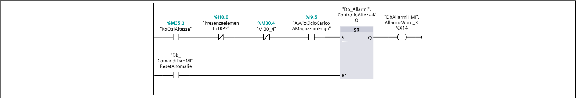
Segmento 66: allarme cesoiamento sx
