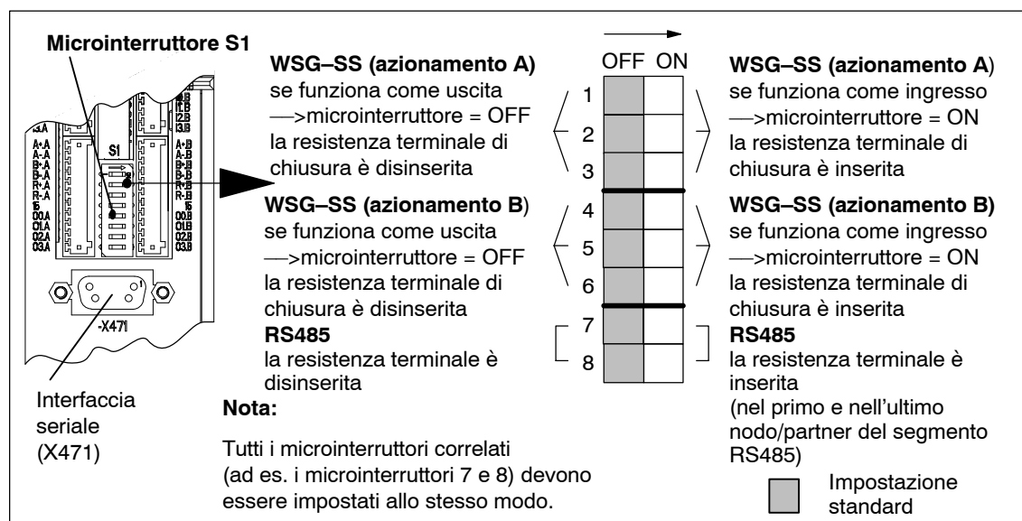
Fig. 1-6 Posto di montaggio e impostazioni del microinterruttore S1
