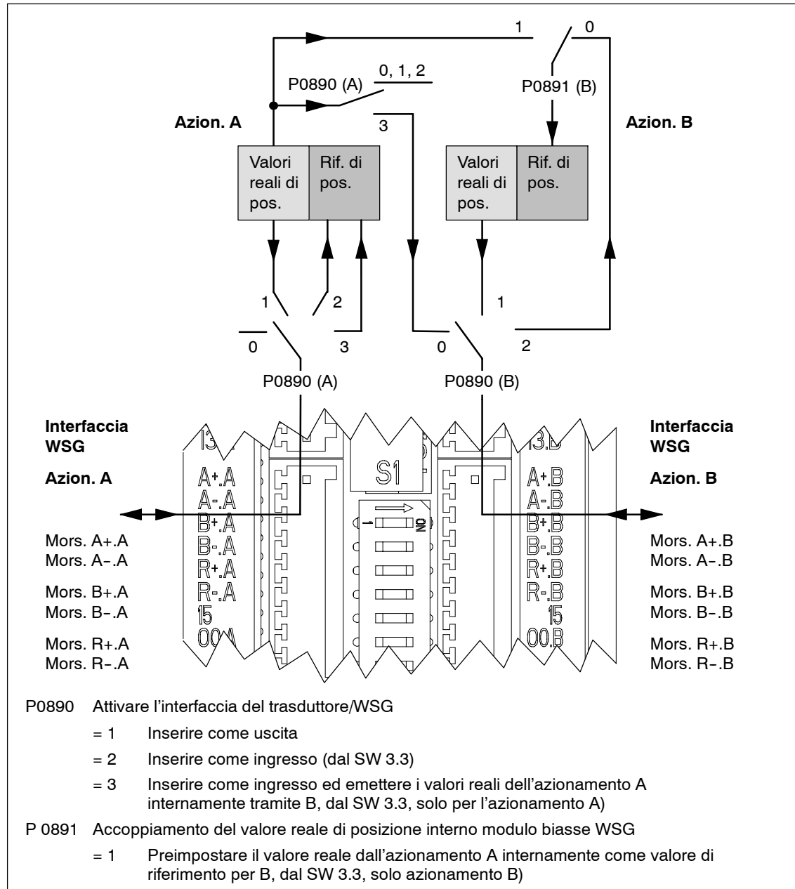
Fig. 6-66 Interfaccia WSG per l'azionamento A e B: parametrizzazione con il P0890 e il P0891
