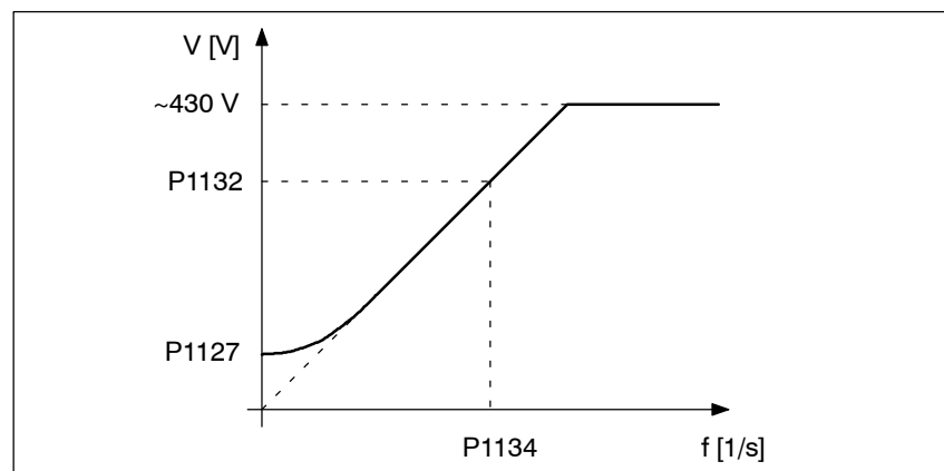
Fig. 7-12 Caratteristica V/f per ARM
