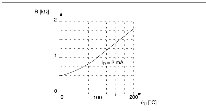
Fig. 4-16 Caratteristica del sensore di temperatura (Temp-F)
