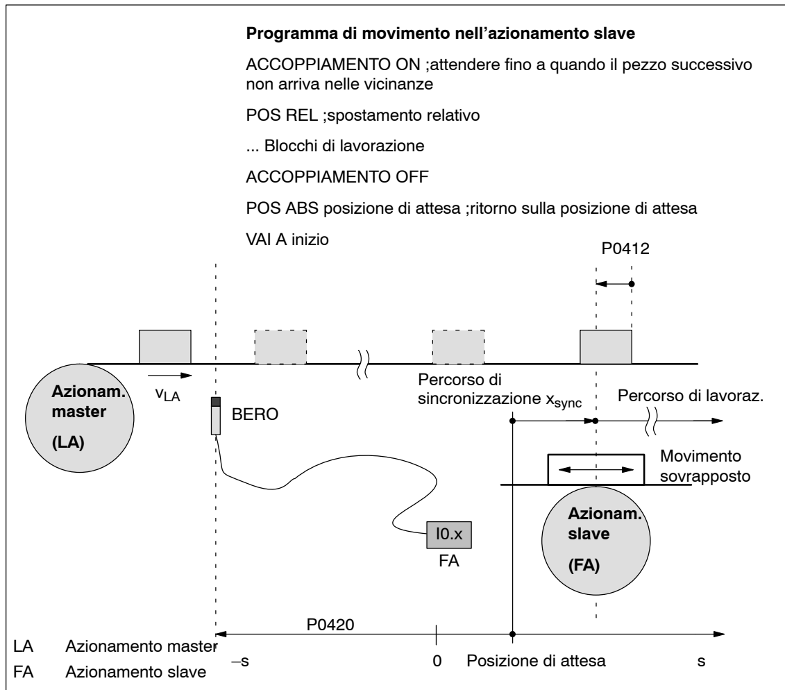
Fig. 6-38 Esempio applicativo: accoppiamento tramite morsetto d'ingresso con funzione Queue
