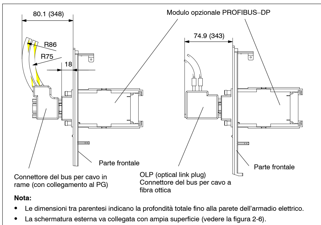
Fig. 2-10 Profondità di montaggio del connettore del bus con il modulo opzionale PROFIBUS-DP
