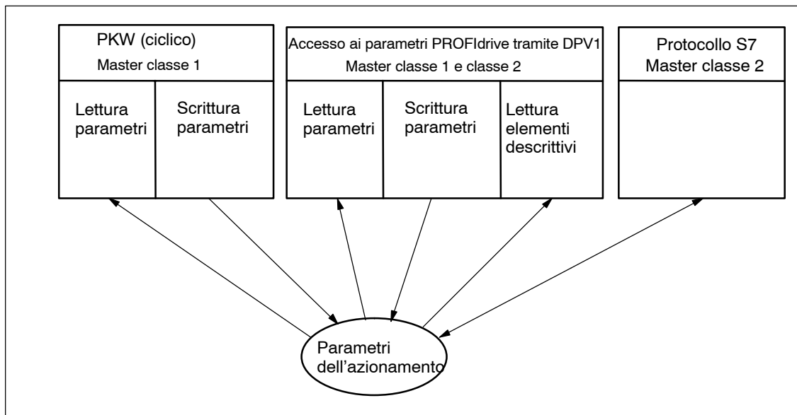
Fig. 5-5 Panoramica dell'accesso ai parametri PROFIdrive
