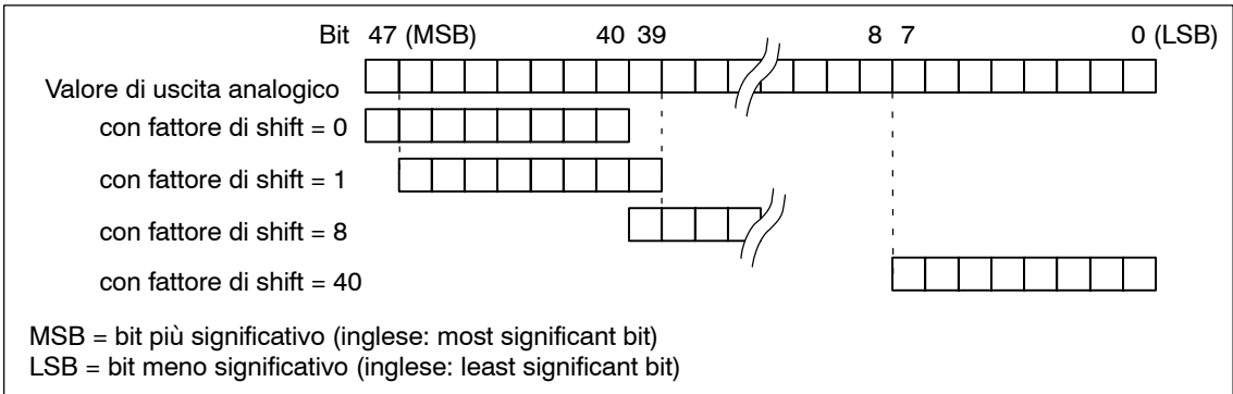
Fig. 6-63 Fattore di shift per l'uscita analogica dei segnali a 48 bit
