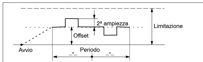
Fig. 7-6 Forma a "gradini" con ampiezza = 0 e offset > ampiezza 2
