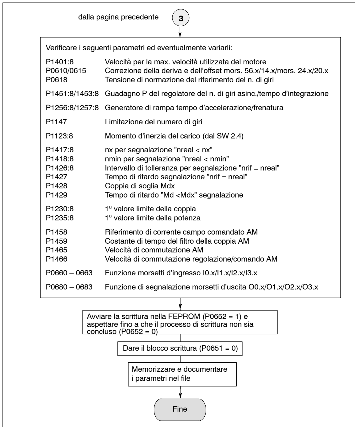
Fig. 4-9 Messa in servizio dei motori asincroni senza trasduttore (parte 3)
