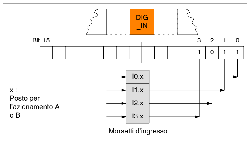
Fig. 5-12 Parola di stato DIG_IN (dal SW 3.1)
