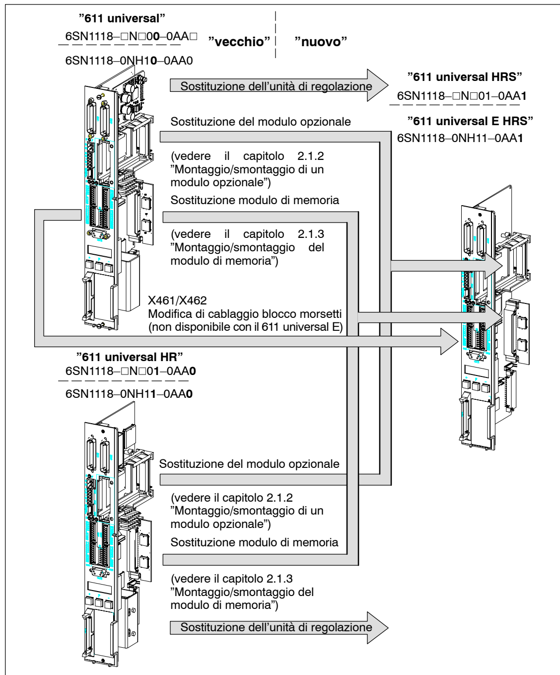
Fig. 2-4 Sostituzione di una unità di regolazione difettosa con una nuova di tipo HRS
