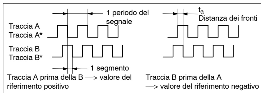
Fig. 6-72 Valore del riferimento di posizione con il segnale in quadratura (P0894 = 0)
