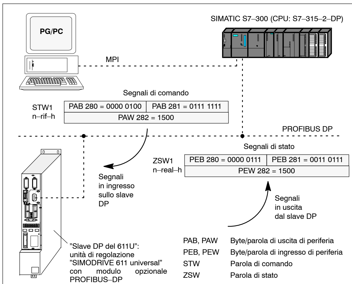
Fig. 5-19 Esempio: muovere l'azionamento via PROFIBUS
