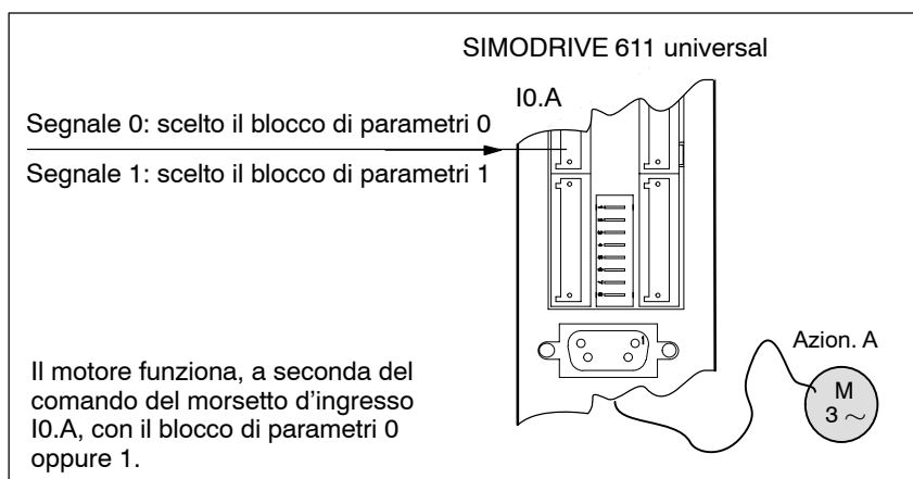
Fig. 6-79 Esempio: commutazione del blocco di parametri
