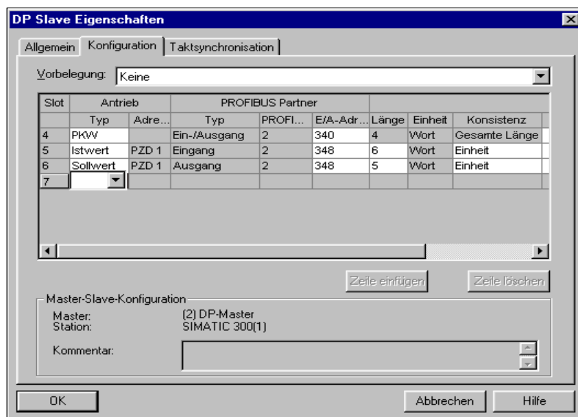
Fig. 6-44 Esempio di configurazione per azionamento master con progettazione S7
