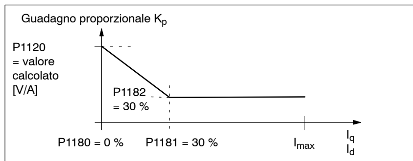
Fig. 4-10 Preimpostazione dell'adattamento del regolatore di corrente con i motori 1FE1
