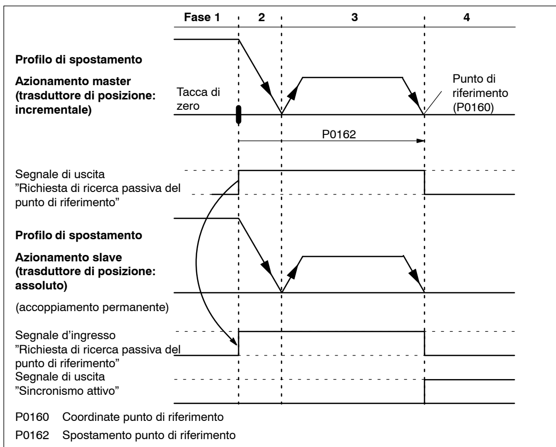
Fig. 6-41 Sequenza nella ricerca del punto di riferimento passiva (azionamento master con trasduttore incrementale e azionamento slave con trasduttore assoluto)
