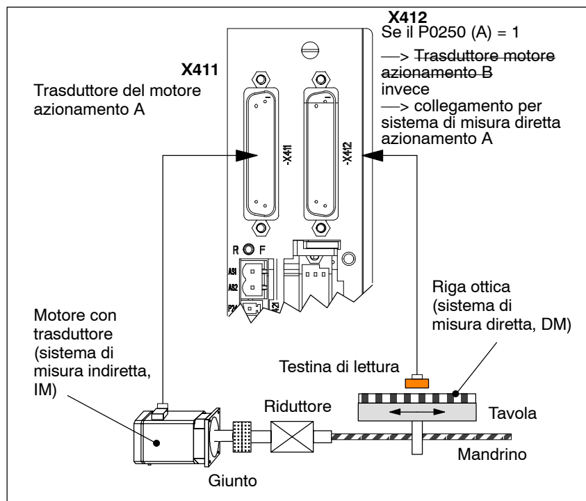
Fig. 4-22 Sistema di misura indiretta e diretta per l'azionamento A
