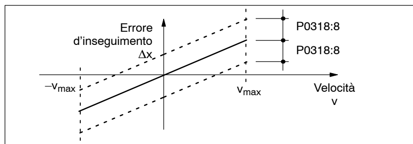
Fig. 6-18 Errore di inseguimento
