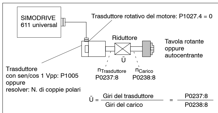
Fig. 6-13 Asse rotante con trasduttore rotativo del motore
