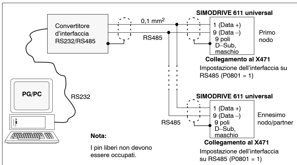
Fig. 2-14 Cavo di collegamento RS485: PG/PC ↔ convertitore d'interfaccia RS232/RS485 ↔ SIMODRIVE 611 universal
