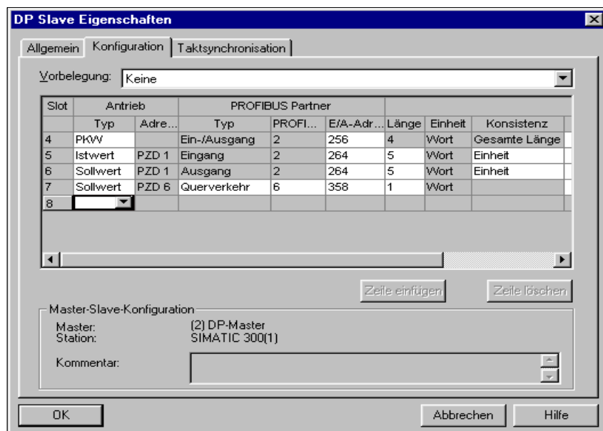
Fig. 6-45 Esempio di configurazione per azionamento slave con progettazione S7
