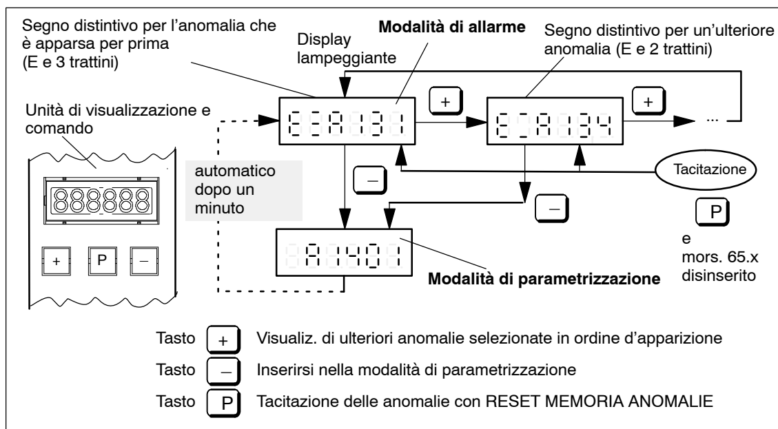
Fig. 7-2 Come comandare se sono intervenute diverse anomalie
