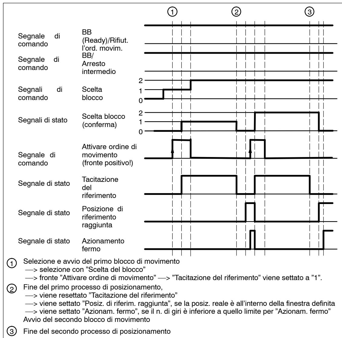
Fig. 6-27 Avvio sequenziale di blocchi singoli
