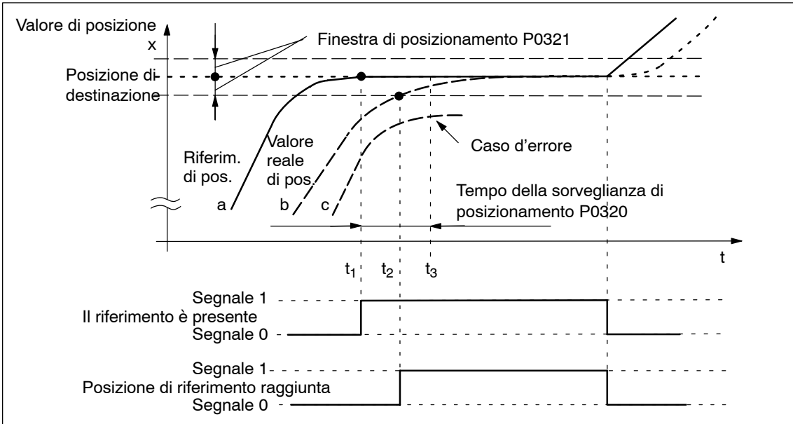
Fig. 6-20 Sorveglianza di posizionamento
