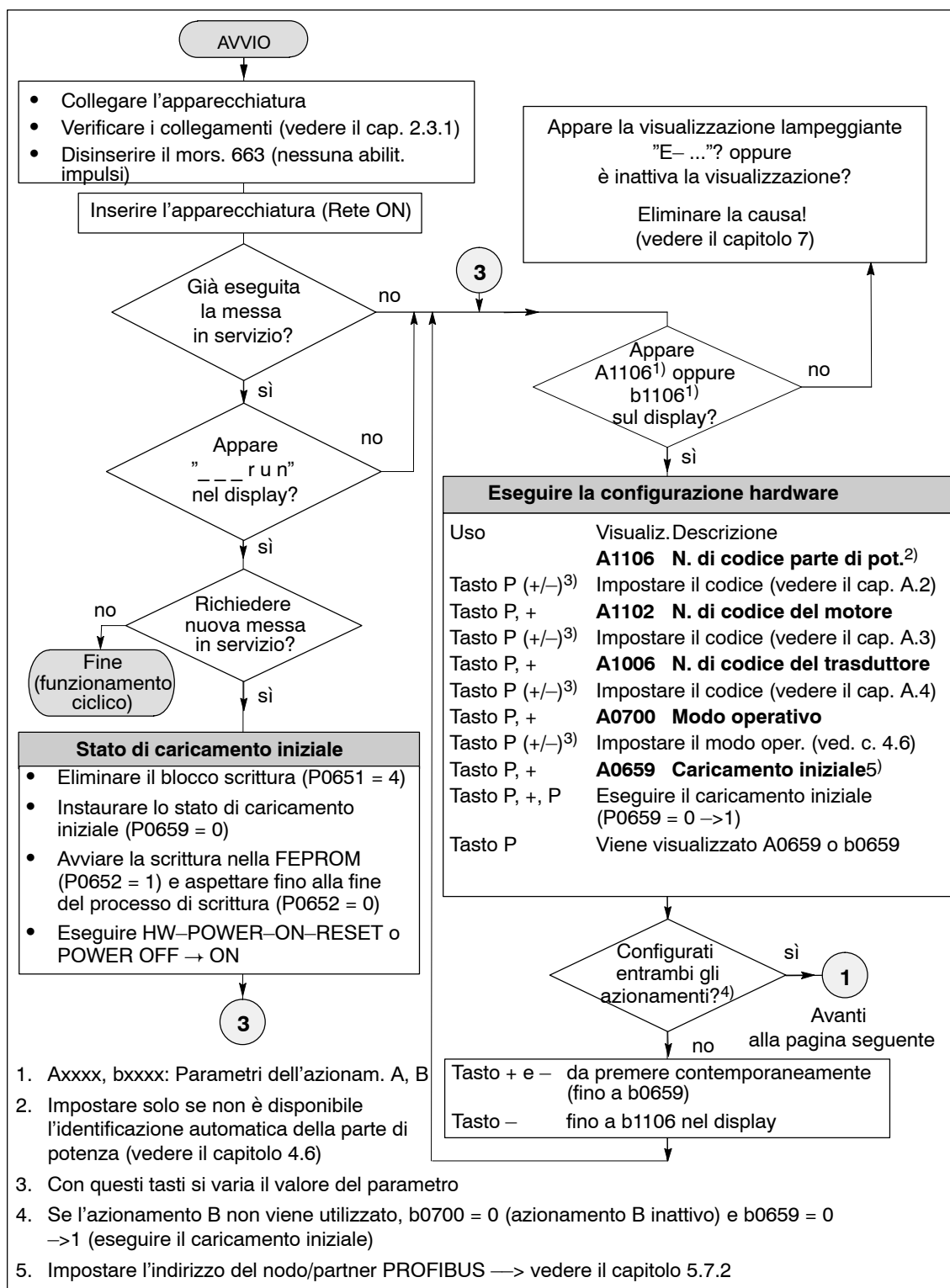
Fig. 4-3 Messa in servizio con l'unità di visualizzazione e comando (parte 1 di 3)
