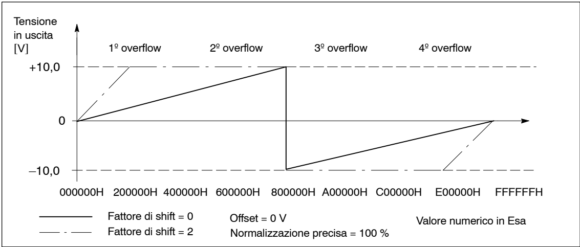
Fig. 6-64 Tensione d'uscita analogica con la protezione alla saturazione (P0631/P0638 = 1)
