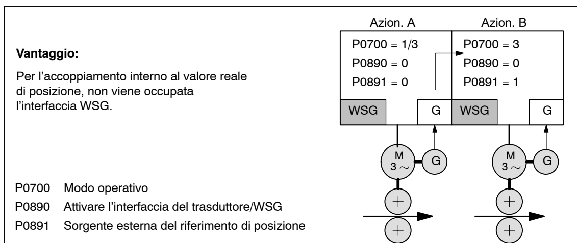
Fig. 6-32 Accoppiamento interno al valore reale di posizione
