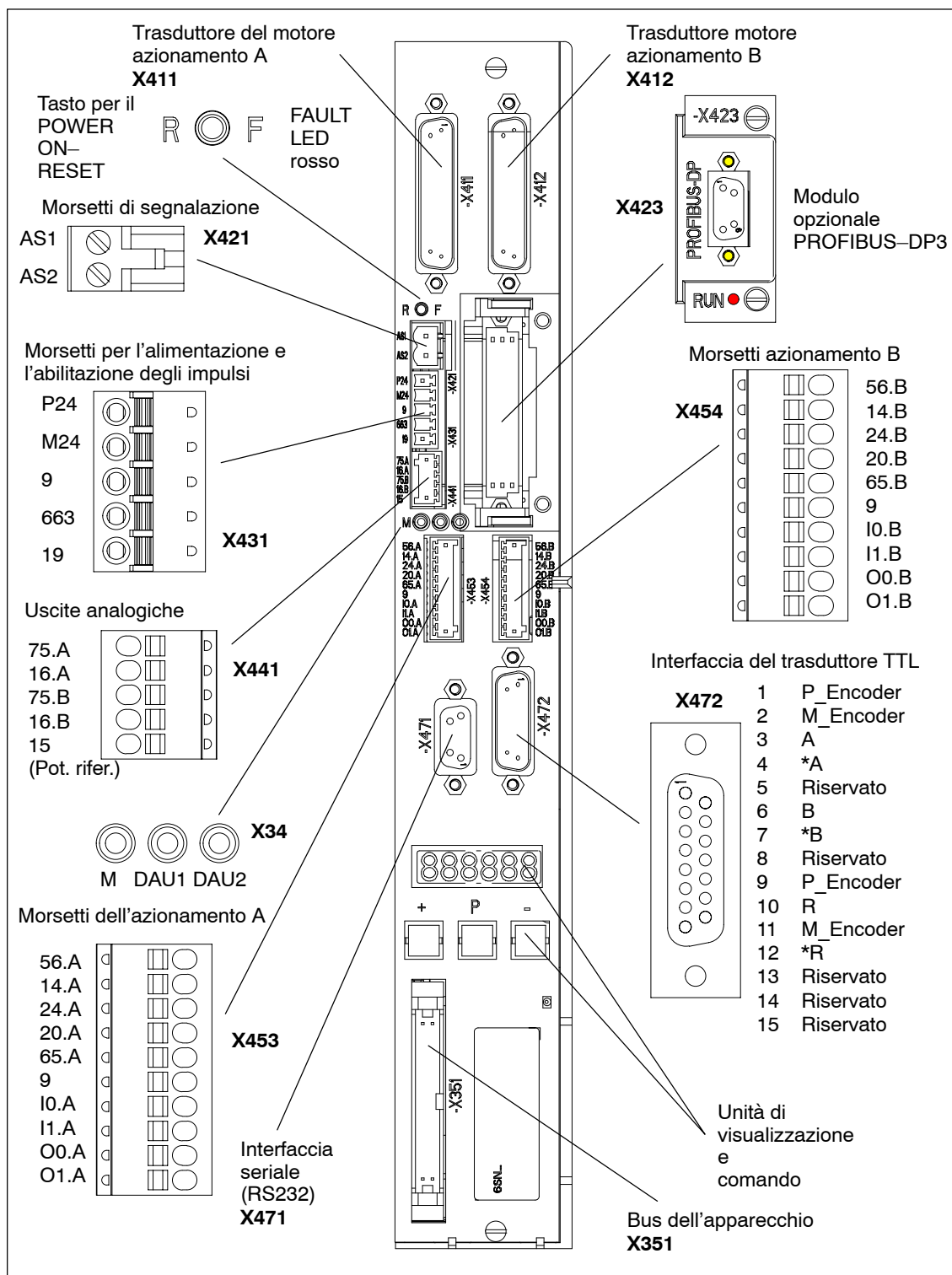
Fig. 1-10 Elementi presenti sulla parte frontale del "SIMODRIVE 611 universal E"
