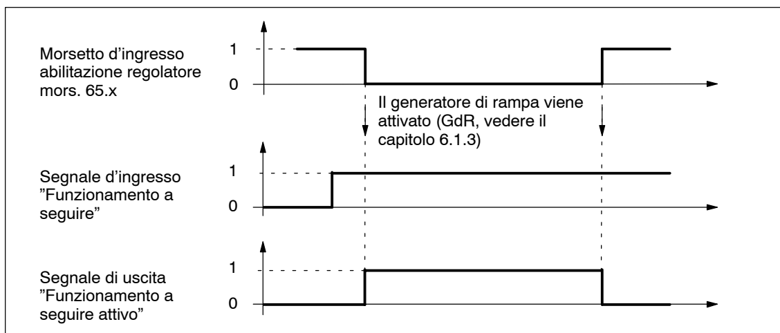
Fig. 6-21 Andamento temporale con il funzionamento a seguire
