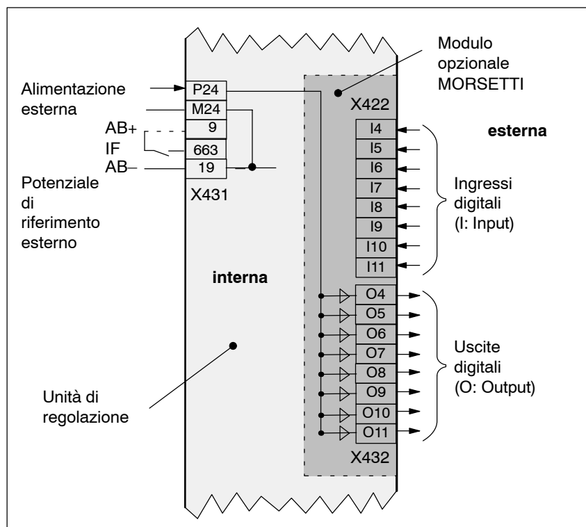
Fig. 2-8 Schema di collegamento del modulo opzionale MORSETTI
