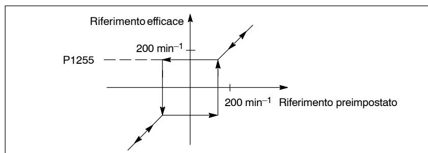
Fig. 6-8 Modo d'azione numero di giri minimo
