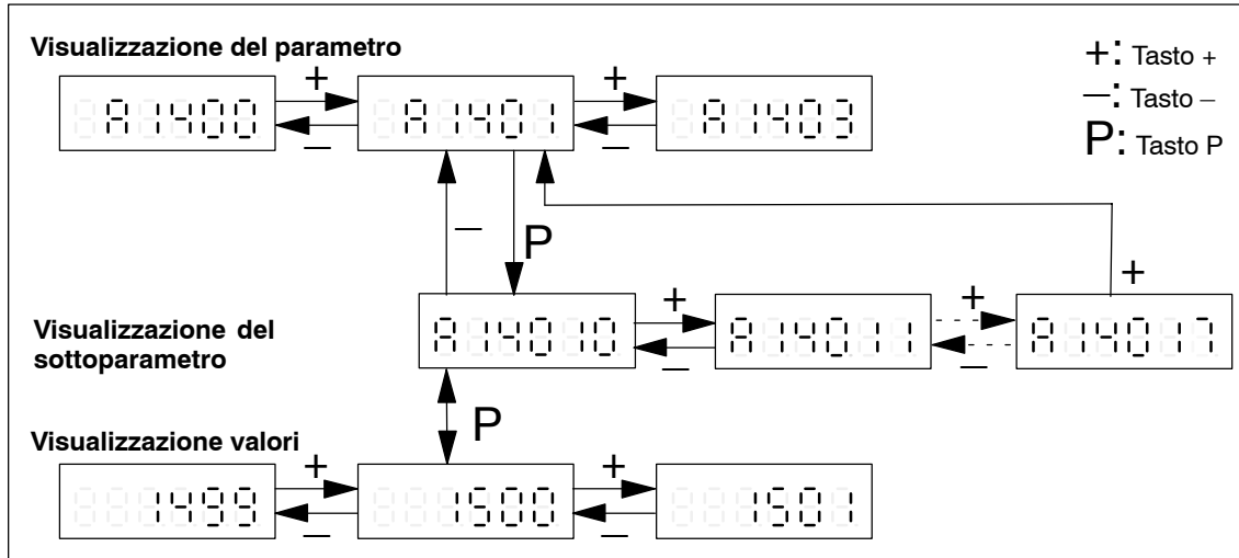
Fig. 3-3 Comando in caso di parametri con sottoparametri e visualizzazione dei valori max. 6 posizioni
