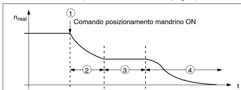
Fig. 6-86 Esempio di posizionamento mandrino
