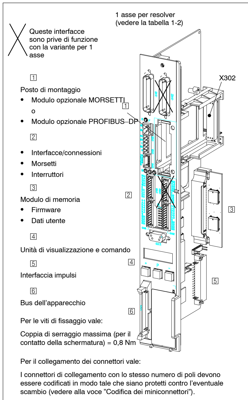
Fig. 1-4 Unità di regolazione per 1 asse
