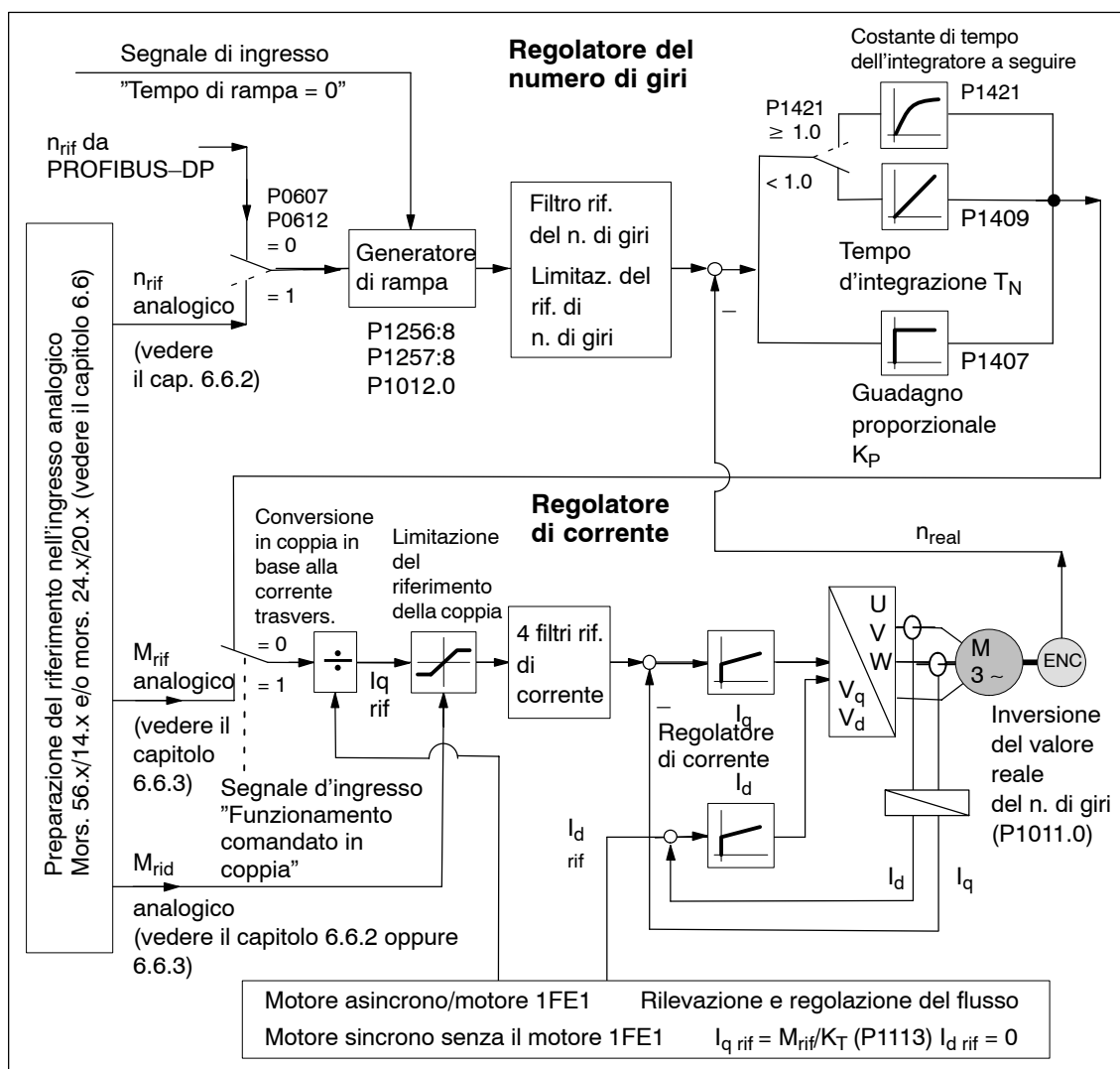
Fig. 6-4 Regolatore di corrente e del numero di giri
