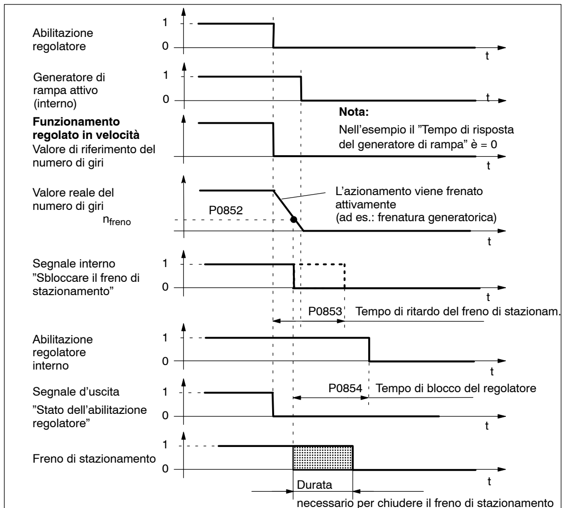
Fig. 6-76 Chiudere il freno: comportamento disattivando l' "Abilitazione regolatore"
