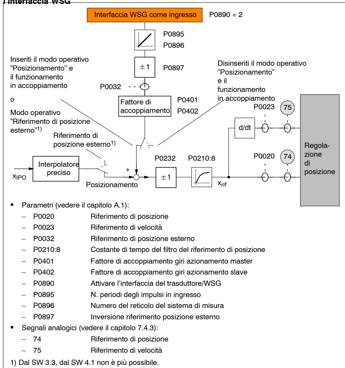
Fig. 6-71 Riferimento di posizione incrementale con l'interfaccia WSG
