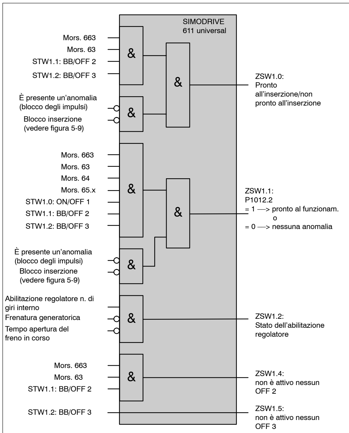
Fig. 5-8 Stati dipendenti dai morsetti HW e dai segnali PROFIBUS
