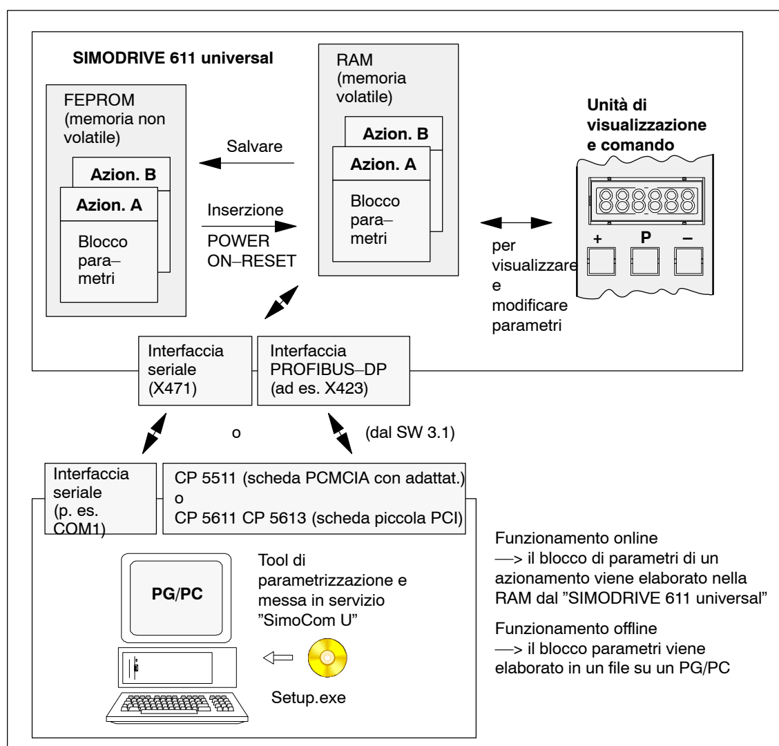
Fig. 3-1 Panoramica per la parametrizzazione
