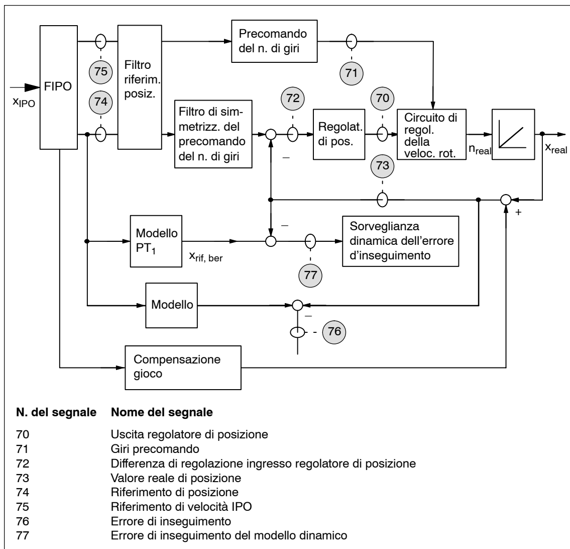
Fig. 6-61 Segnali analogici per il anello di regolazione della posizione
