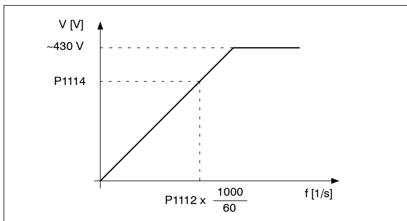
Fig. 7-13 Caratteristica V/f per SRM
