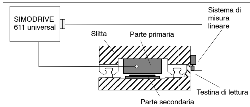
Fig. 6-12 Asse lineare con trasduttore lineare del motore
