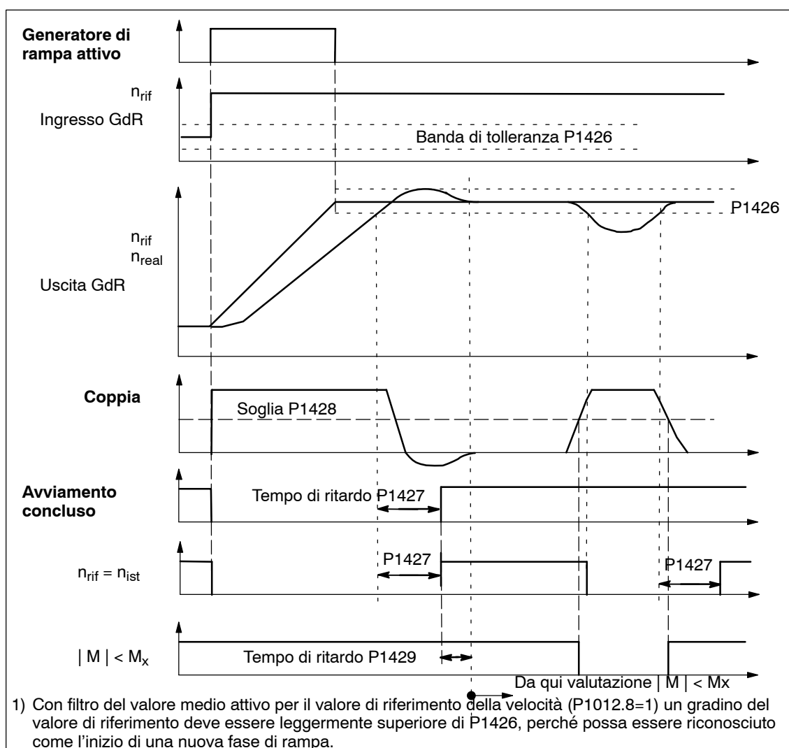
Fig. 6-5 Andamento del segnale del generatore di rampa
