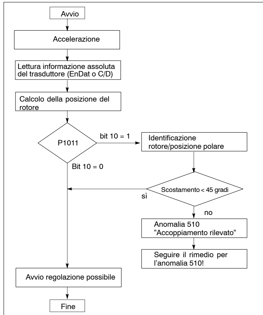
Fig. 6-92 Sorveglianza della plausibilità con trasduttore assoluto
