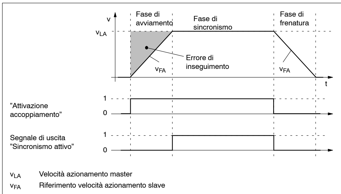
Fig. 6-35 Sincronismo di velocità (P0410 = 1 o 3)
