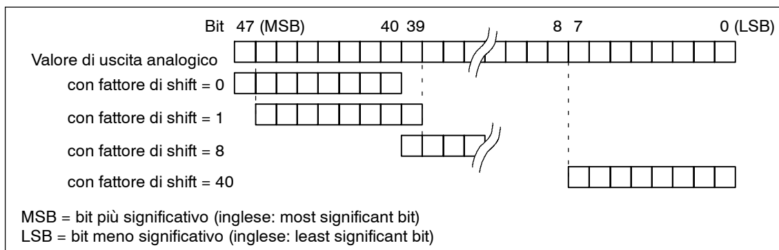
Fig. 7-9 Fattore di shift per l'uscita analogica dei segnali a 48 bit
