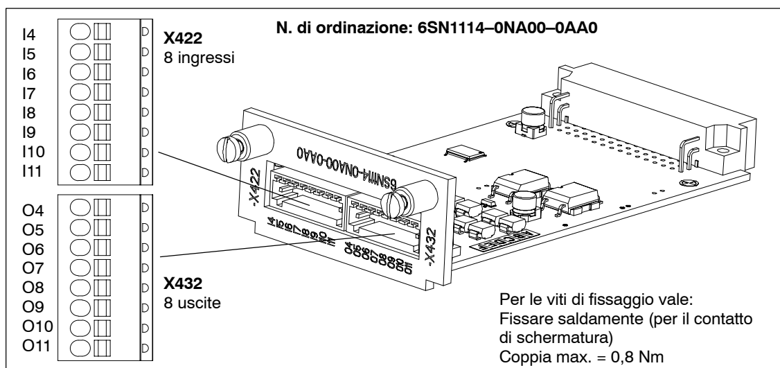
Fig. 1-7 Modulo opzionale MORSETTI
