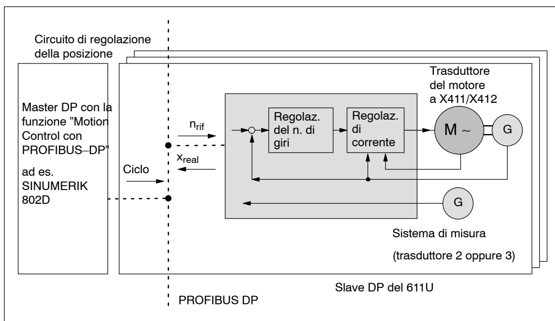
Fig. 5-25 Panoramica del "Motion Control con PROFIBUS-DP": esempio con master DP e 3 slave DP
