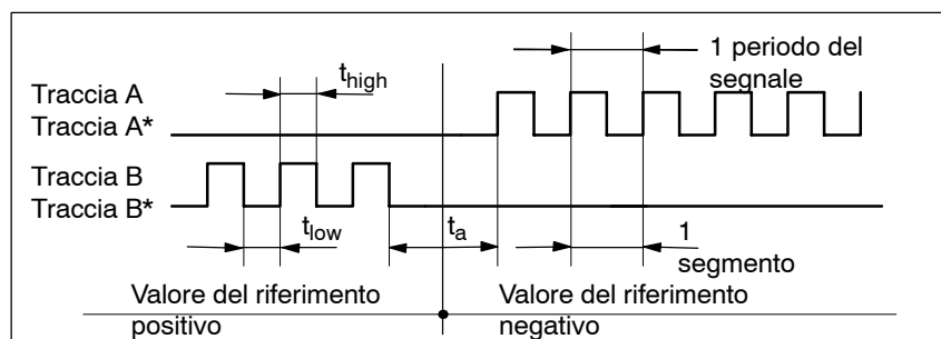
Fig. 6-74 Valore del riferimento di posizione con il segnale avanti/indietro (P0894 = 2)
