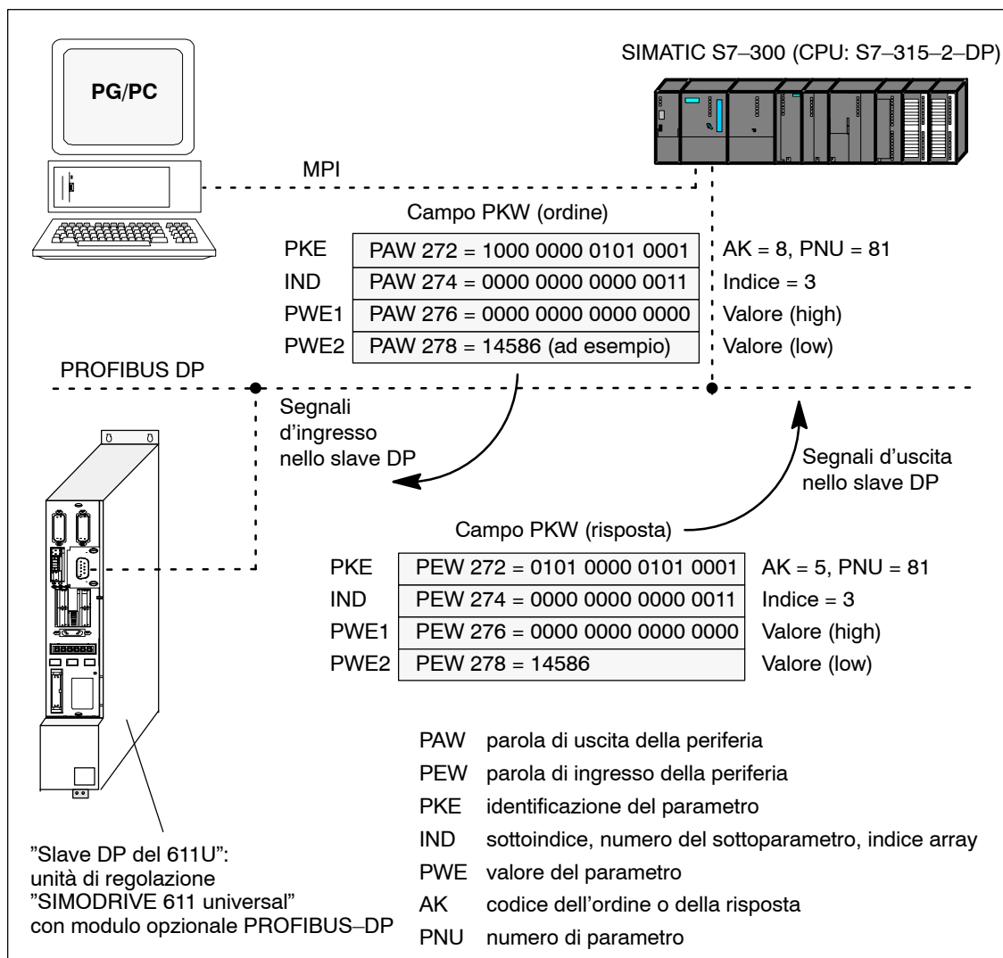
Fig. 5-21 Esempio: scrittura dei parametri con PROFIBUS
