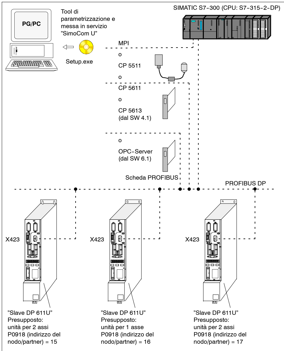
Fig. 3-11 SimoCom U con PROFIBUS (esempio con 3 unità di regolazione)
