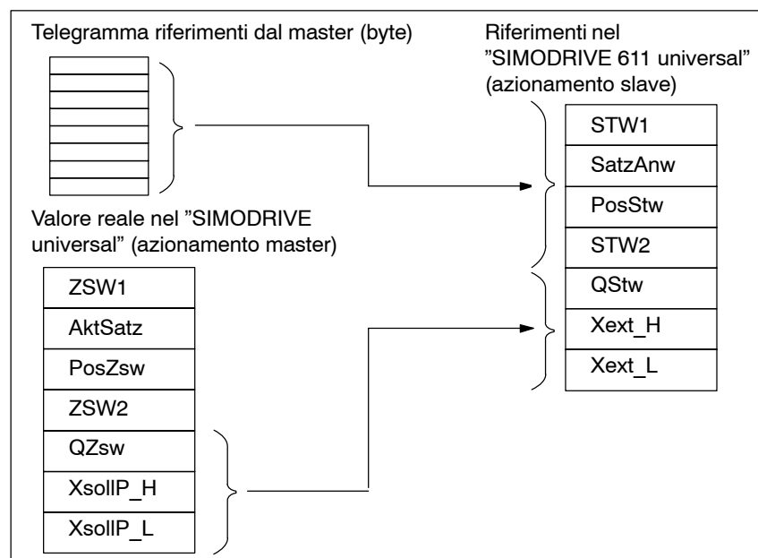
Fig. 5-33 Esempio di attribuzione dei dati di processo per una applicazione con funzionamento sincrono
