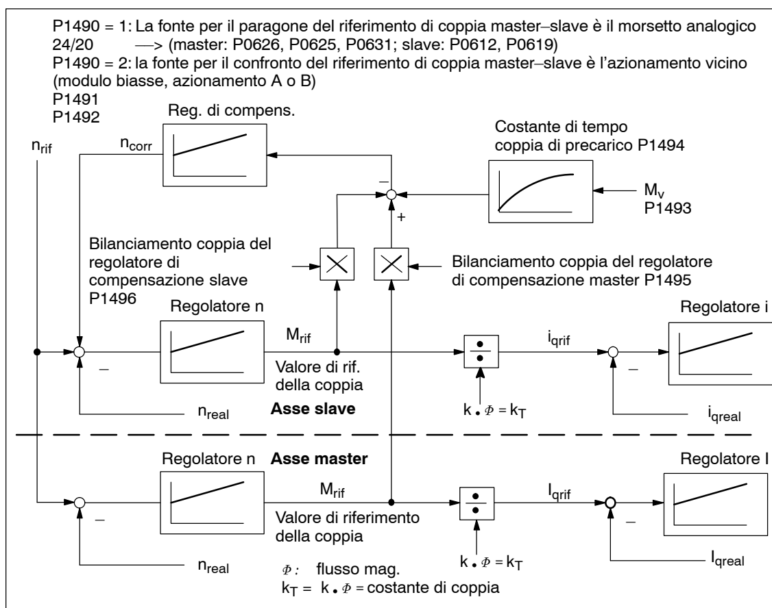
Fig. 6-48 Struttura del regolatore di parità
