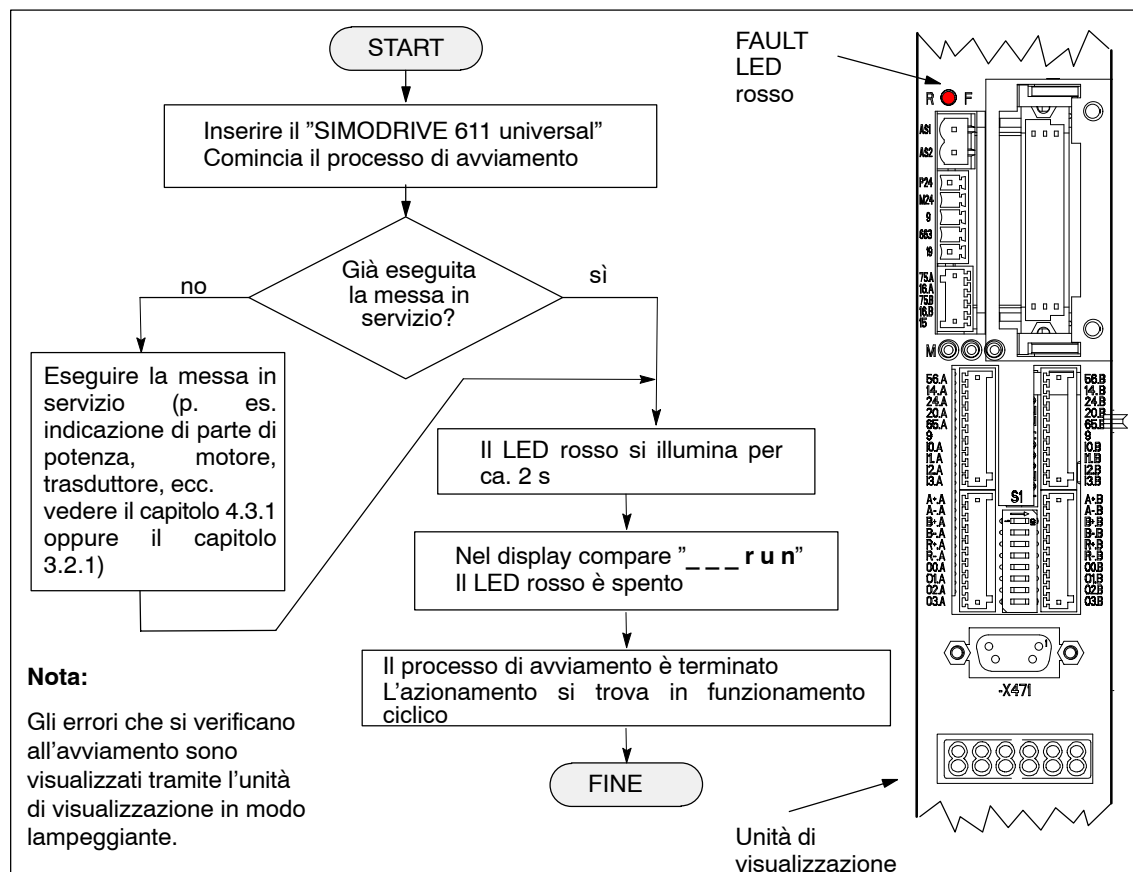
Fig. 4-1 Avviamento del "SIMODRIVE 611 universal"
