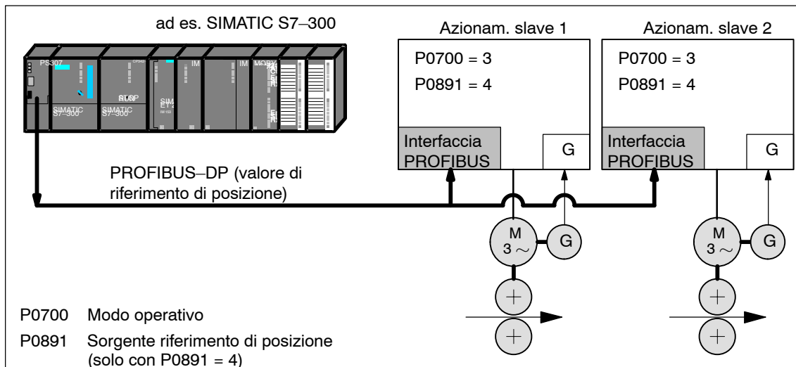
Fig. 6-33 Master DP, ad es. SIMATIC S7-300 come sorgente per il "Riferimento esterno della posizione"
