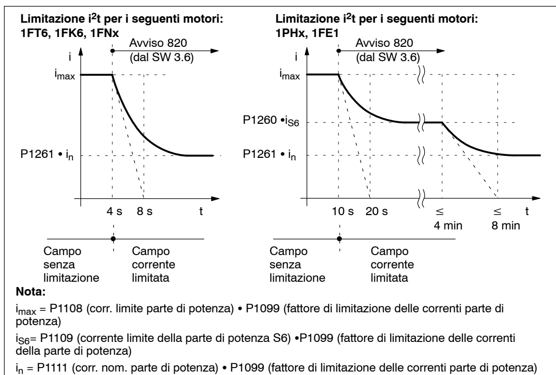
Fig. A-2 Comportamento con il funzionamento continuativo al limite di corrente
