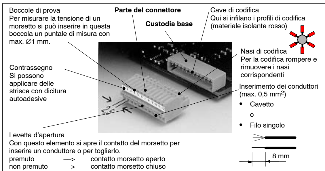
Fig. 2-5 Connettore di collegamento nella forma compatta (miniconnettore)
