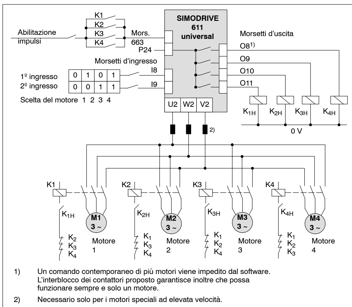
Fig. 6-82 Collegamento proposto: commutazione di 4 motori ognuno con un blocco di dati del motore
