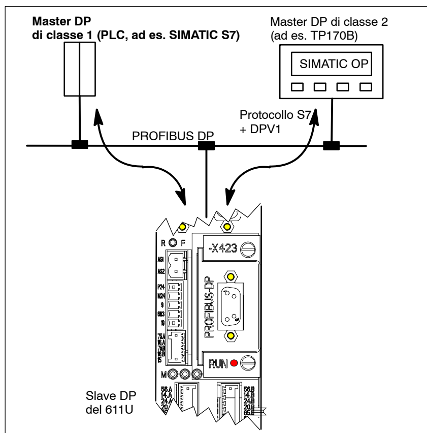
Fig. 5-6 Comunicazione SIMATIC OP – "SIMODRIVE 611 universal"
