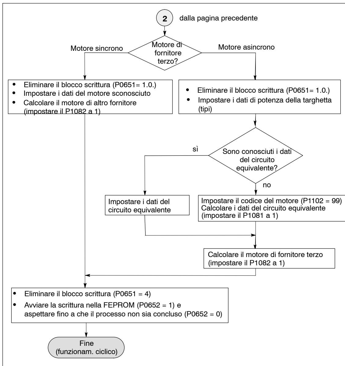
Fig. 4-5 Messa in servizio con l'unità di visualizzazione e comando (parte 3 di 3)
