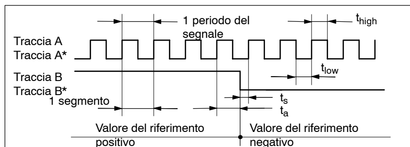
Fig. 6-73 Valore del riferimento di posizione con il segnale impulso/direzione (P0894 = 1)
