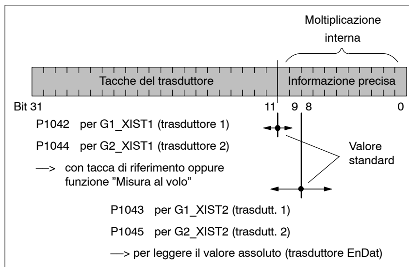
Fig. 5-18 Suddivisione e impostazioni nel Gx\_XIST2
