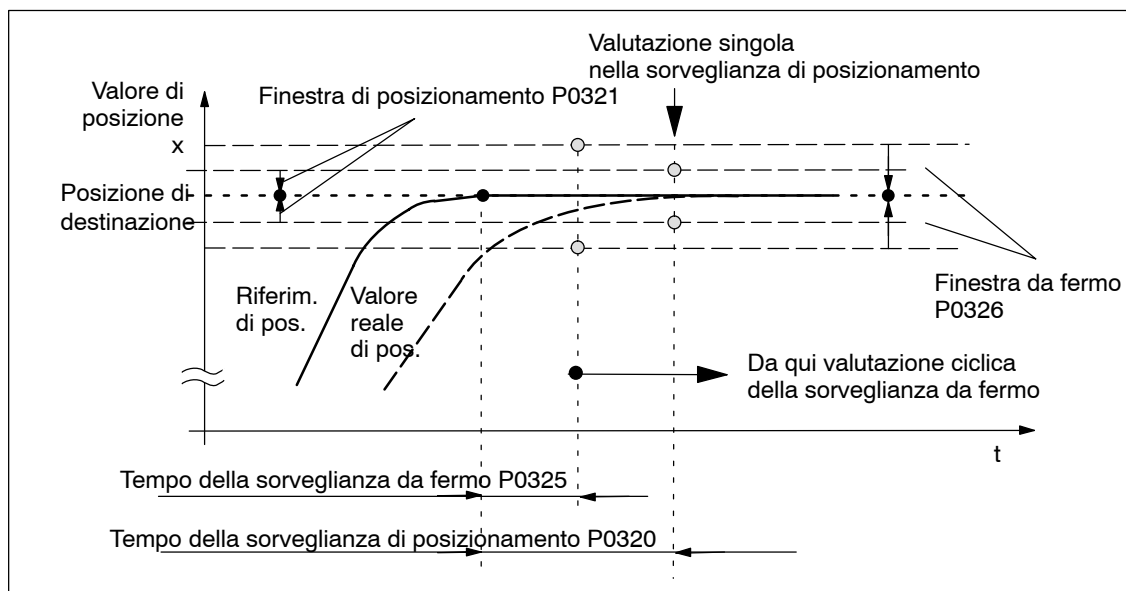
Fig. 6-19 Sorveglianza da fermo e di posizionamento
