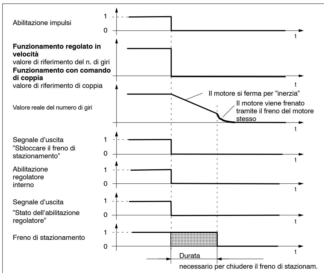
Fig. 6-77 Chiudere il freno: comportamento disabilitando l'"Abilitazione impulsi"
