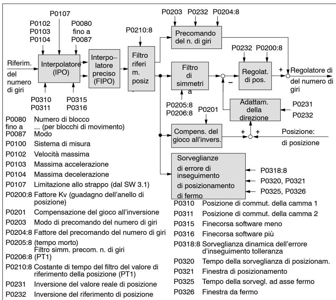
Fig. 6-14 Componenti per la regolazione della posizione
