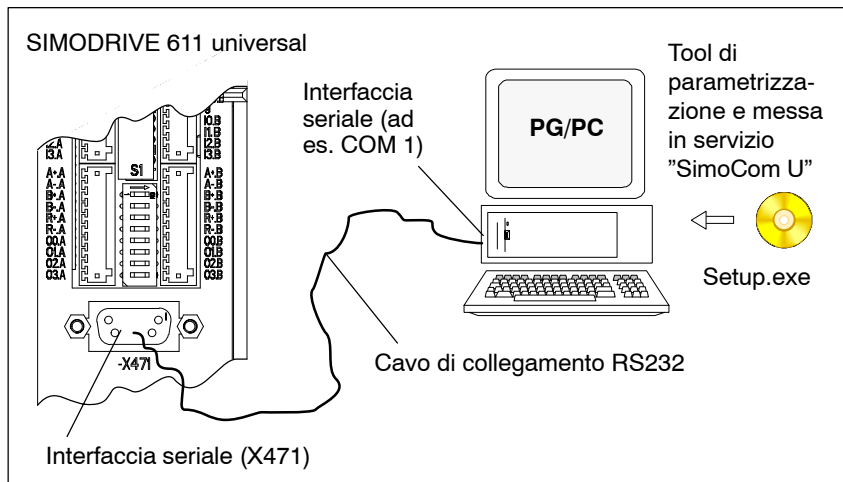
Fig. 3-9 Comunicazione tramite RS232
