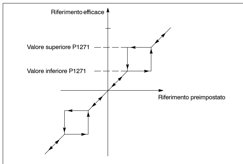
Fig. 6-9 Modo d'azione esclusione campo numero di giri
