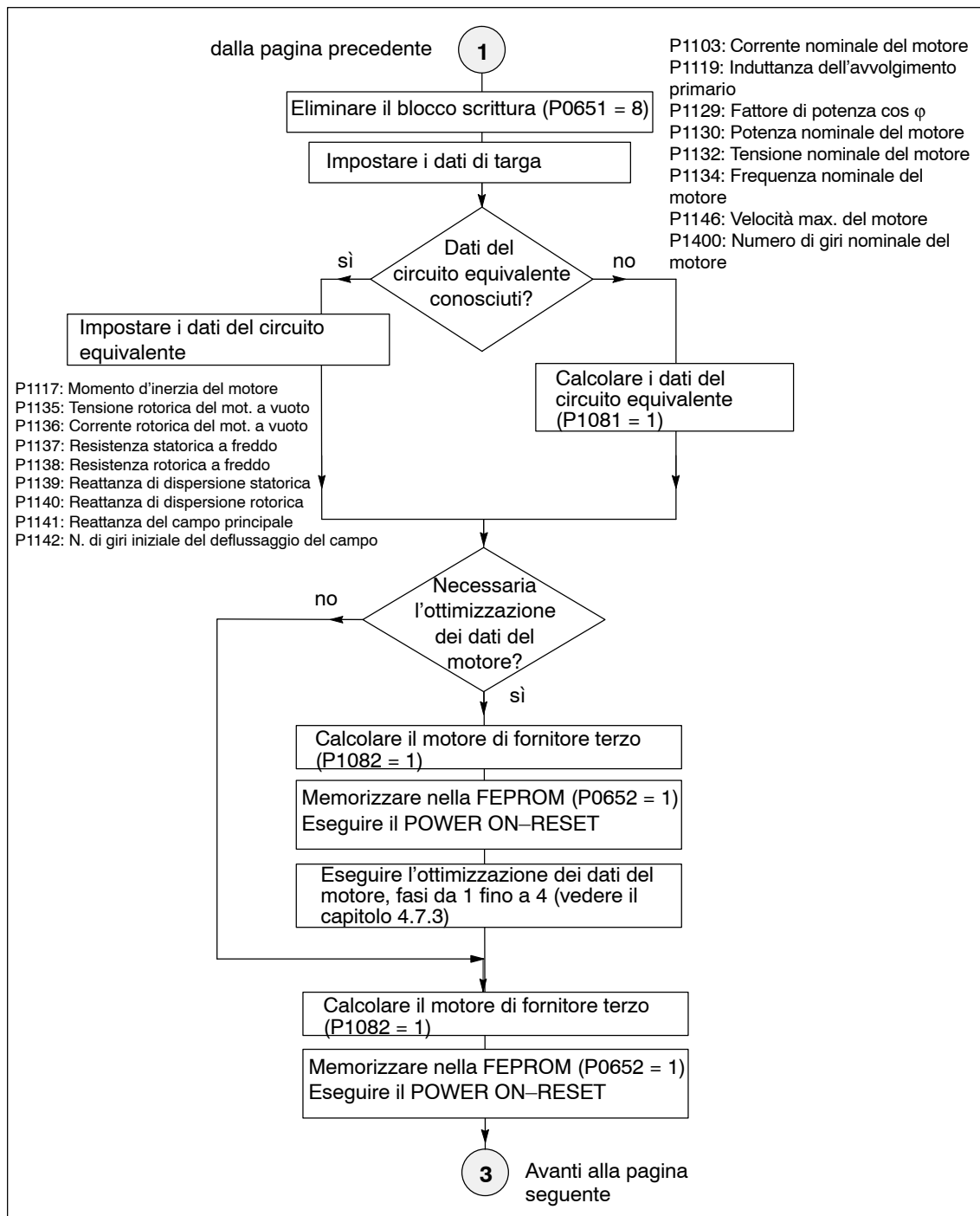
Fig. 4-8 Messa in servizio dei motori asincroni senza trasduttore (parte 2)
