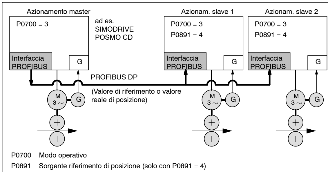
Fig. 6-34 Accoppiamento in sincronismo di più slave DP
