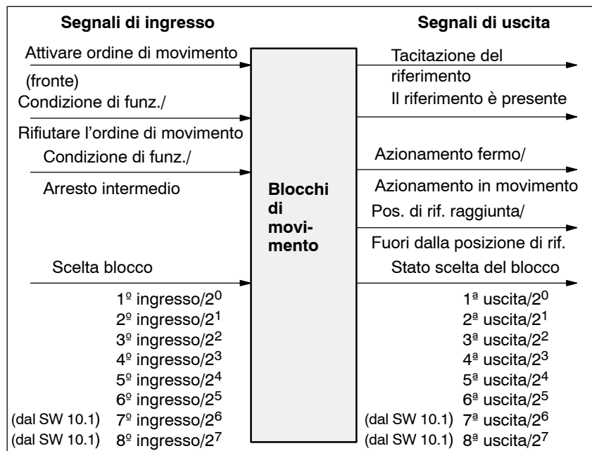
Fig. 6-26 Segnali d'ingresso/di uscita per i blocchi di movimento
