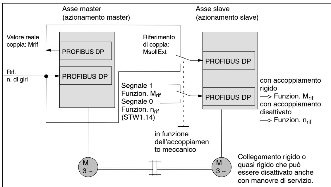
Fig. 6-43 Esempio: accoppiamento di due azionamenti con master/slave via PROFIBUS-DP
