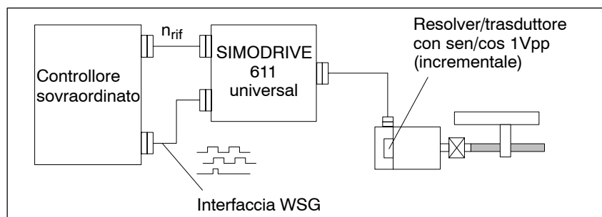
Fig. 6-2 Posizionamento per mezzo di un controllore sovraordinato, formazione del valore reale di posizione tramite trasduttore angolare (WSG)
