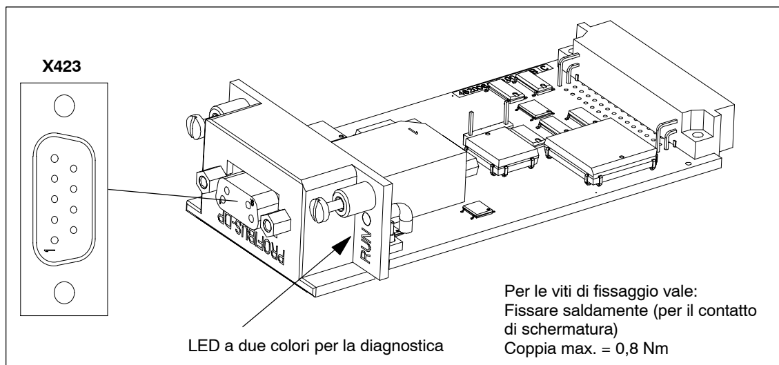
Fig. 1-8 Modulo opzionale PROFIBUS-DP
