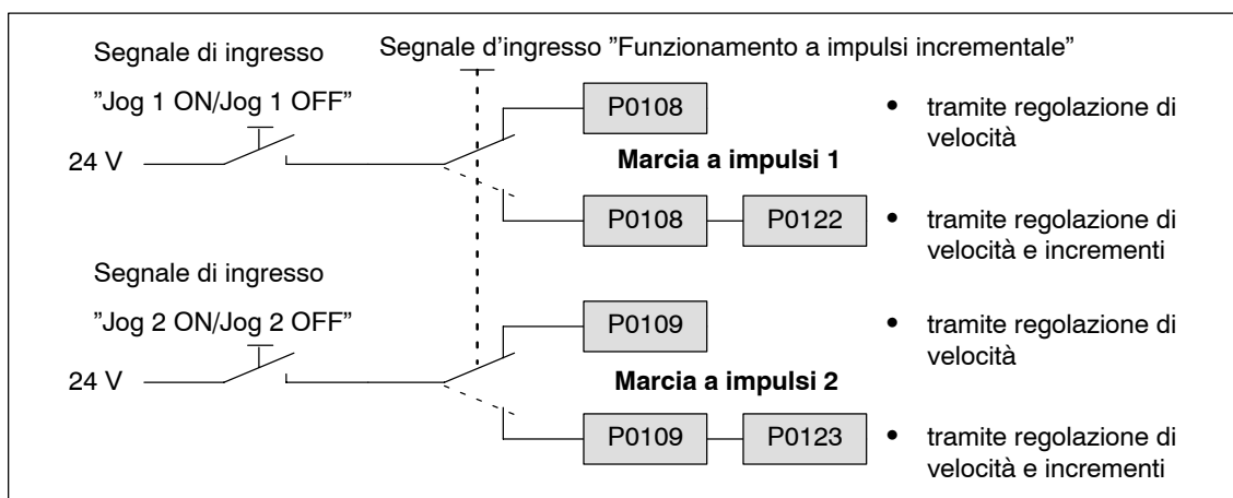
Fig. 6-24 Funzionamento a impulsi: tramite regolazione di velocità o incrementale
