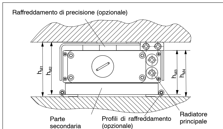
Fig. 4-15 Valori di controllo per il montaggio del motore
