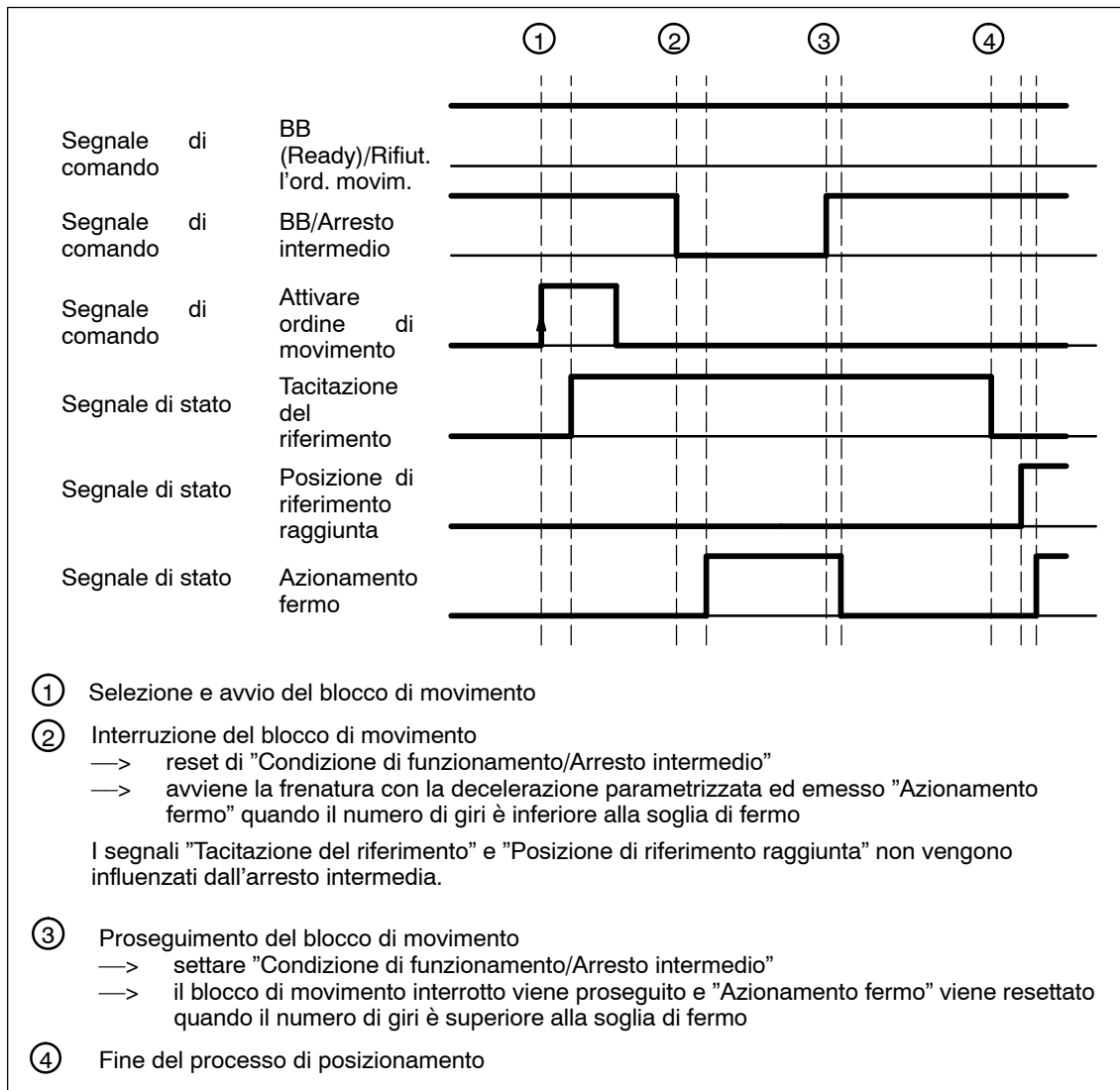
Fig. 6-28 Comportamento con la sosta intermedia di un blocco di movimento
