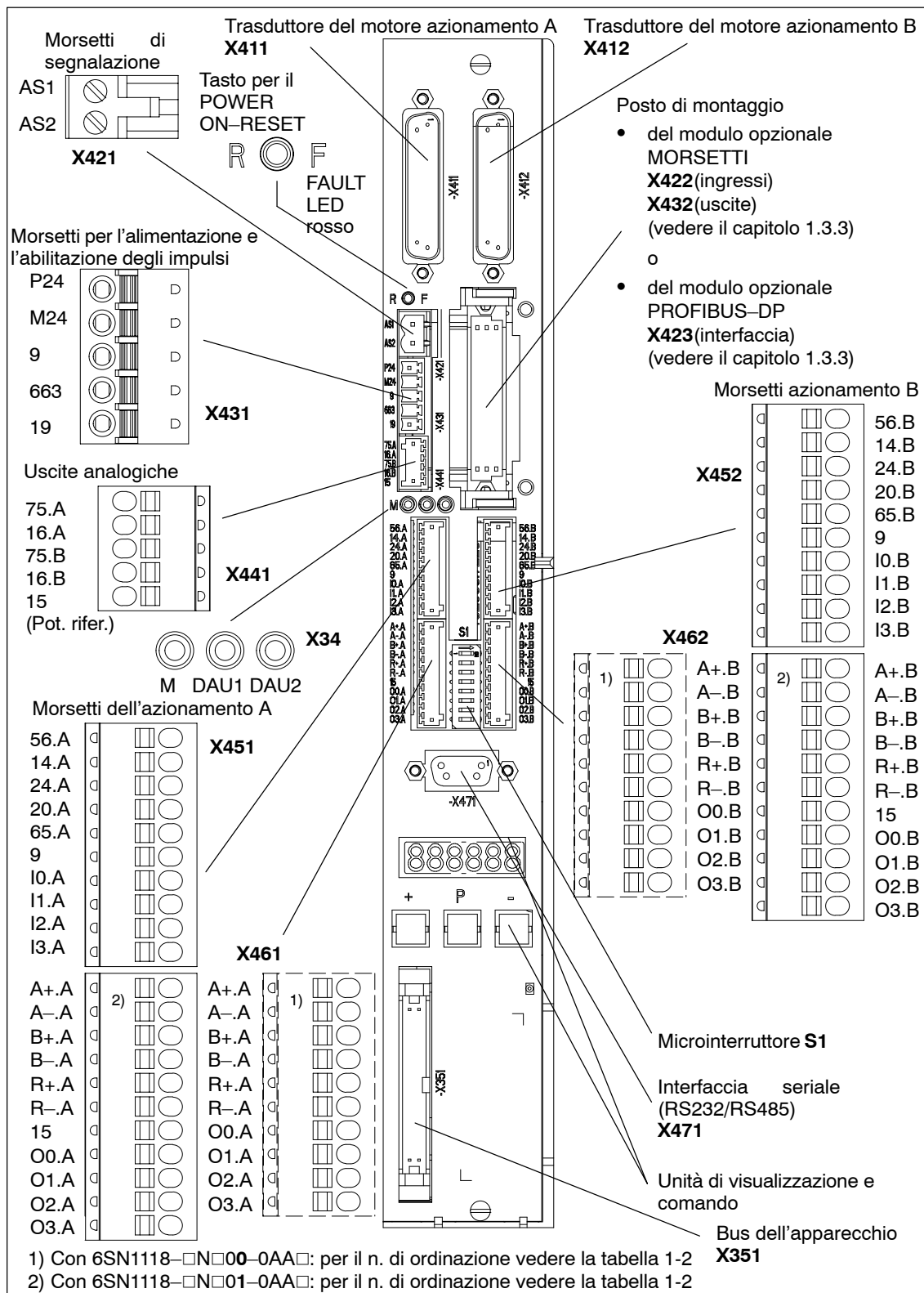
Fig. 1-5 Elementi posti sulla parte frontale (tolta la copertura, nessun modulo opzionale installato)
