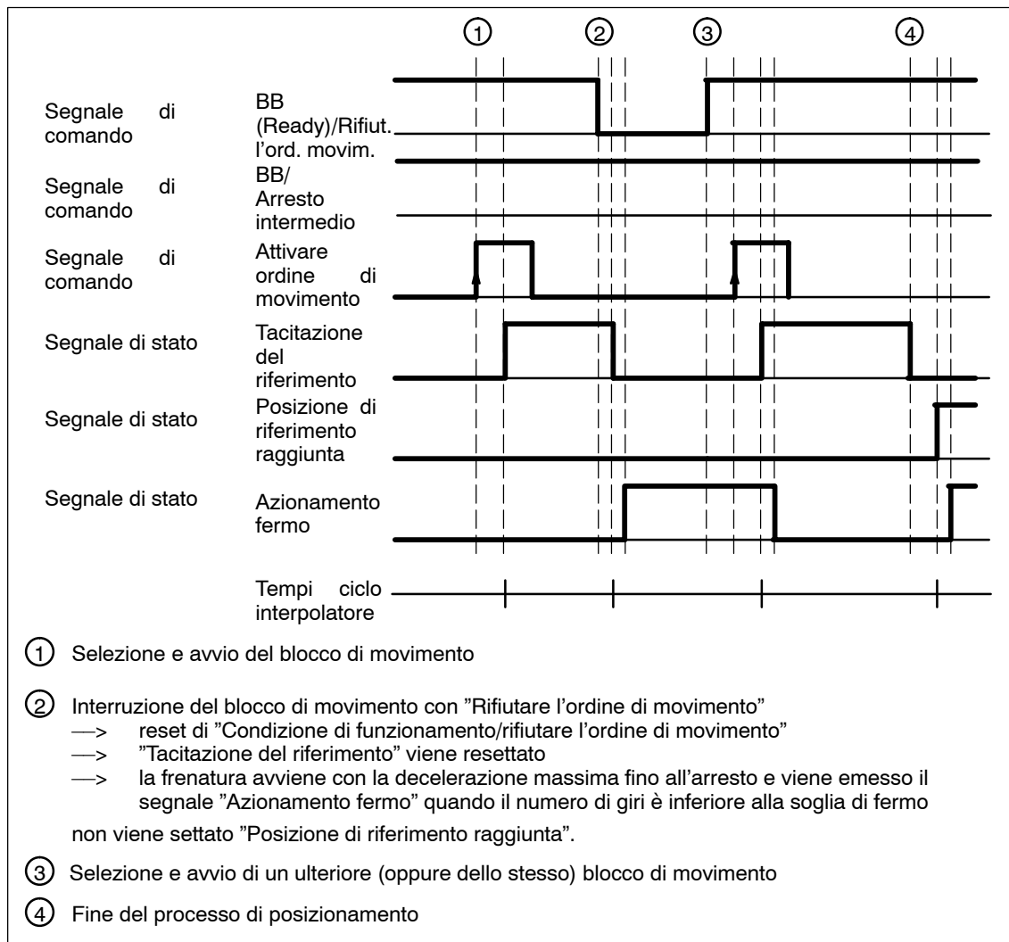
Fig. 6-29 Comportamento con interruzione di un blocco di movimento
