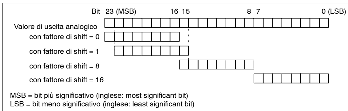
Fig. 7-8 Fattore di shift per l'uscita analogica dei segnali a 24 bit
