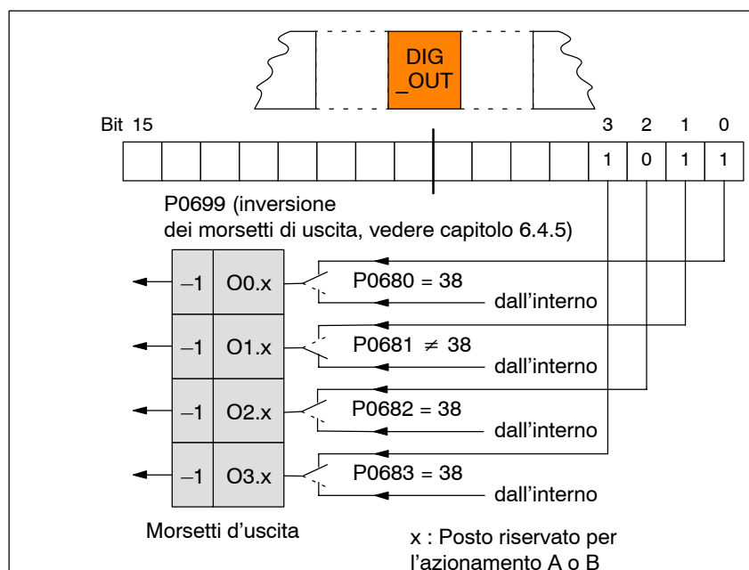
Fig. 5-11 Parola di comando DIG_OUT (dal SW 3.1)
