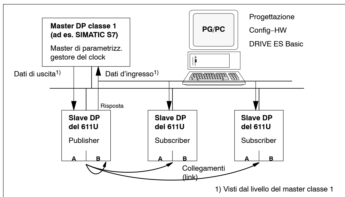
Fig. 5-30 Comunicazione con traffico trasversale con modello Publisher–Subscriber
