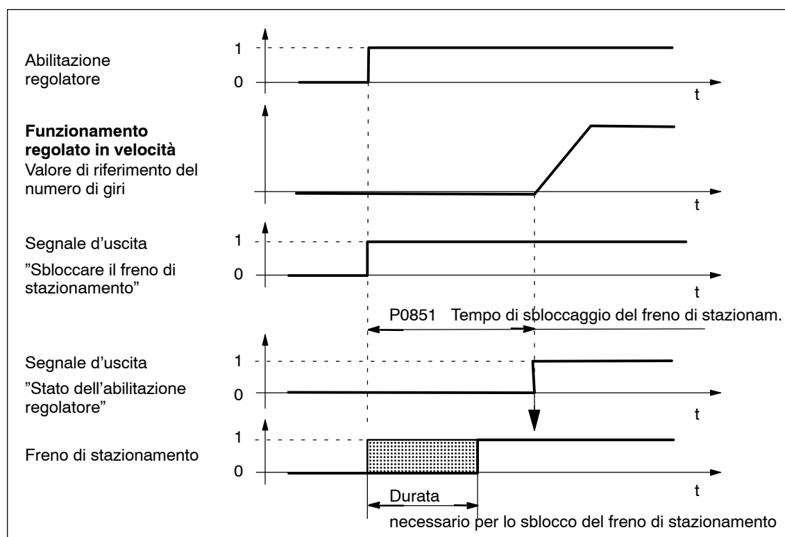
Fig. 6-75 Sbloccare il freno: comportamento all'attivazione del "Abilitazione regolatore"
