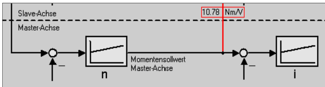
Fig. 6-53 Visualizzazione normalizzazione ingressi asse slave
