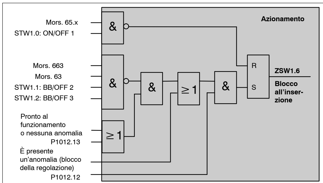
Fig. 5-9 Formazione del blocco inserzione
