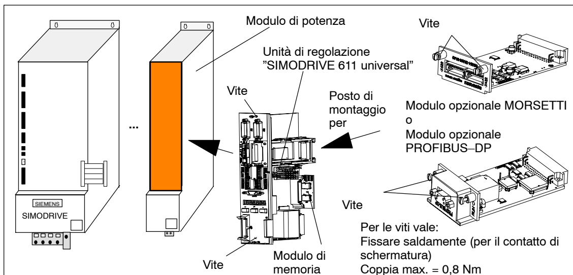
Fig. 2-1 Montaggio dell'unità di regolazione e di un modulo opzionale
