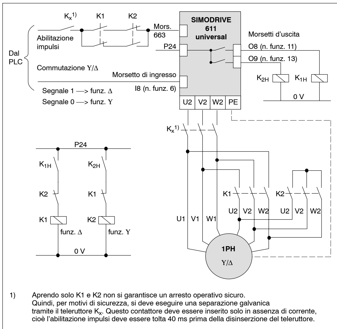
Fig. 6-83 Collegamento proposto: commutazione di un motore nel funzionamento stella/triangolo
