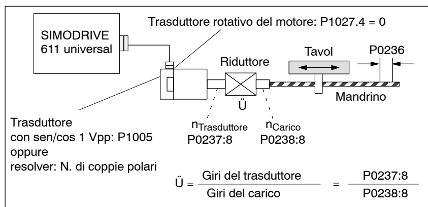
Fig. 6-10 Asse lineare con trasduttore rotativo del motore (vite a ricircolo di sfere)
