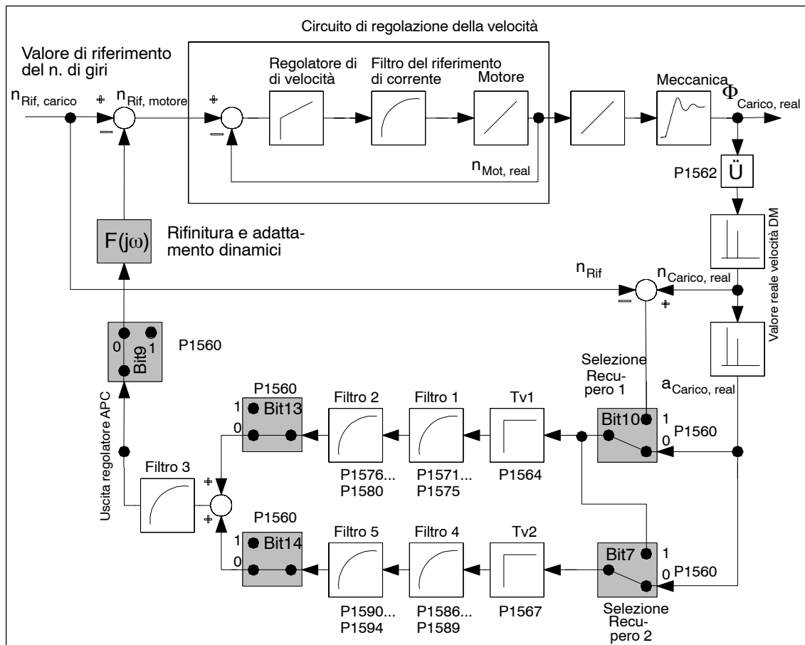
Fig. 6-93 Struttura di base APC
