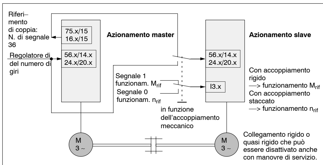
Fig. 6-59 Esempio: accoppiamento di 2 assi con il master/slave con gli ingressi/uscite analogici
