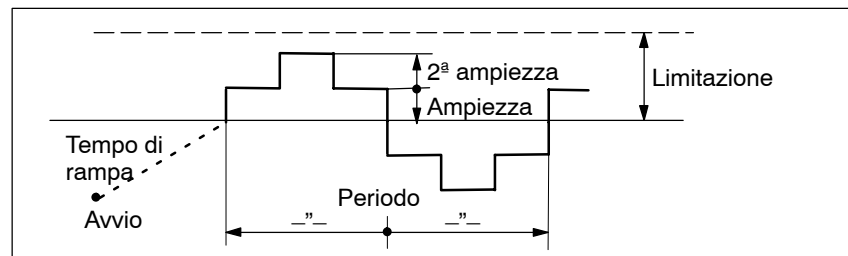
Fig. 7-7 Forma della curva a "gradini" con ampiezza > 0 e offset = 0
