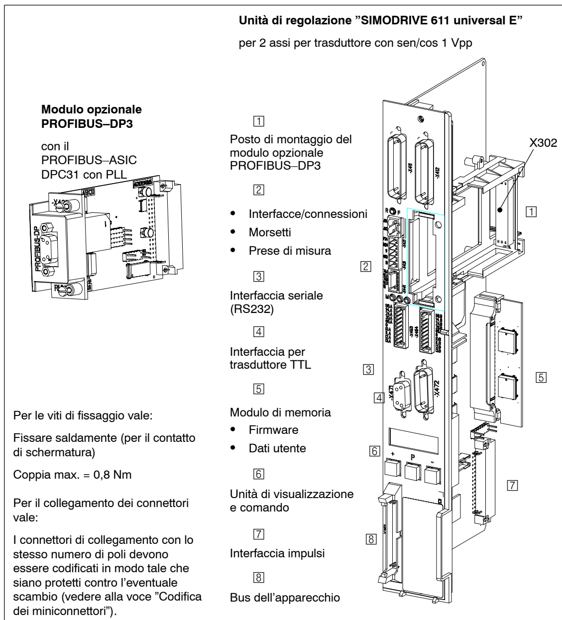
Fig. 1-9 Unità di regolazione "SIMODRIVE 611 universal E" con modulo opzionale PROFIBUS-DP3
