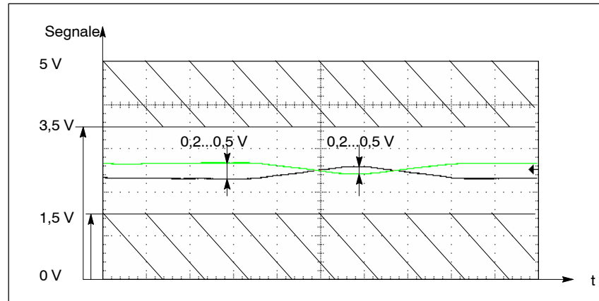
Fig. A-4 Andamento dei segnali in presenza di impulso di zero/segnale di riferimento R+ e R–
