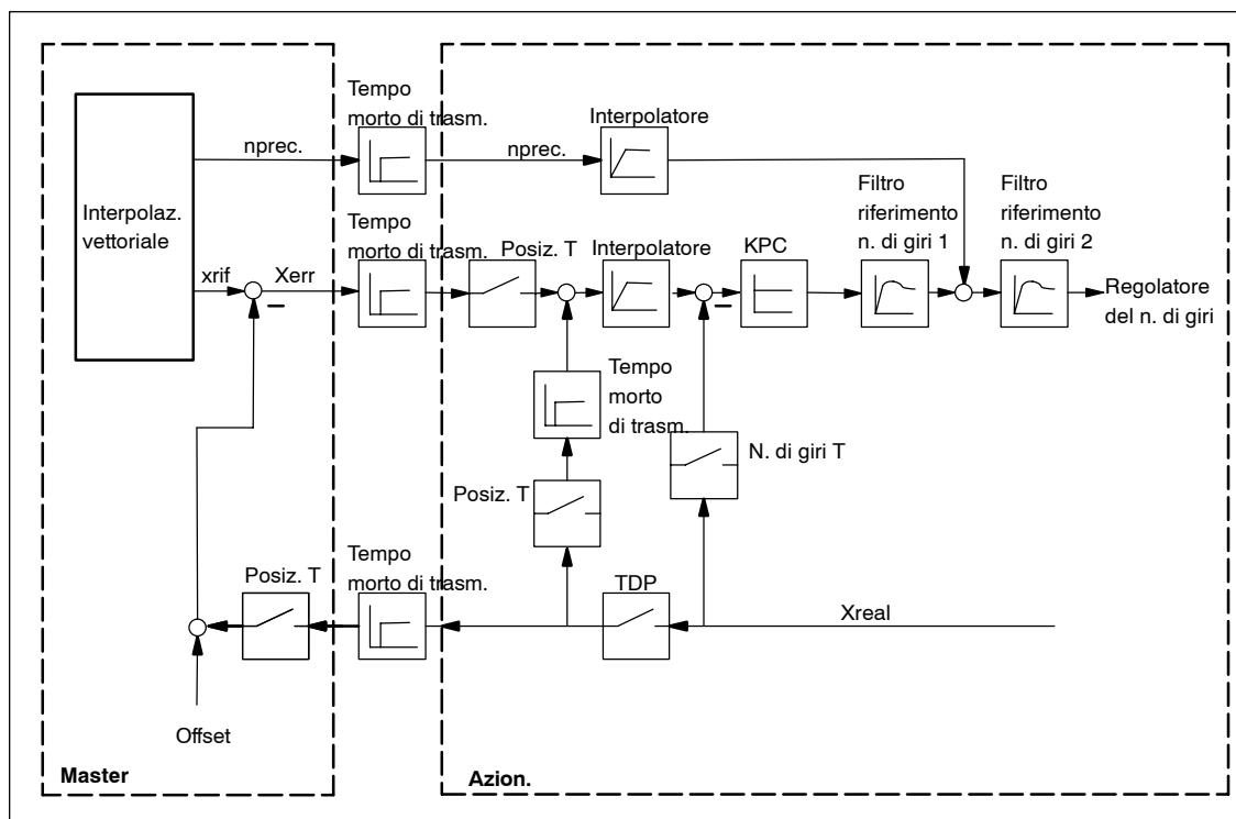
Fig. 6-85 Principio della regolazione dinamica della rigidità; il valore di riferimento del numero di giri viene utilizzato come precomando del numero di giri
