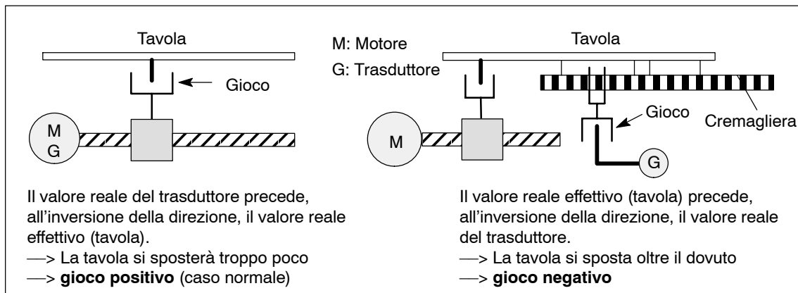
Fig. 6-16 Gioco all'inversione positivo e negativo
