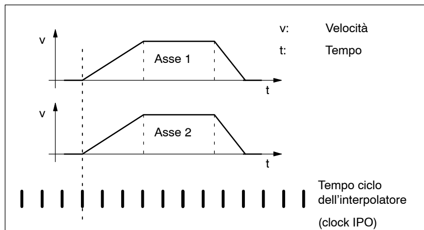
Fig. 5-27 Esempio: avvio contemporaneo del movimento
