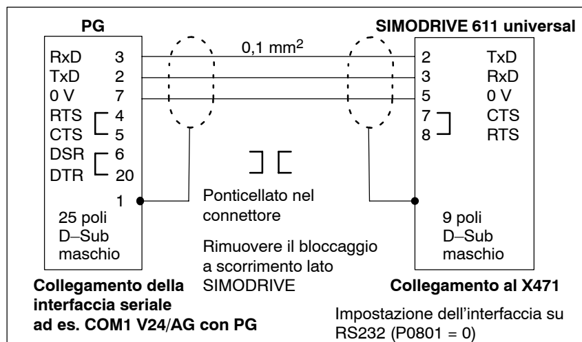
Fig. 2-13 Cavo di collegamento RS232: PG ↔ SIMODRIVE 611 universal
