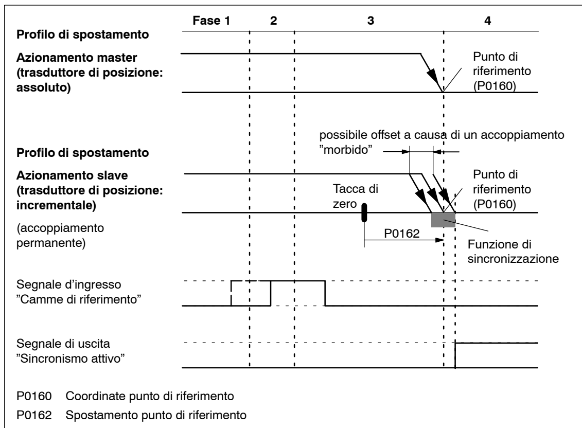
Fig. 6-40 Sequenza nella ricerca del punto di riferimento passiva (azionamento master con trasduttore assoluto, azionamento slave con trasduttore incrementale)
