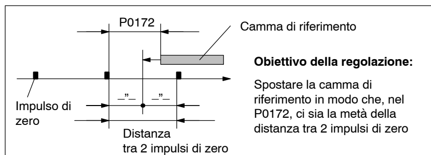
Fig. 6-23 Regolazione della camma di riferimento
