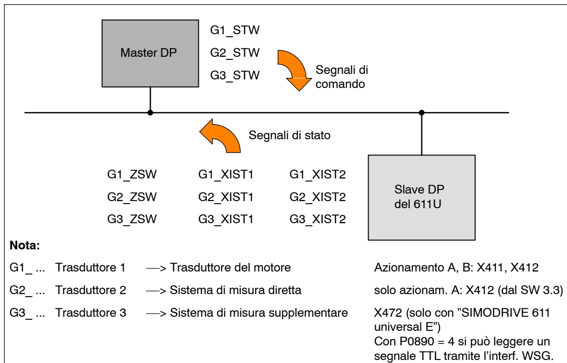
Fig. 5-13 Dati di processo dell'interfaccia del trasduttore
