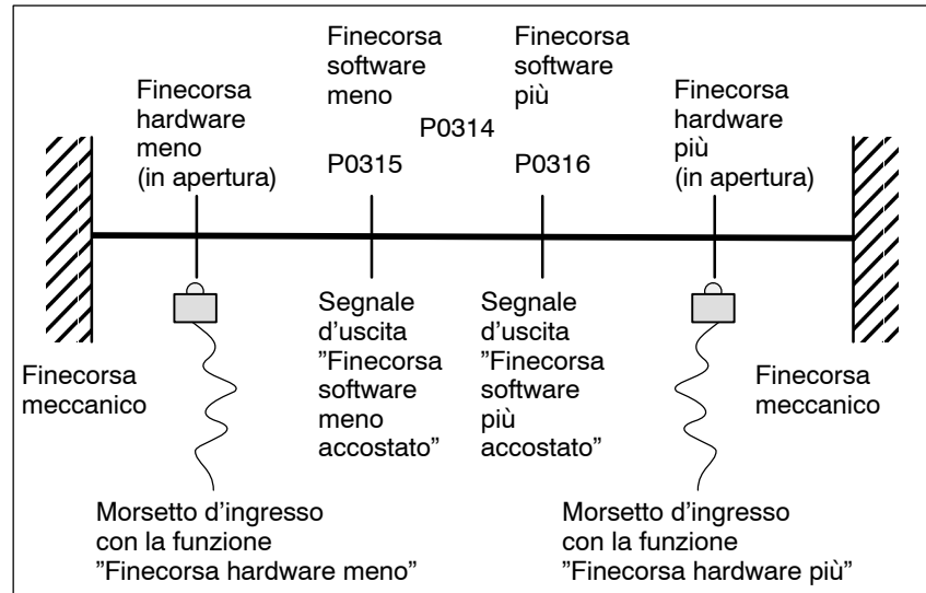
Fig. 6-15 Panoramica delle sorveglianze dei finecorsa
