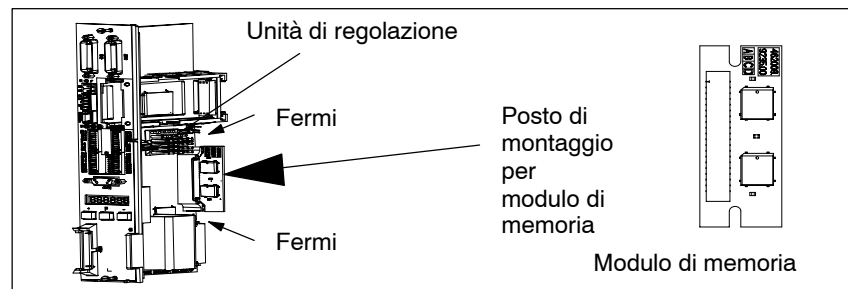
Fig. 2-2 Montaggio/smontaggio del modulo di memoria
