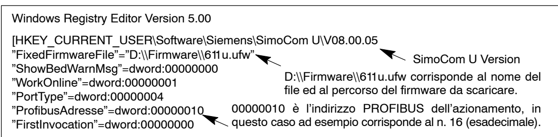
Fig. 4-2 Esempio di testo del file ".reg" per il collegamento tramite PROFIBUS-DP
