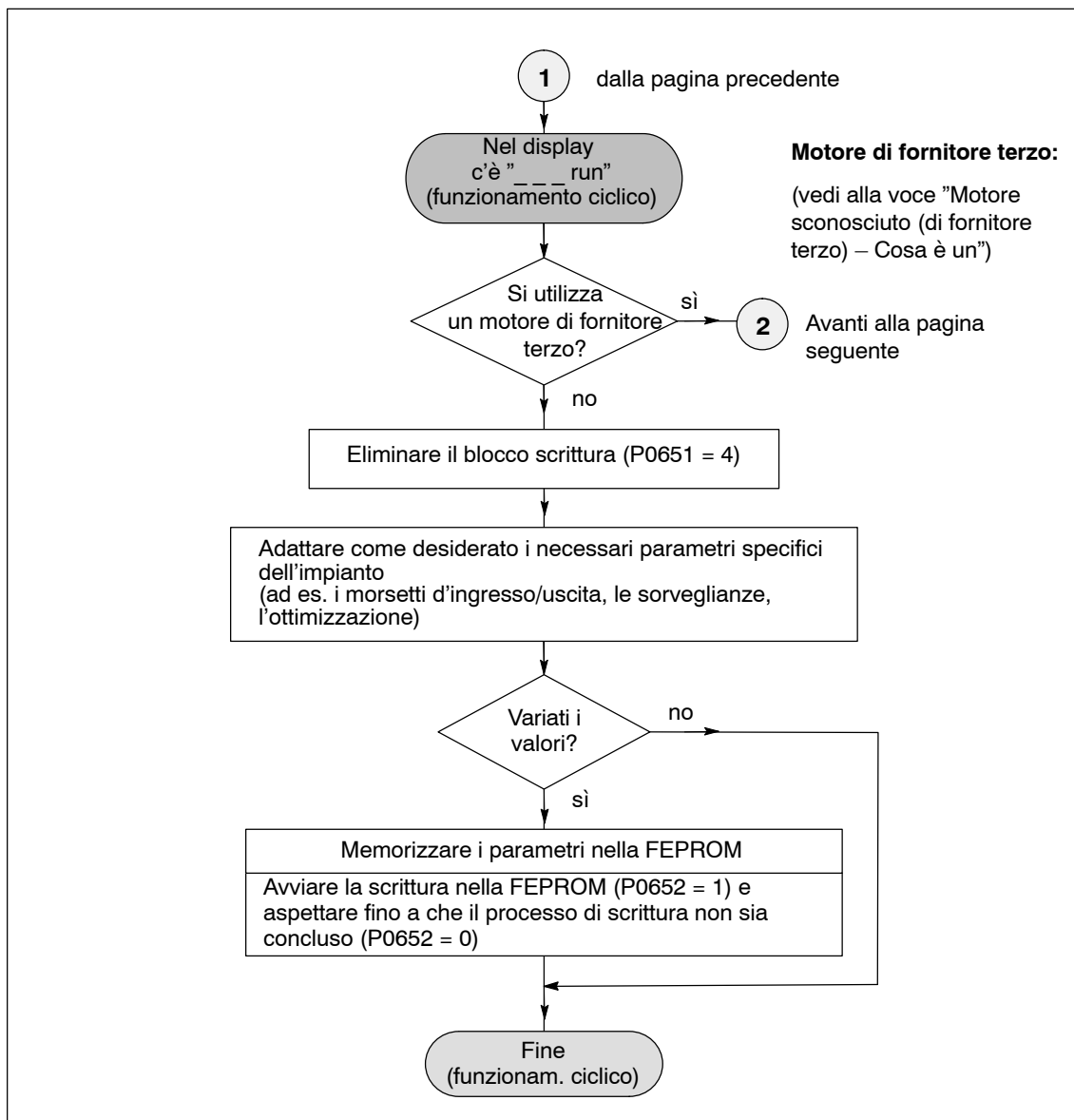
Fig. 4-4 Messa in servizio con l'unità di visualizzazione e comando (parte 2 di 3)
