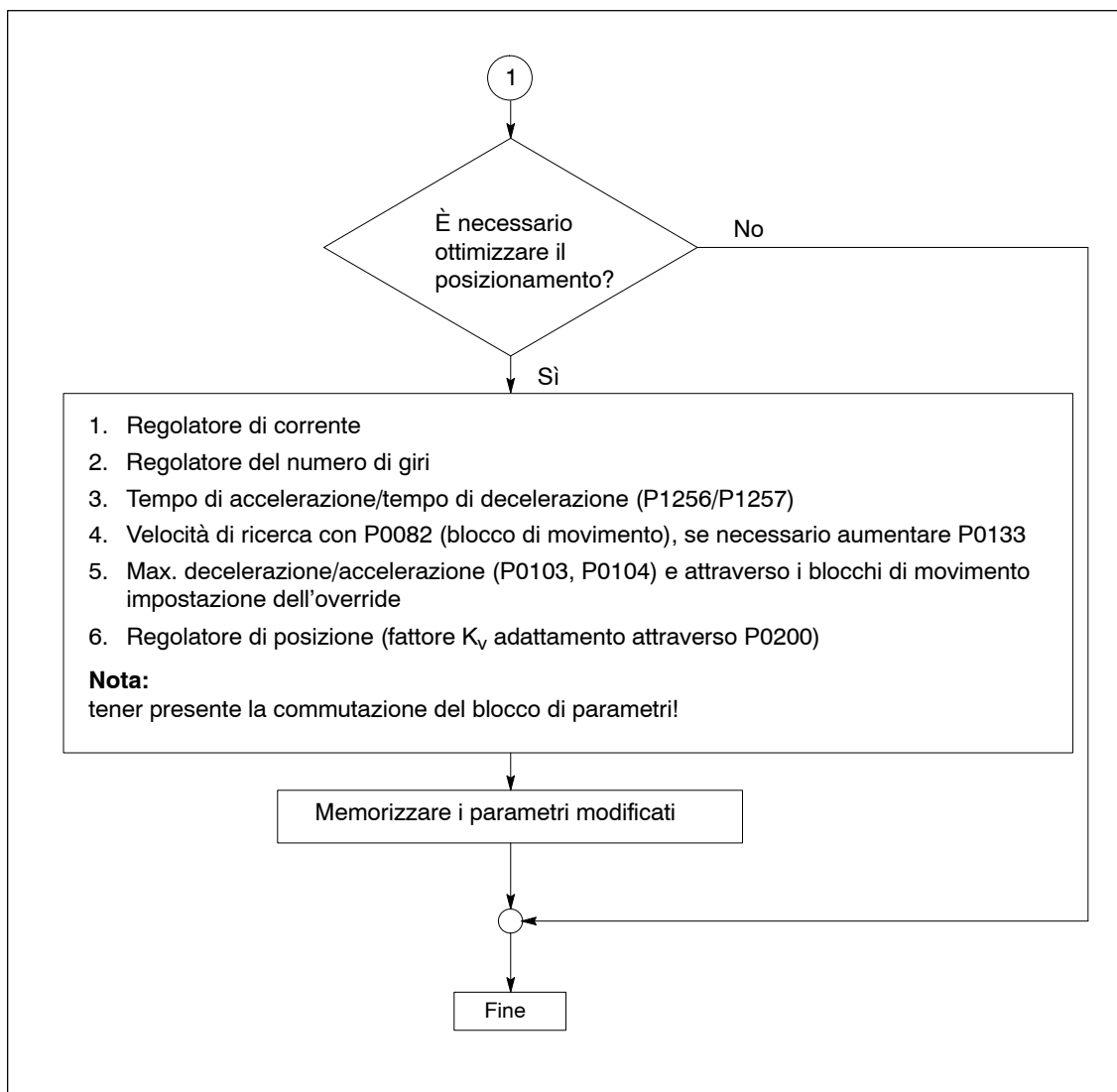
Fig. 6-90 Esempio di messa a punto del posizionamento mandrino, continuazione
