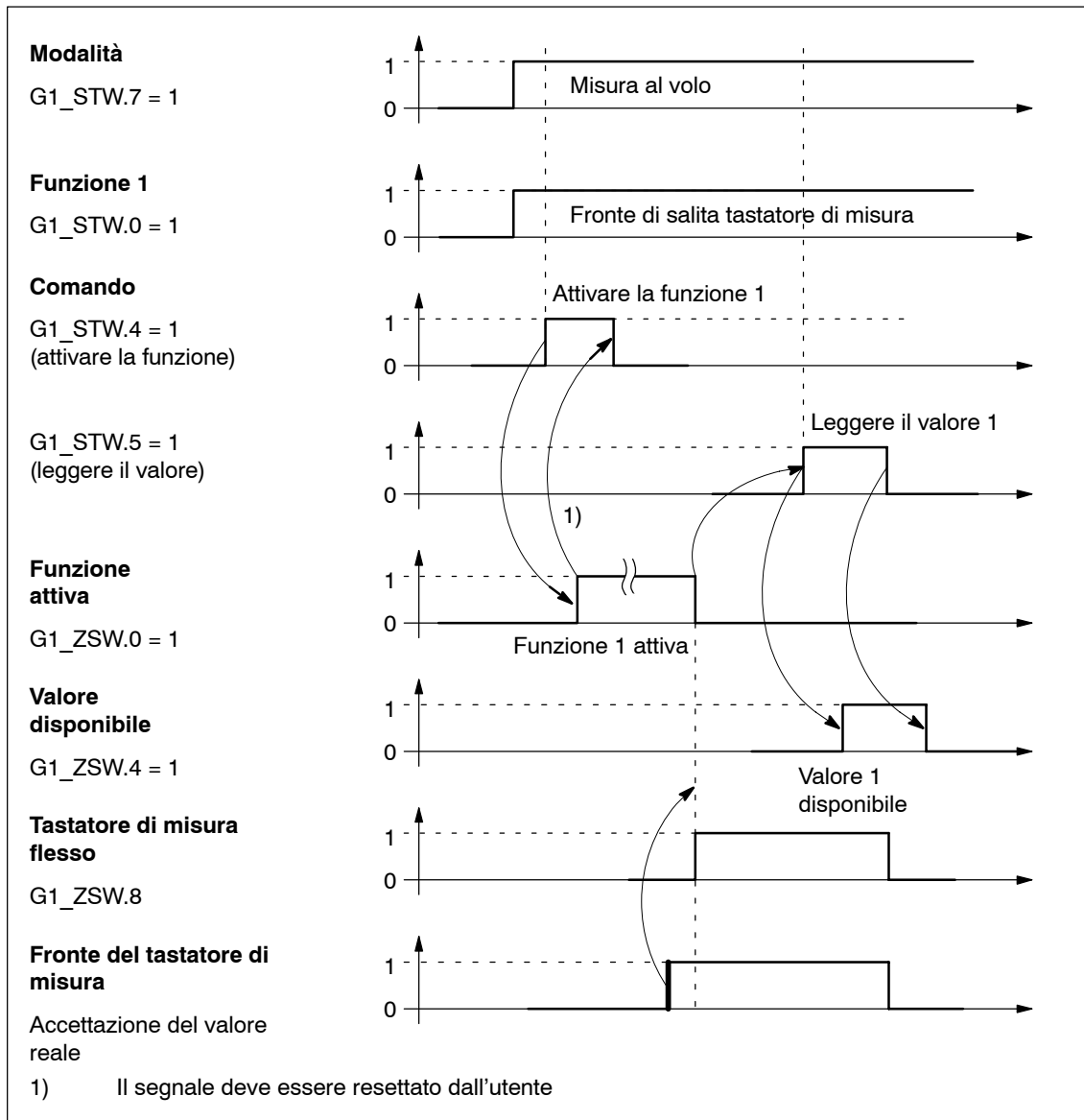
Fig. 5-15 Diagramma sequenziale con la funzione "Misure al volo"
