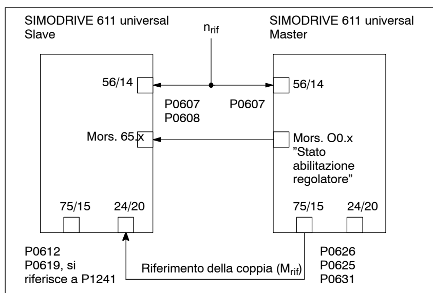
Fig. 6-49 Accoppiamento assi con 2 moduli monoasse per mezzo dei morsetti I/O
