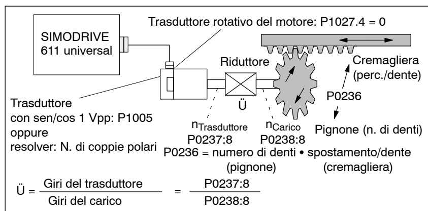
Fig. 6-11 Asse lineare con trasduttore rotativo del motore (pignone/cremagliera)
