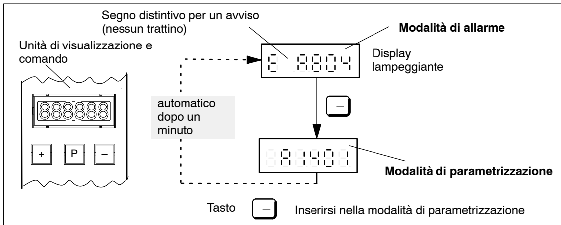
Fig. 7-3 Come comandare se è presente un avviso
