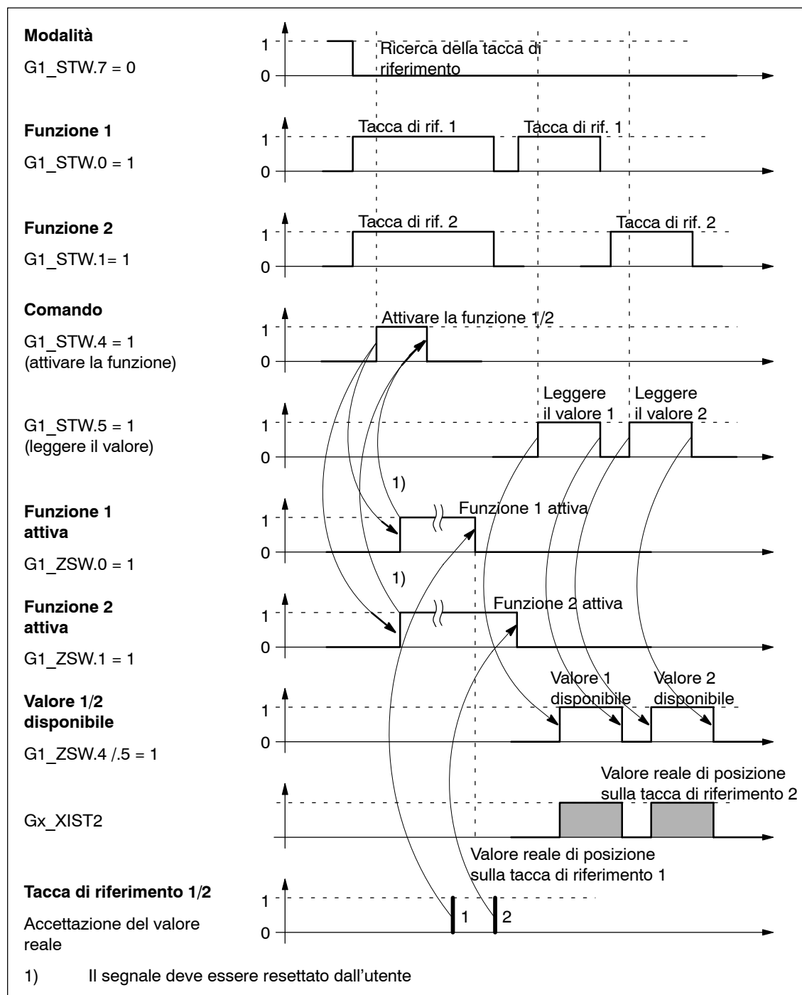
Fig. 5-14 Diagramma sequenziale con la funzione "Ricerca della tacca di riferimento"
