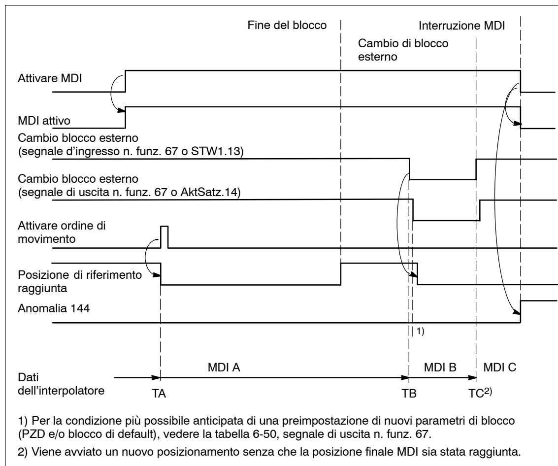
Fig. 6-30 Segnali di comando e di stato in MDI
