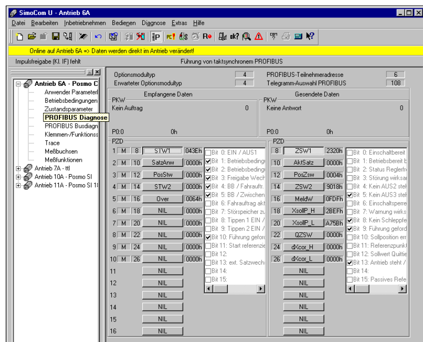
Fig. 5-38 Parametrizzazione azionamento master
