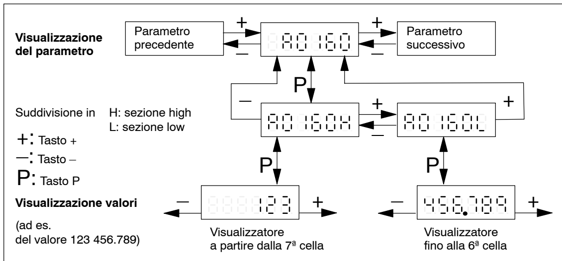
Fig. 3-4 Comando in caso di parametri senza sottoparametri e visualizzazione dei valori > 6 posizioni
