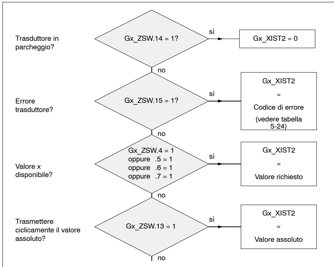
Fig. 5-17 Priorità per le funzioni e Gx_XIST2
