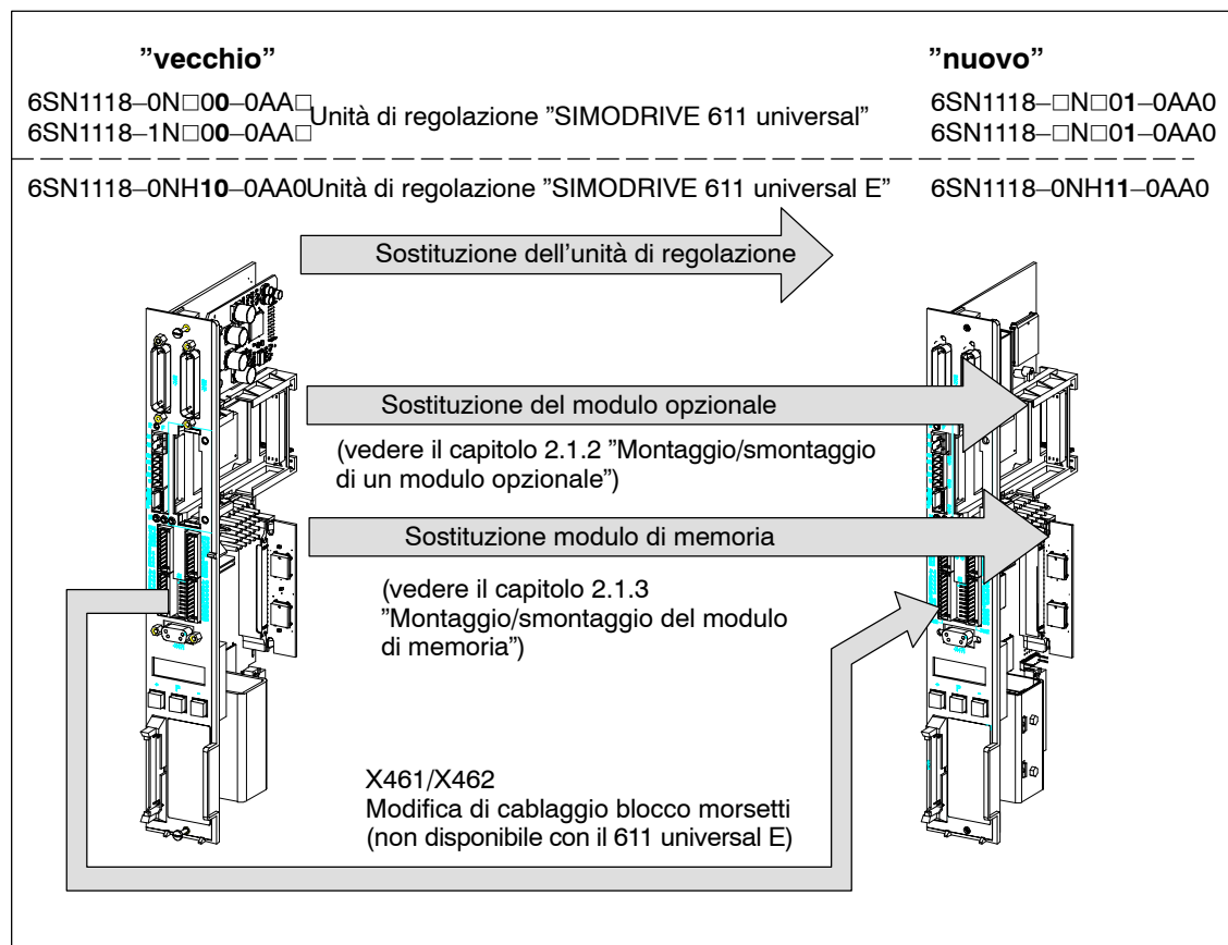
Fig. 2-3 Sostituzione di una unità di regolazione difettosa con una nuova di tipo HR
