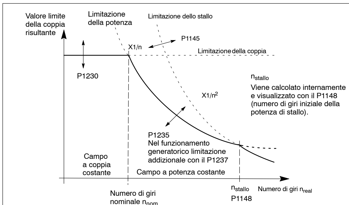
Fig. 6-7 Limitazione del riferimento di coppia
