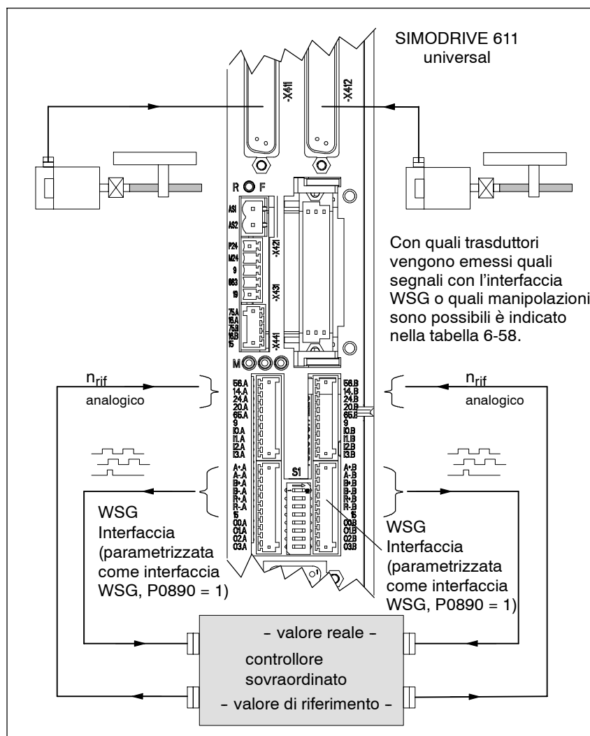
Fig. 6-67 Interfaccia WSG parametrizzata come uscita
