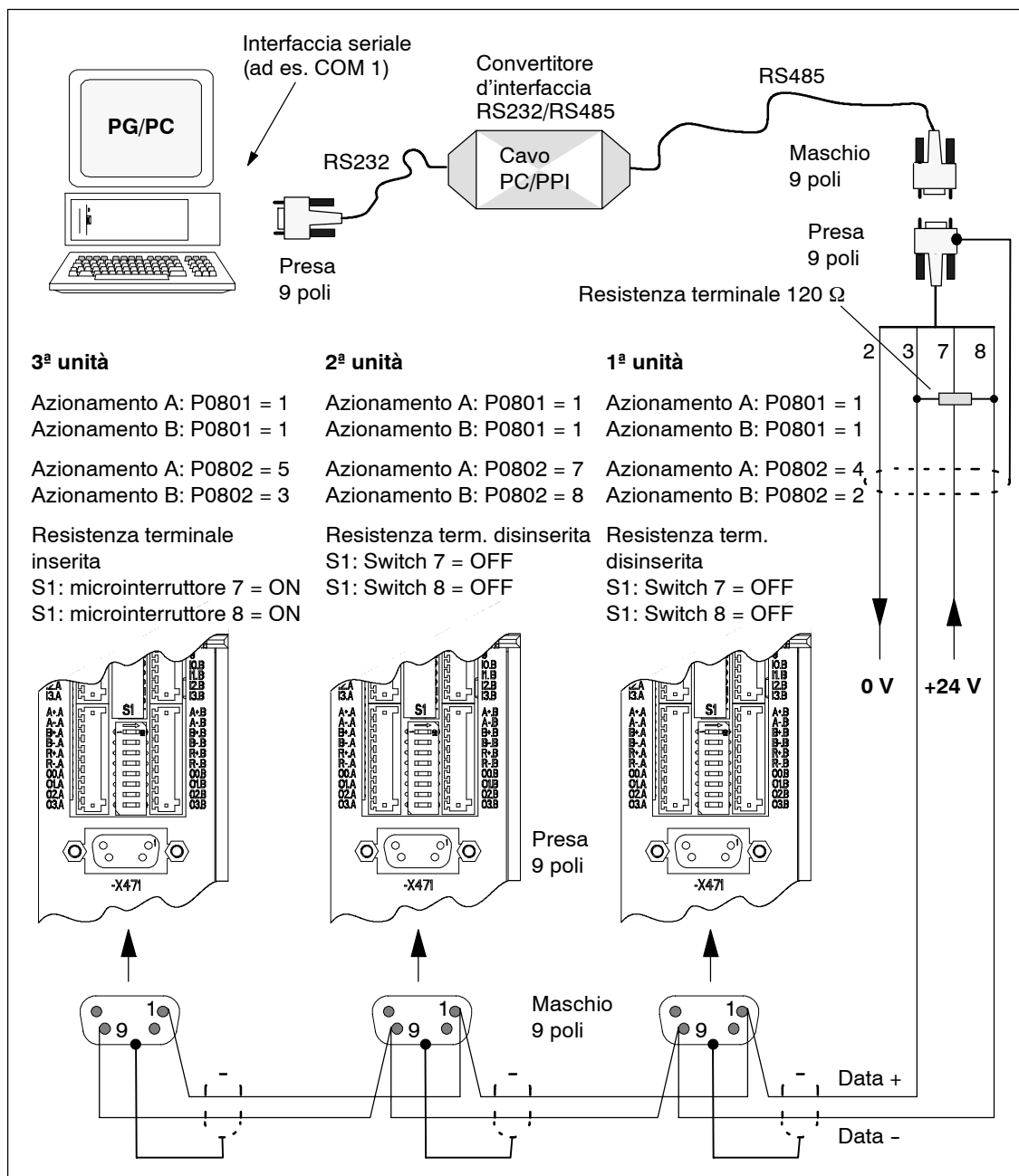
Fig. 3-10 Comunicazione tramite RS485 (esempio con 3 nodi/partner)
