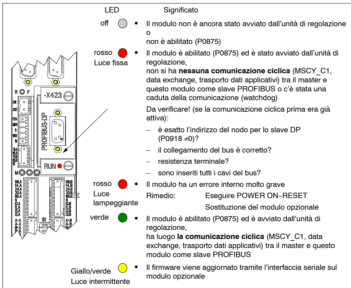
Fig. 5-22 Visualizzazioni LED per la diagnostica
