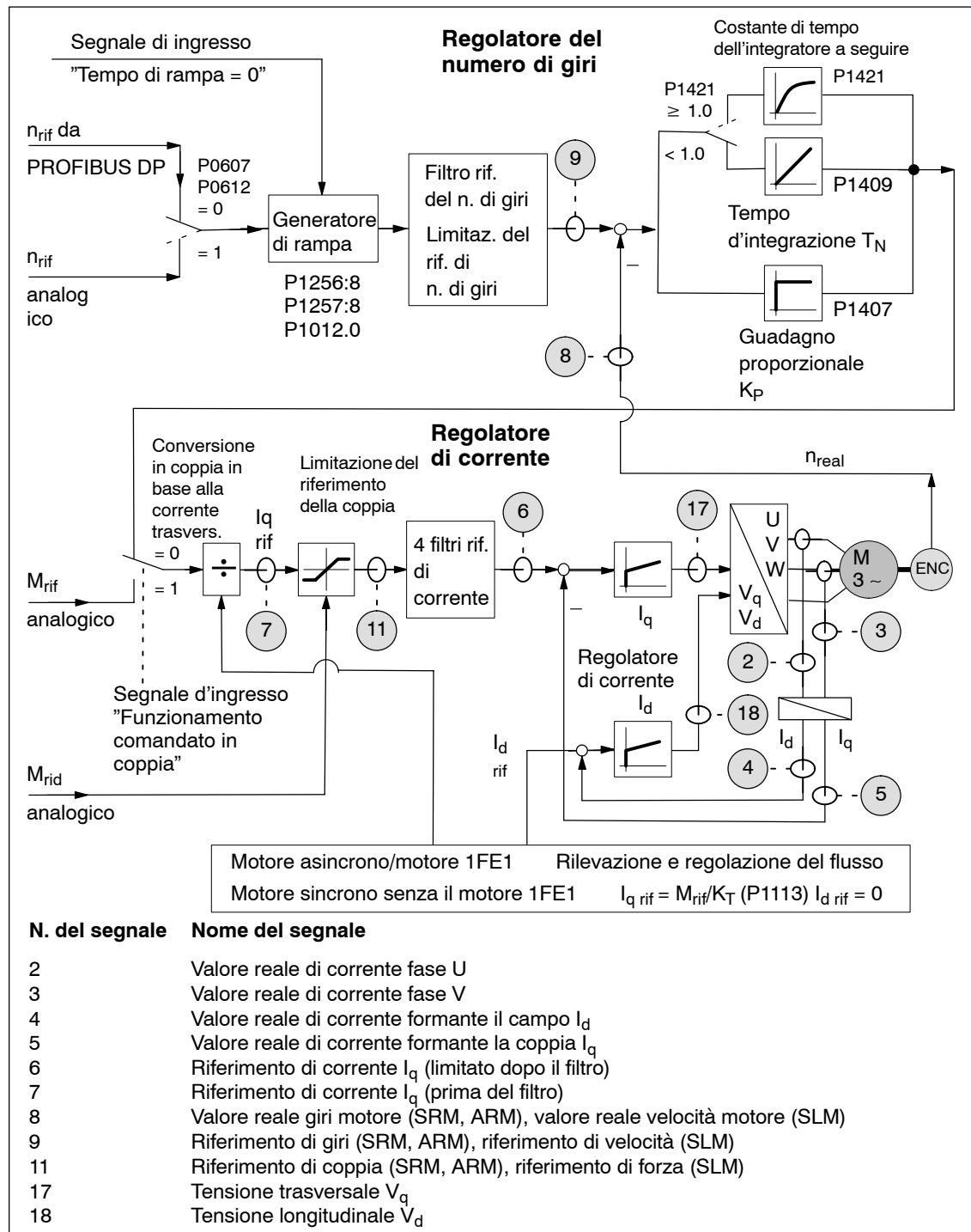
Fig. 6-60 Segnali analogici per il circuito di regolazione della corrente/del n. di giri
