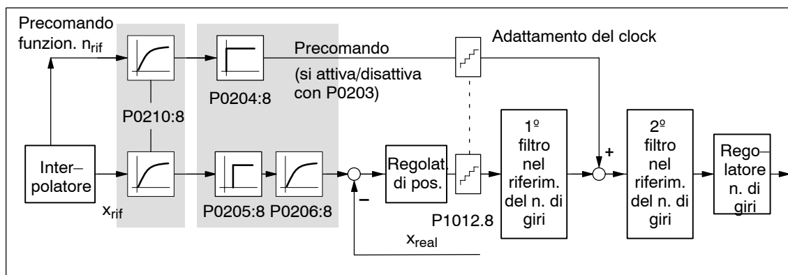
Fig. 6-17 Precomando del regolatore del numero di giri
