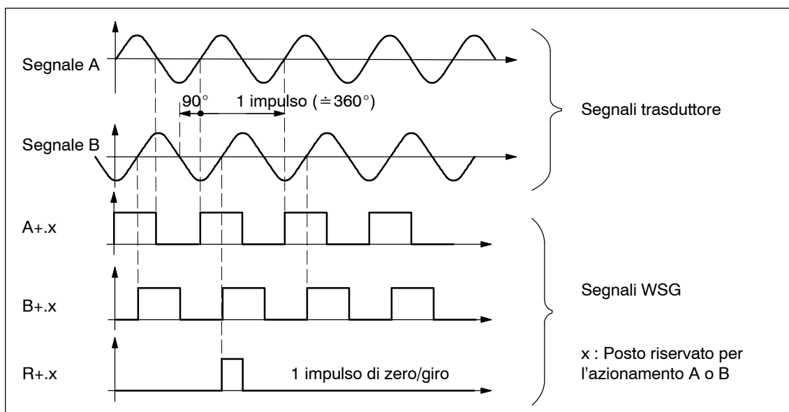
Fig. 6-69 Segnali WSG con i trasduttori incrementali con sen/cos 1Vpp
