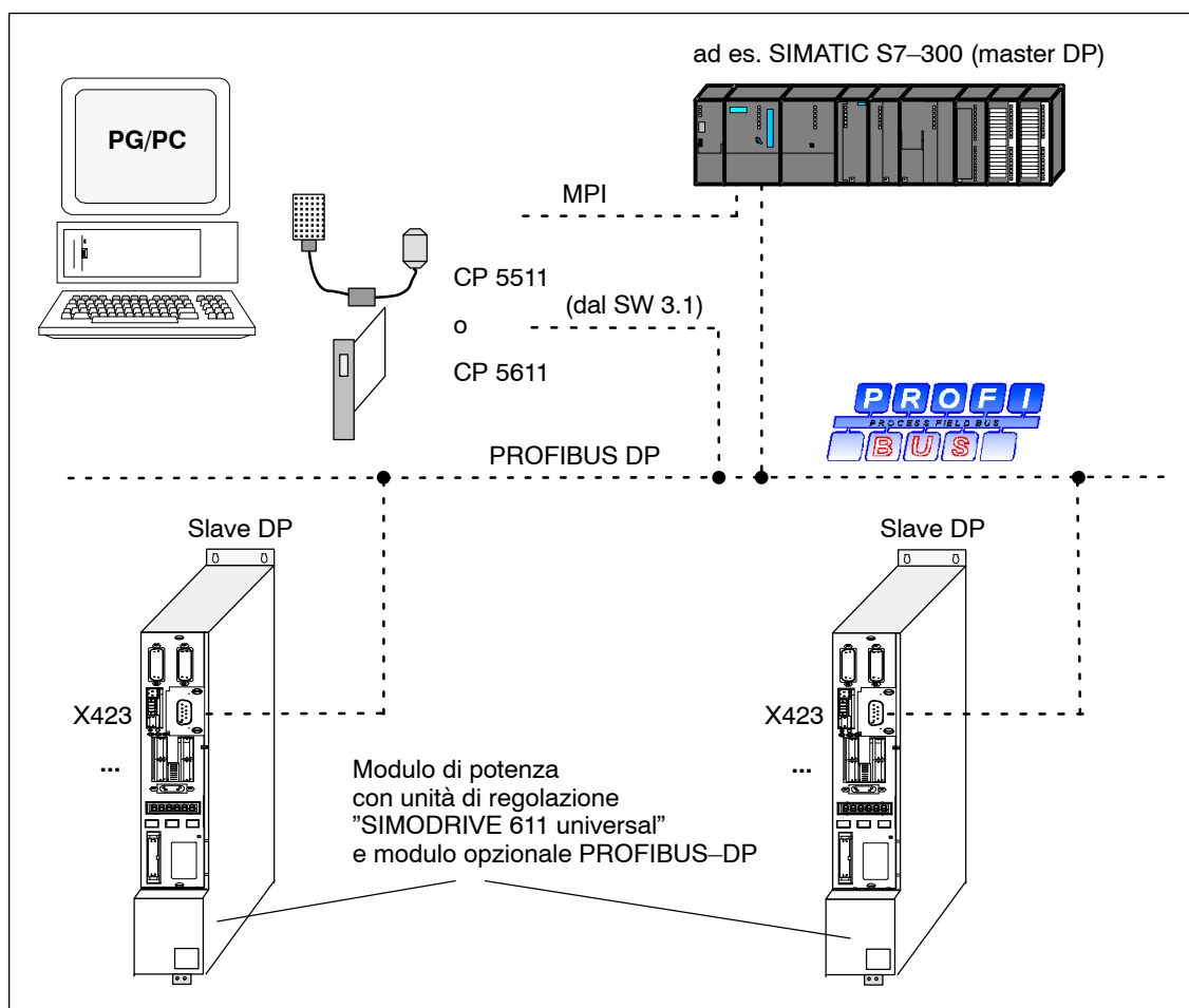
Fig. 2-9 Schema di collegamento del modulo opzionale PROFIBUS-DP
