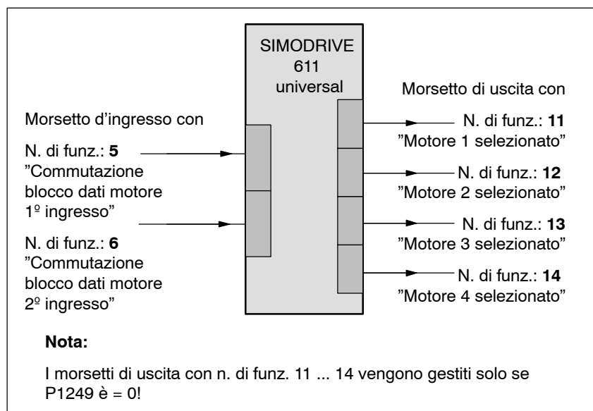
Fig. 6-80 Segnali di ingresso/uscita: morsetti liberamente parametrizzabili
