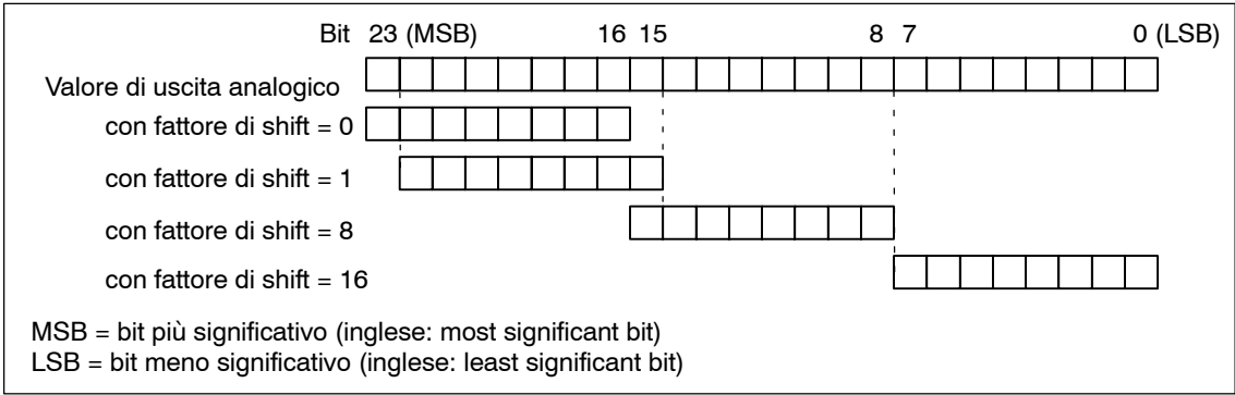
Fig. 6-62 Fattore di shift per l'uscita analogica dei segnali a 24 bit
