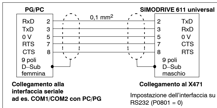
Fig. 2-11 Cavo di collegamento RS232 con i conduttori RTS/CTS: PG/PC ↔ SIMODRIVE 611 universal
