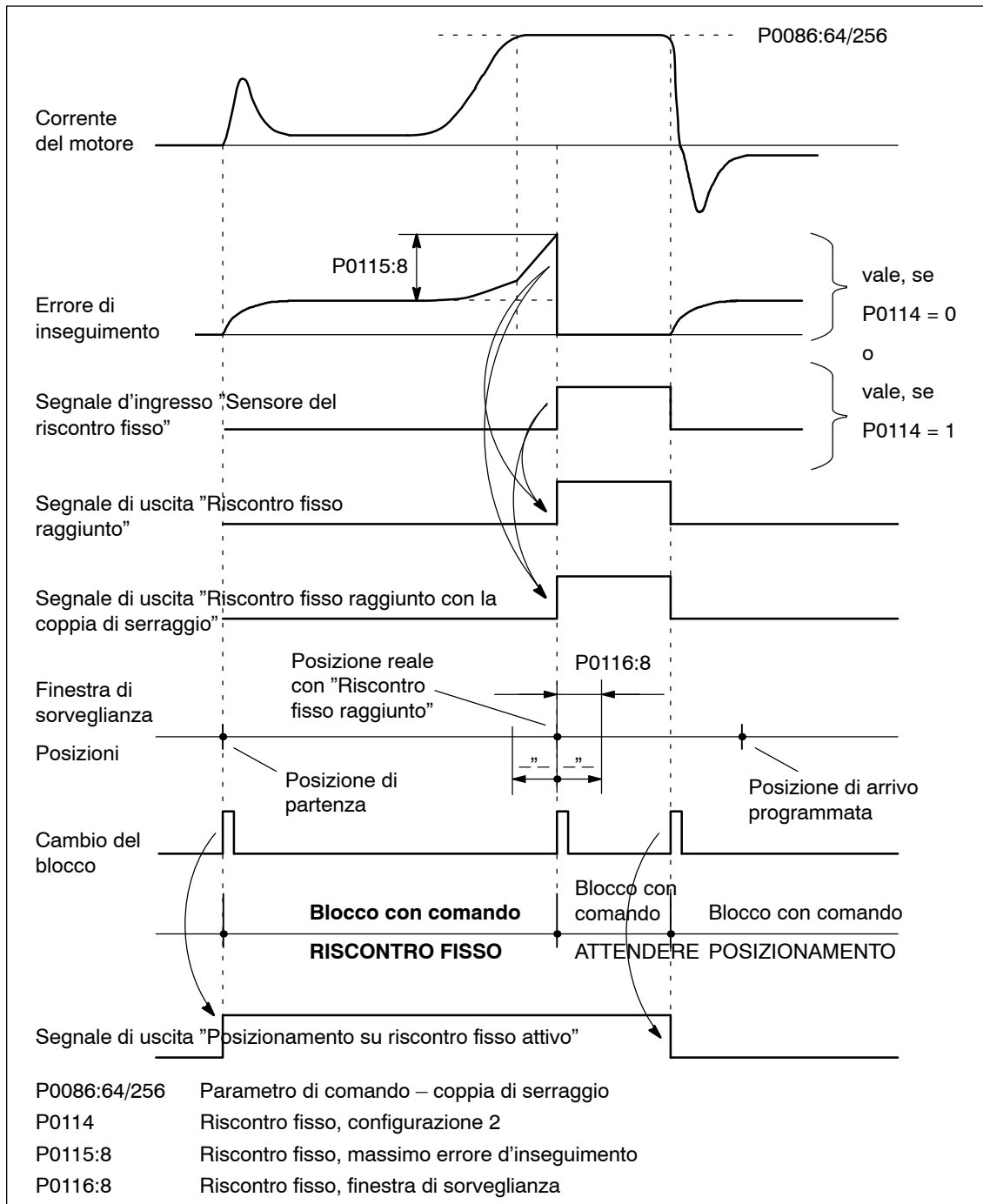
Fig. 6-84 Andamento dei segnali con la funzione "Posizionamento su riscontro fisso"
