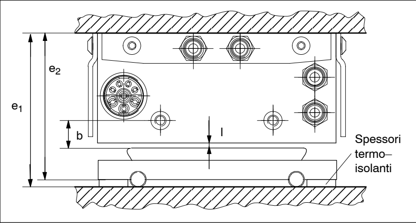
Fig. 4-14 Dimensioni di controllo per il montaggio del motore 1FN1
