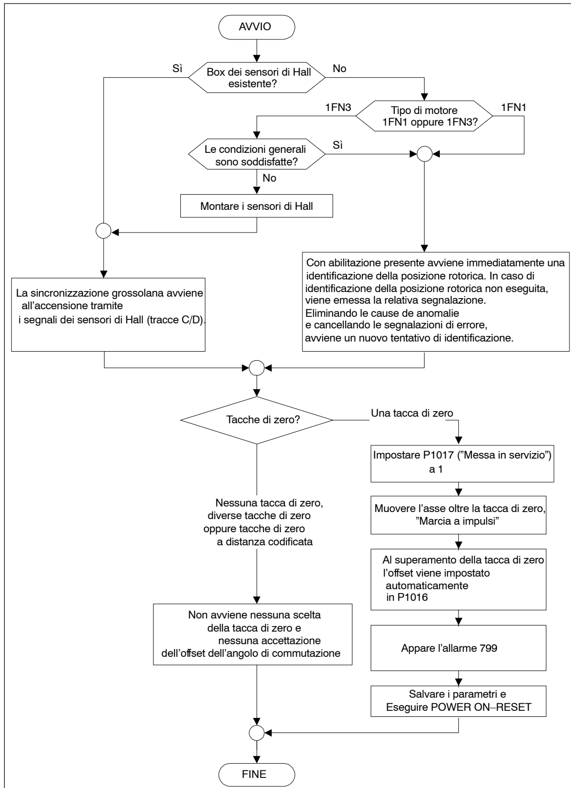
Fig. 4-12 Sistema di misura incrementale
