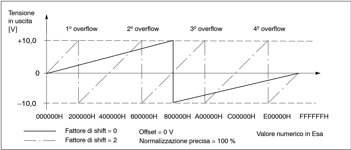
Fig. 6-65 Tensione d'uscita analogica senza la protezione alla saturazione (P0631/P0638 = 0)
