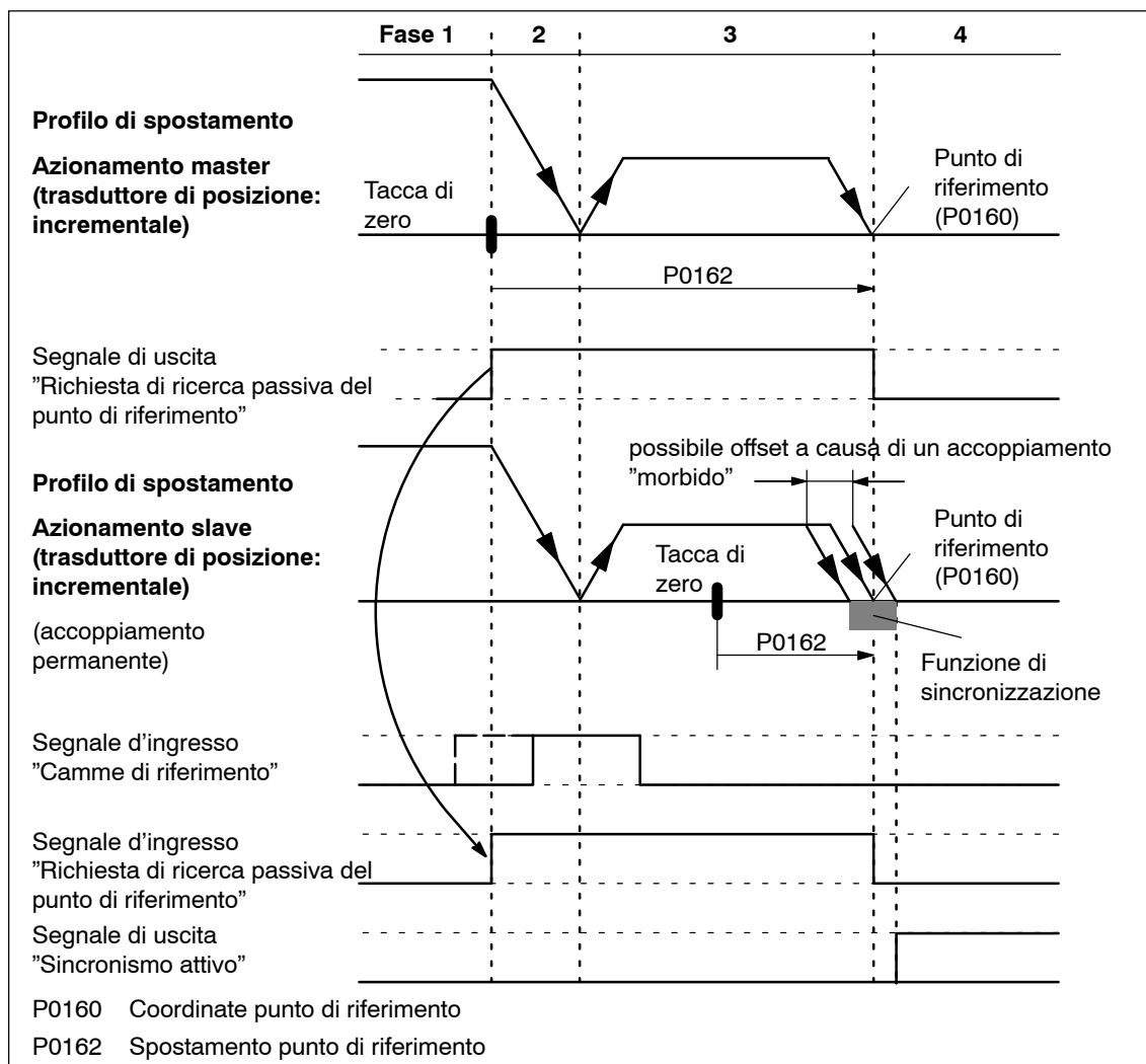
Fig. 6-39 Sequenza nella ricerca del punto di riferimento passiva (azionamento master e azionamento slave con trasduttore incrementale)
