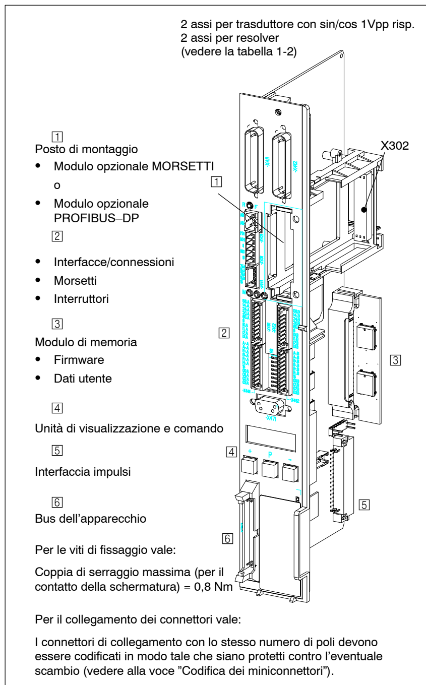
Fig. 1-3 Unità di regolazione per 2 assi
