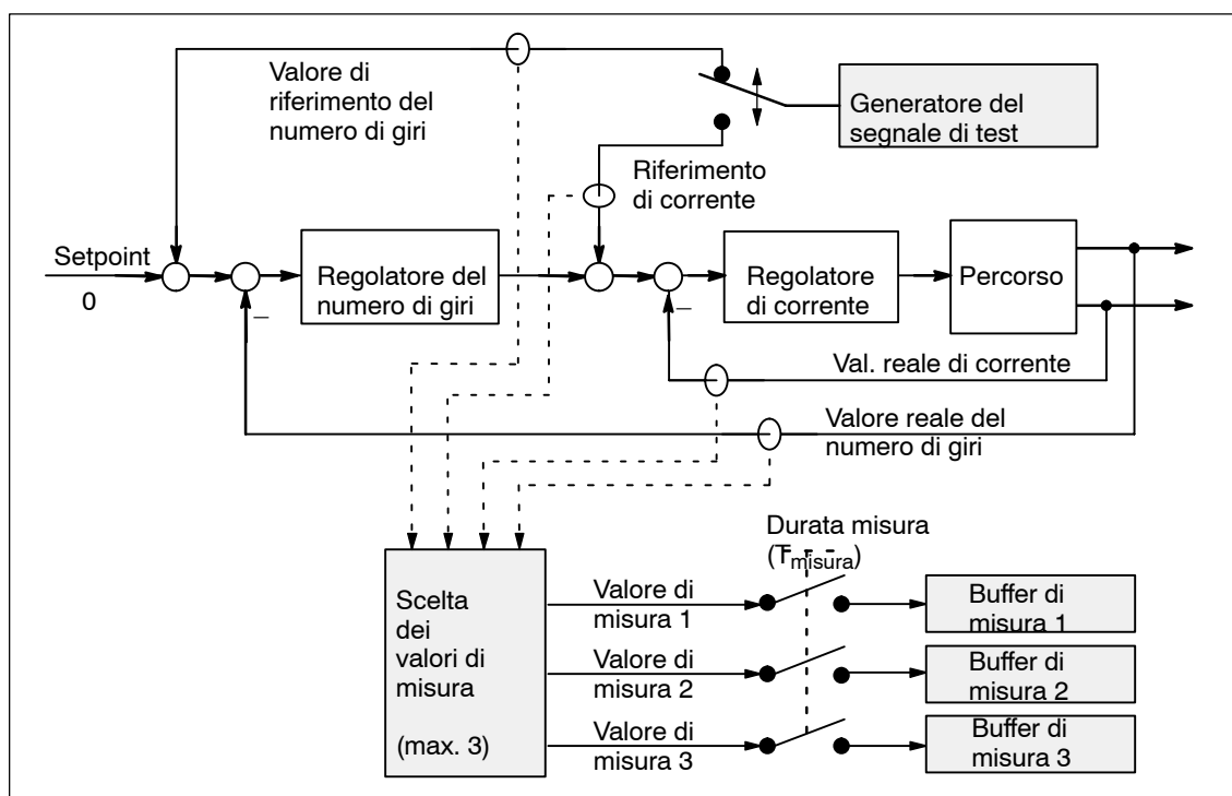
Fig. 7-11 Schema a blocchi della misura dell'azionamento
