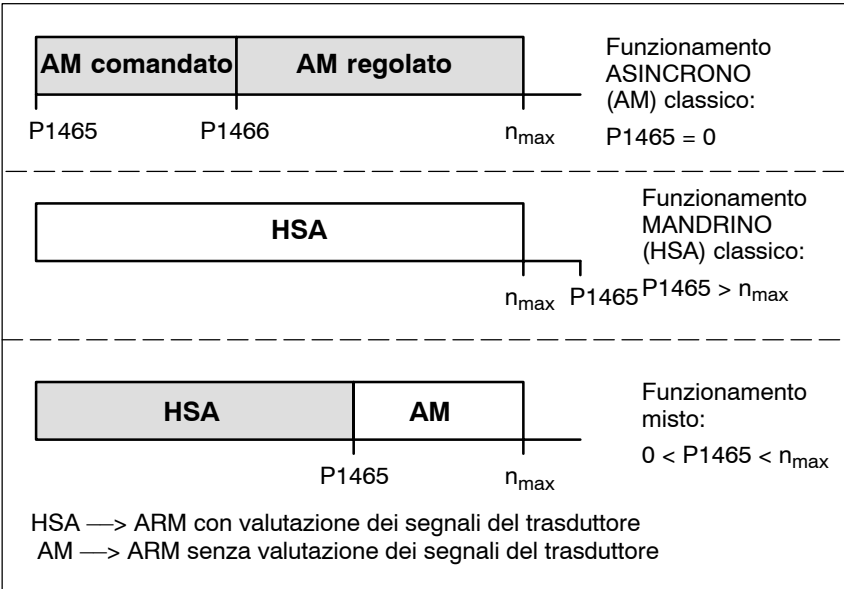
Fig. 4-6 Settori di funzionamento MANDRINO/ASINCRONO
