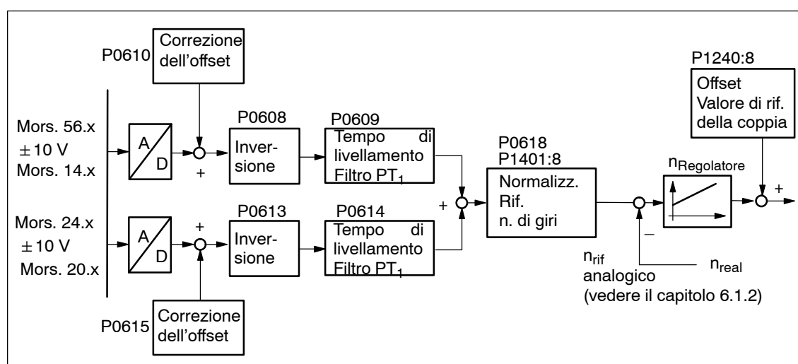
Fig. 6-55 Funzionamento regolato in velocità con i mors. 56.x/14.x e/o i mors. 24.x/20.x
