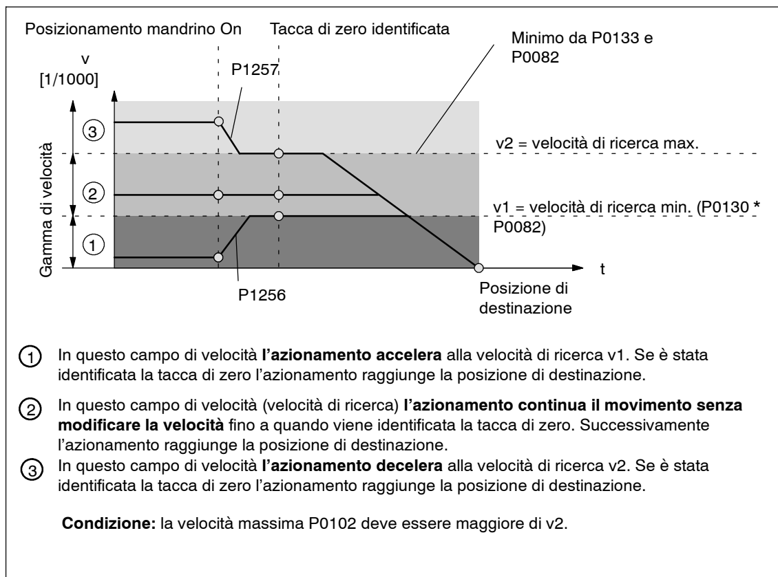
Fig. 6-88 Posizionamento mandrino con n-rif, se è stata eseguita in precedenza la ricerca del punto zero
