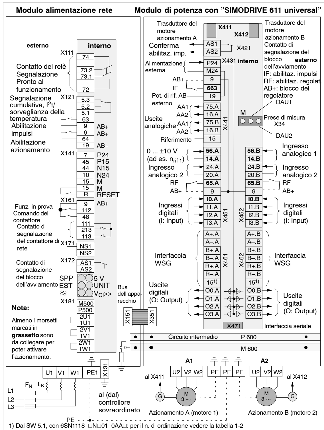
Fig. 2-7 Schema di collegamento per l'unità di regolazione
