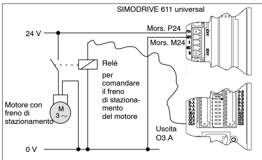
Fig. 6-78 Esempio: comandare il freno di stazionamento del motore con l'uscita O3.A
