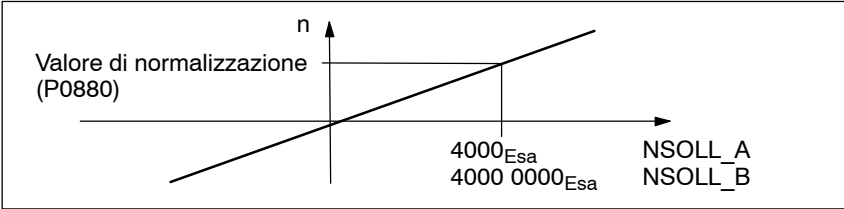
Fig. 5-10 Normalizzazione della velocità
