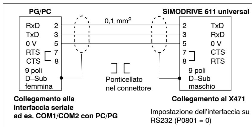
Fig. 2-12 Cavo di collegamento RS232 senza i conduttori RTS/CTS: PG/PC ↔ SIMODRIVE 611 universal
