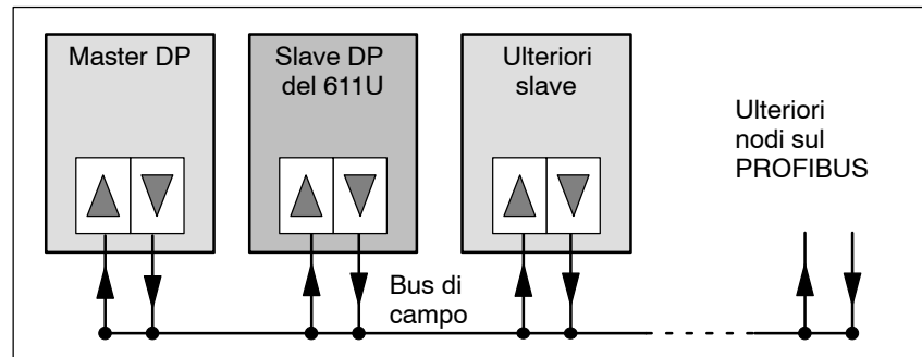
Fig. 5-1 Scambio dei dati con il PROFIBUS
