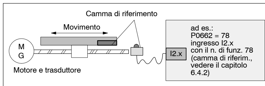
Fig. 6-22 Montaggio di una camma di riferimento
