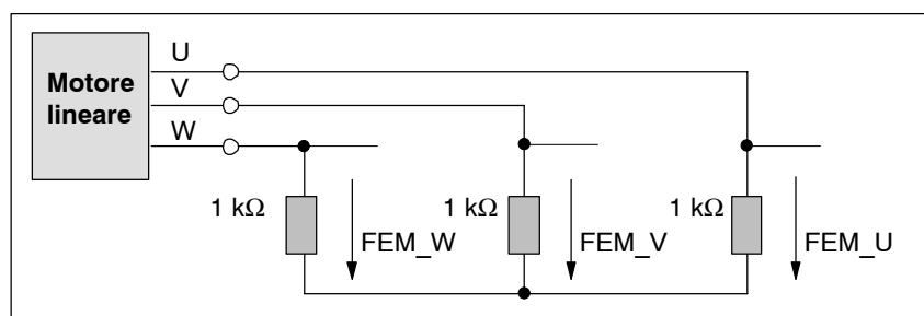
Fig. 4-20 Disposizione per la verifica delle misure
