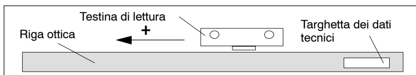
Fig. 4-18 Rilevamento della direzione di conteggio con il sistema di misura della ditta Heidenhain
