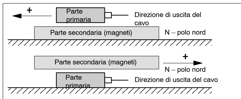
Fig. 4-21 Determinazione della direzione positiva del motore (campo rotante destrorso)
