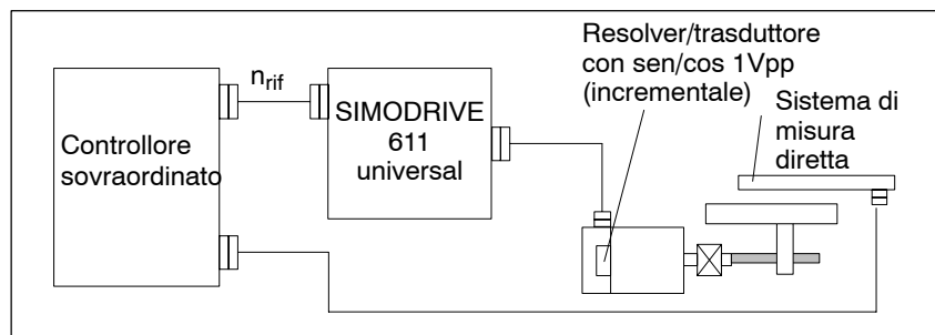
Fig. 6-3 Posizionamento per mezzo di un controllore sovraordinato, rilevamento del valore reale di posizione attraverso il sistema di misura diretta
