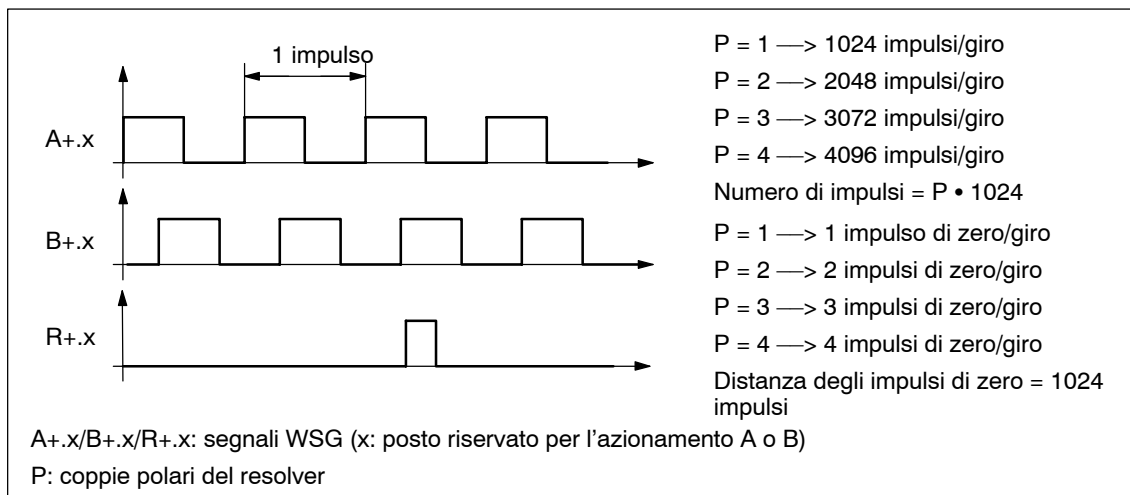
Fig. 6-68 Segnali WSG con i resolver
