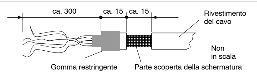
Fig. 2-6 Preparazione del finale del cavo per il collegamento della schermatura
