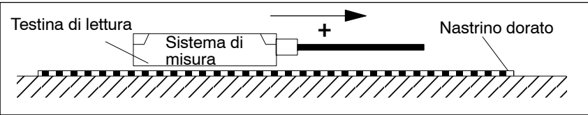
Fig. 4-19 Rilevamento della direzione di conteggio con il sistema di misura della ditta Renishaw
