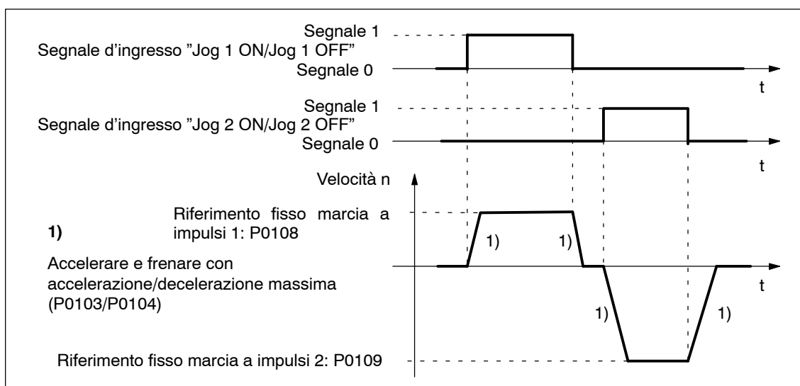
Fig. 6-25 Accelerazione e frenatura nella marcia a impulsi
