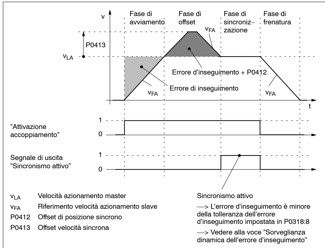
Fig. 6-36 Sincronismo di posizione (P0410 = 2 o 4)
