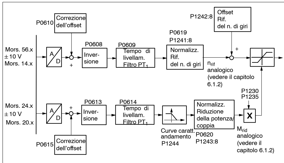
Fig. 6-58 Funzionamento comandato in coppia con i mors. 56.x/14.x e riduzione della coppia/potenza con i mors. 24.x/20.x
