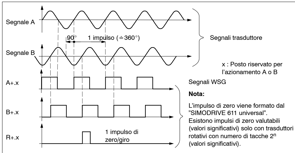
Fig. 6-70 Segnali WSG con i trasduttori assoluti con sen/cos 1Vpp e interfaccia EnDat
