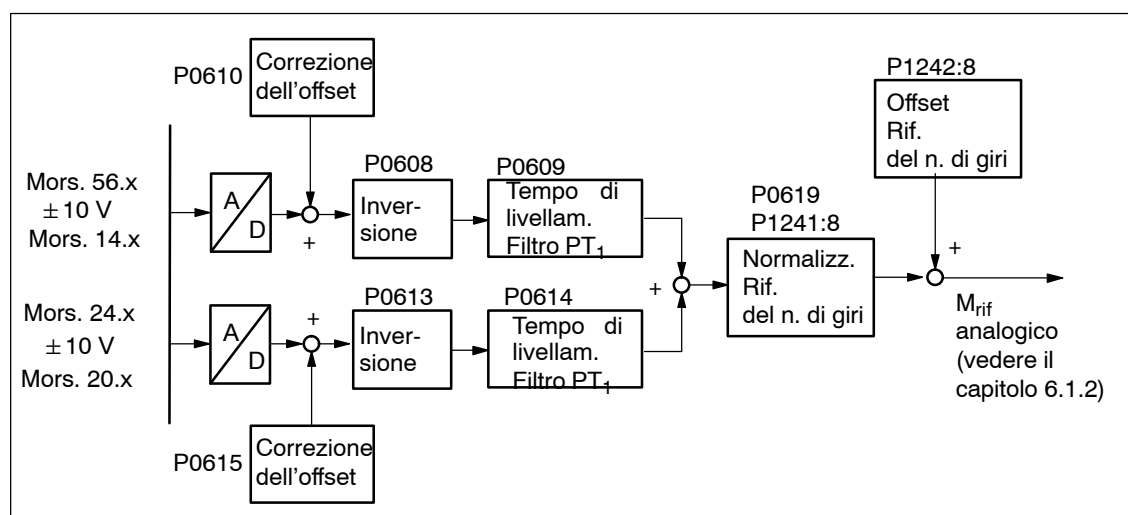
Fig. 6-57 Funzionamento comandato in coppia tramite i mors. 56.x/14.x e/o i mors. 24.x/20.x
