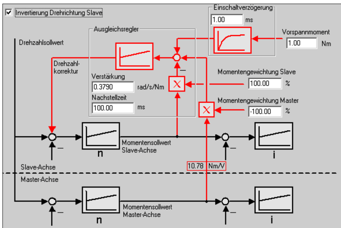
Fig. 6-54 Inversione direzione di rotazione asse slave
