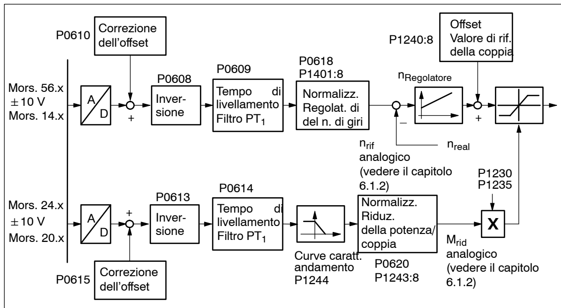
Fig. 6-56 Funzionamento regolato in velocità con i mors. 56.x/14.x e riduzione della coppia/potenza con i mors. 24.x/20.x
