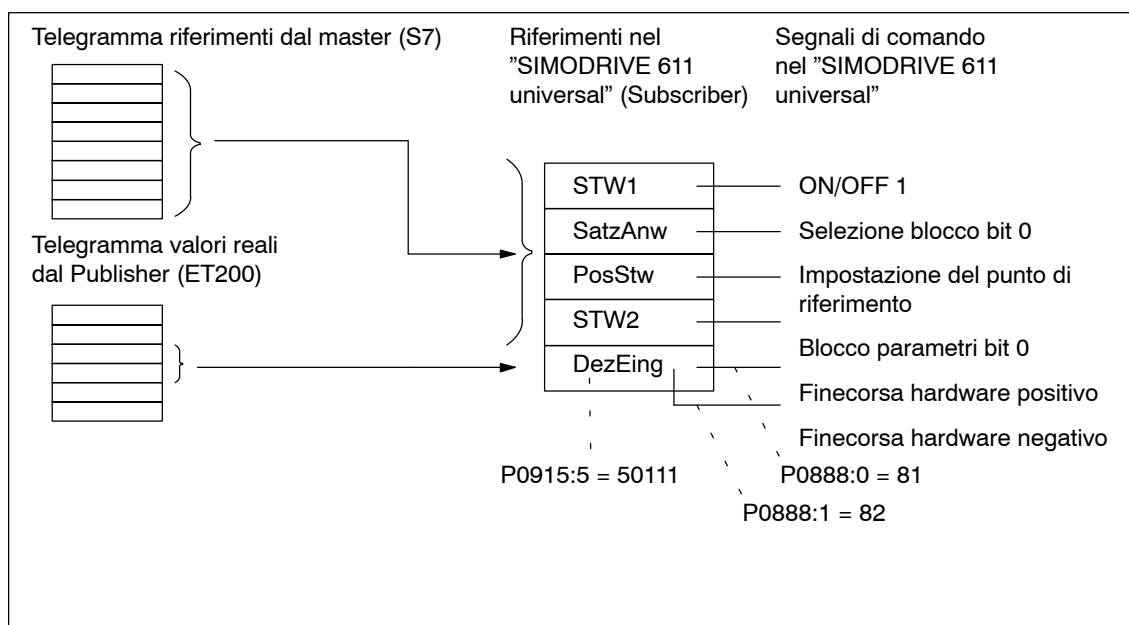
Fig. 5-34 Esempio di funzionamento misto con segnali di comando
