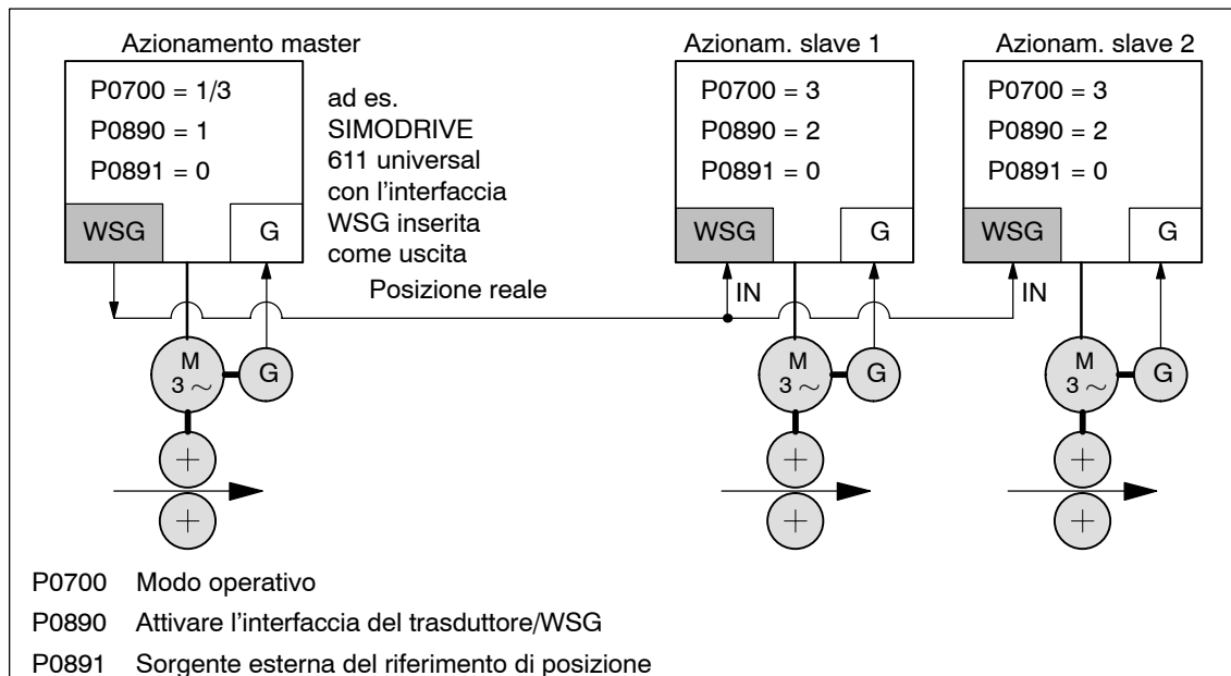
Fig. 6-31 Interfaccia WSG come fonte per il riferimento di posizione
