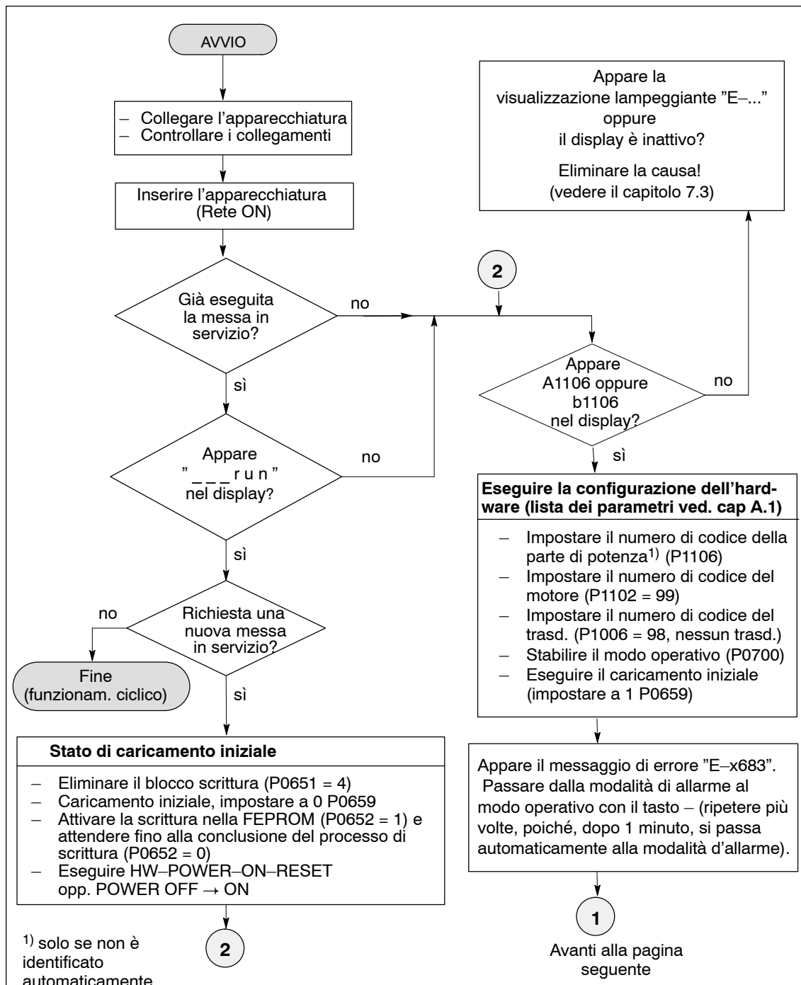
Fig. 4-7 Messa in servizio dei motori asincroni senza trasduttore (parte 1)
