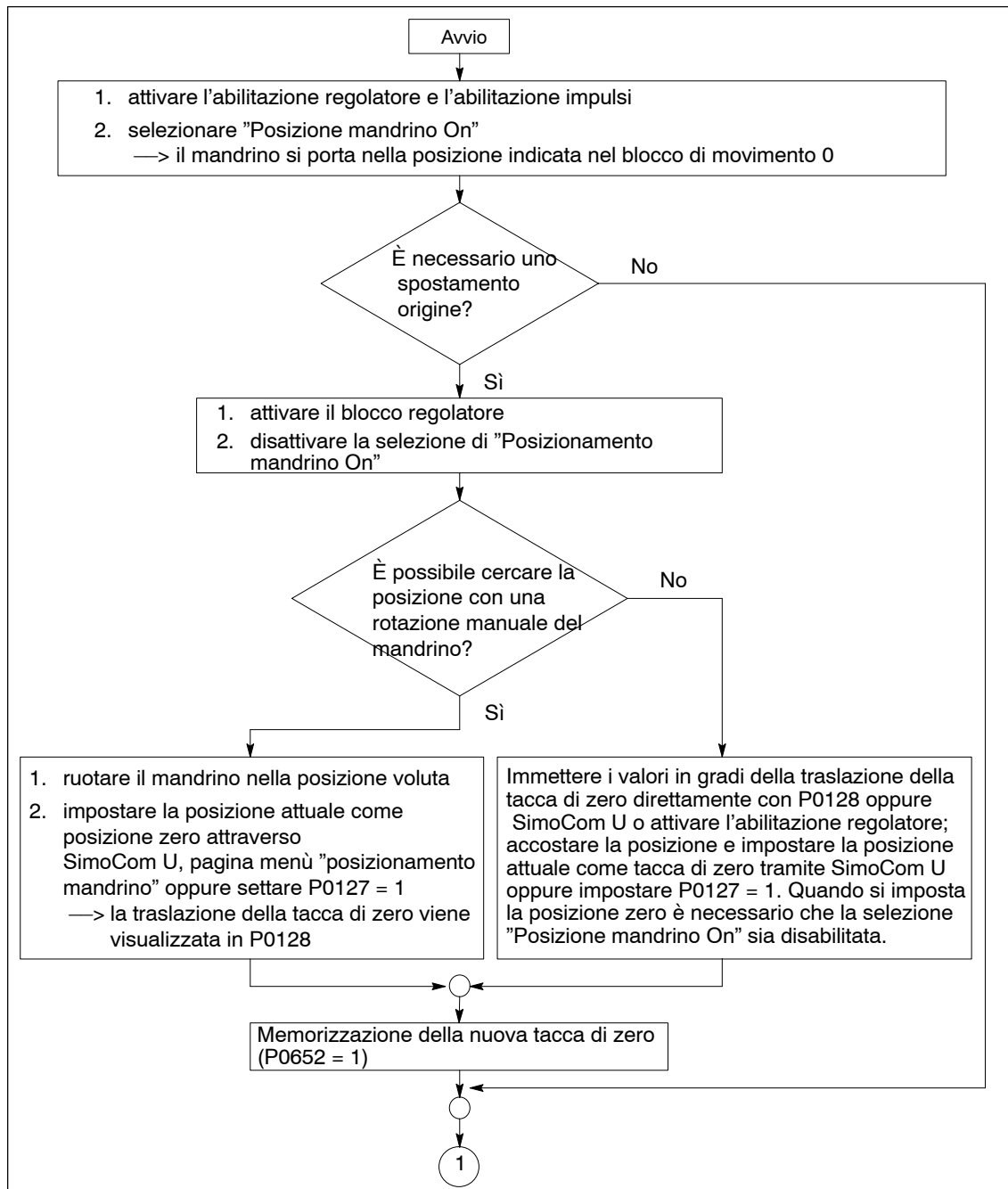
Fig. 6-89 Esempio di messa a punto del posizionamento mandrino
