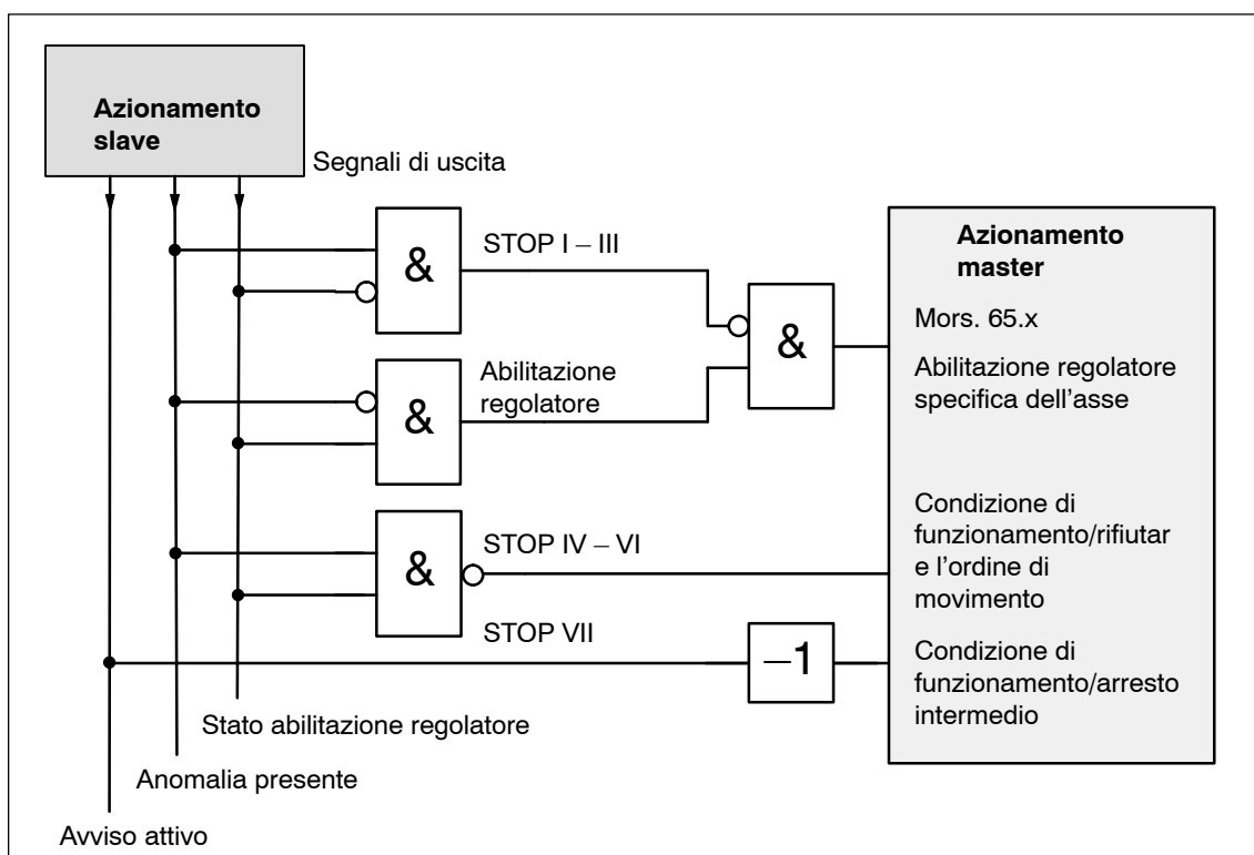
Fig. 6-42 Esempio: gestione delle anomalie nell'azionamento slave tramite l'azionamento master
