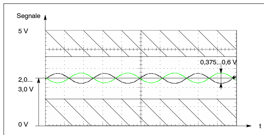
Fig. A-3 Andamento dei segnali in presenza dei segnali di traccia A+, A-, B+, B-, C+, C-, D+ e D-
