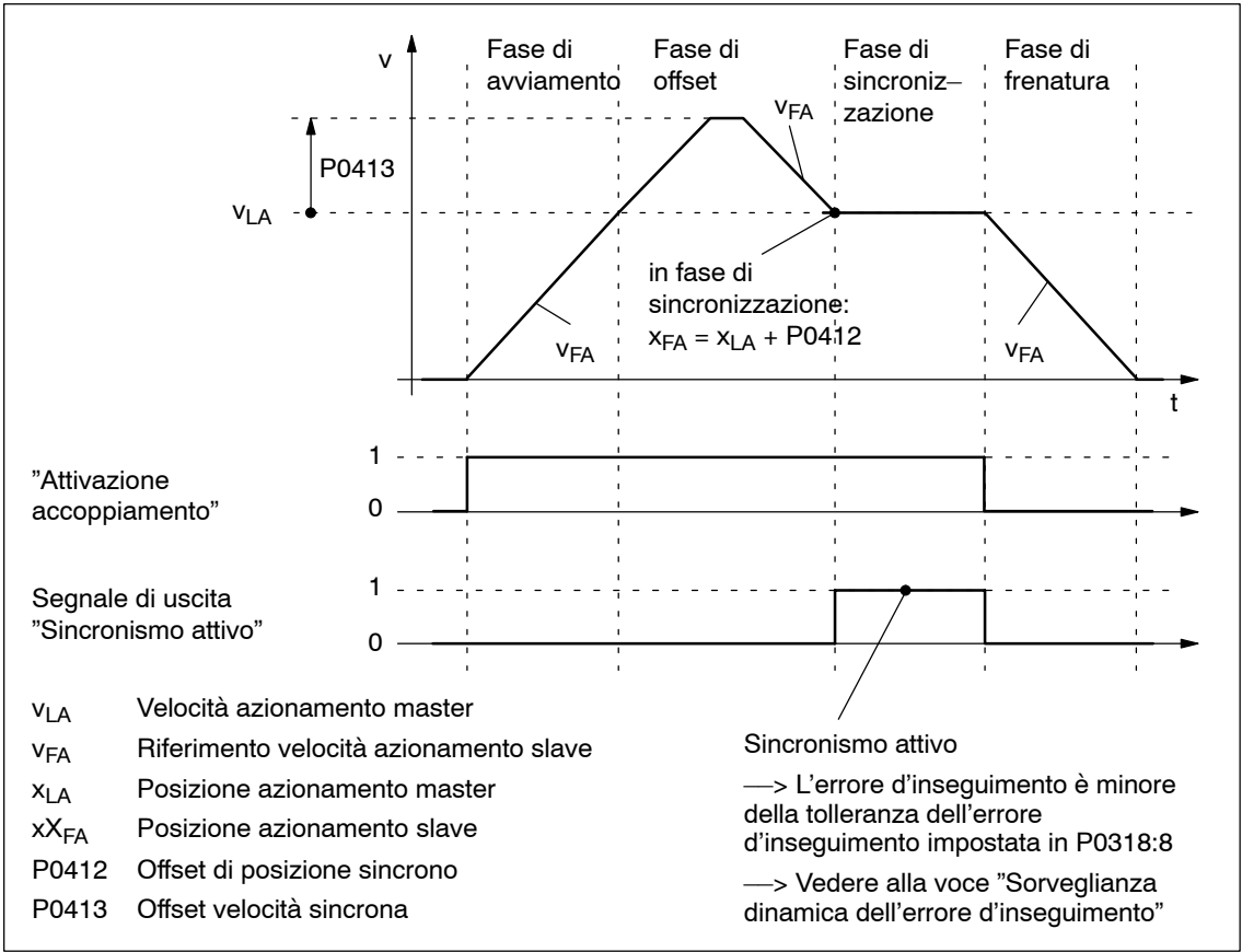
Fig. 6-37 Su posizione assoluta (P0410 = 7 o 8)
