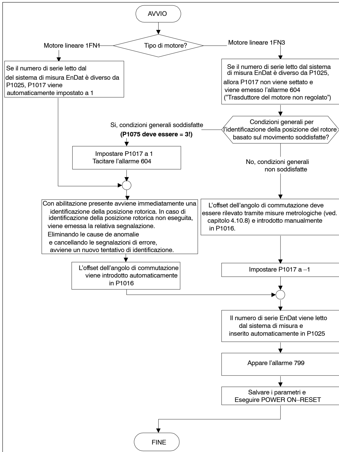
Fig. 4-13 Sistema di misura assoluto
