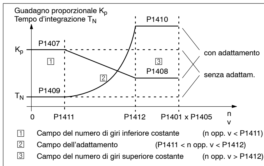
Fig. 6-6 Adattamento dei parametri del regolatore del numero di giri mediante la caratteristica
