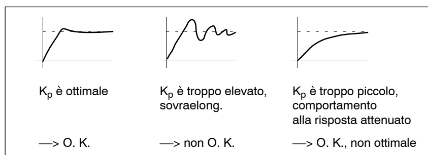
Fig. 4-11 Come si valuta la risposta al gradino?
