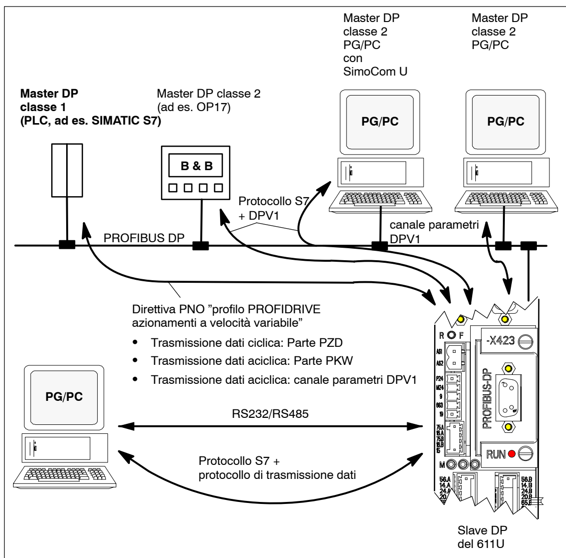
Fig. 5-2 Protocolli con lo "Slave DP del 611U"
