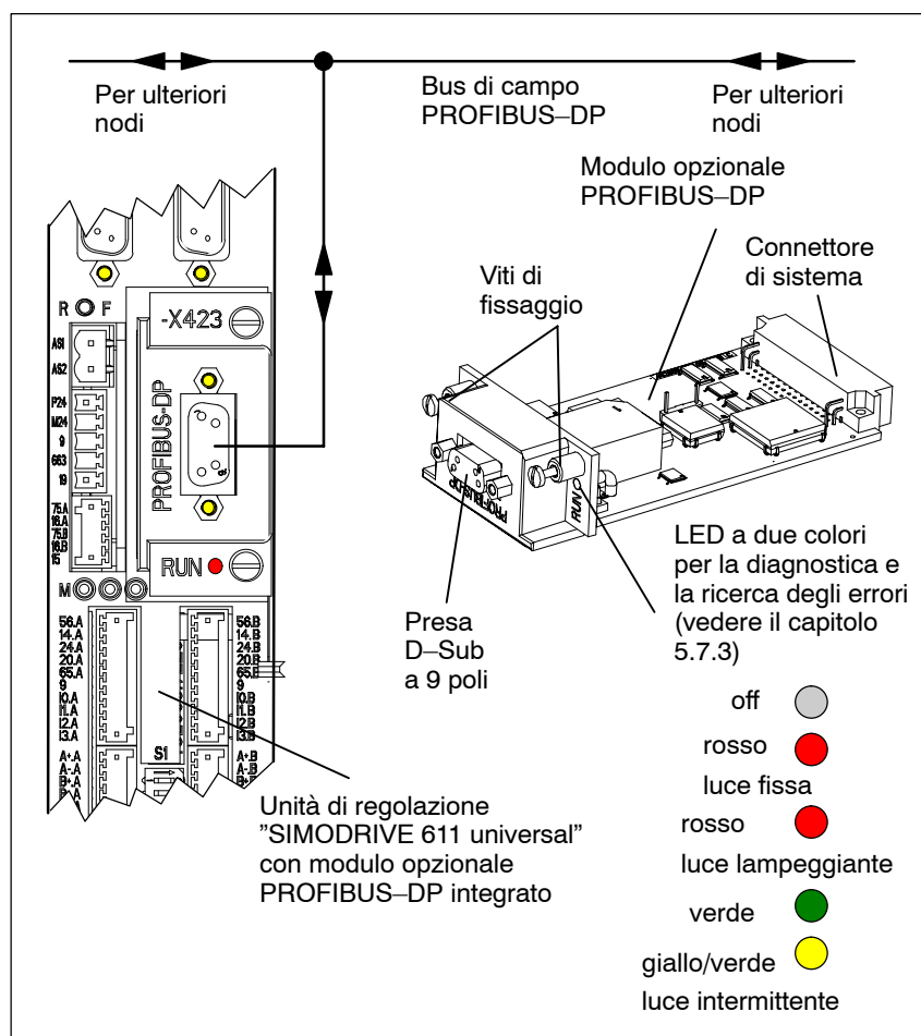
Fig. 5-3 "SIMODRIVE 611 universal" con modulo opzionale PROFIBUS-DP
