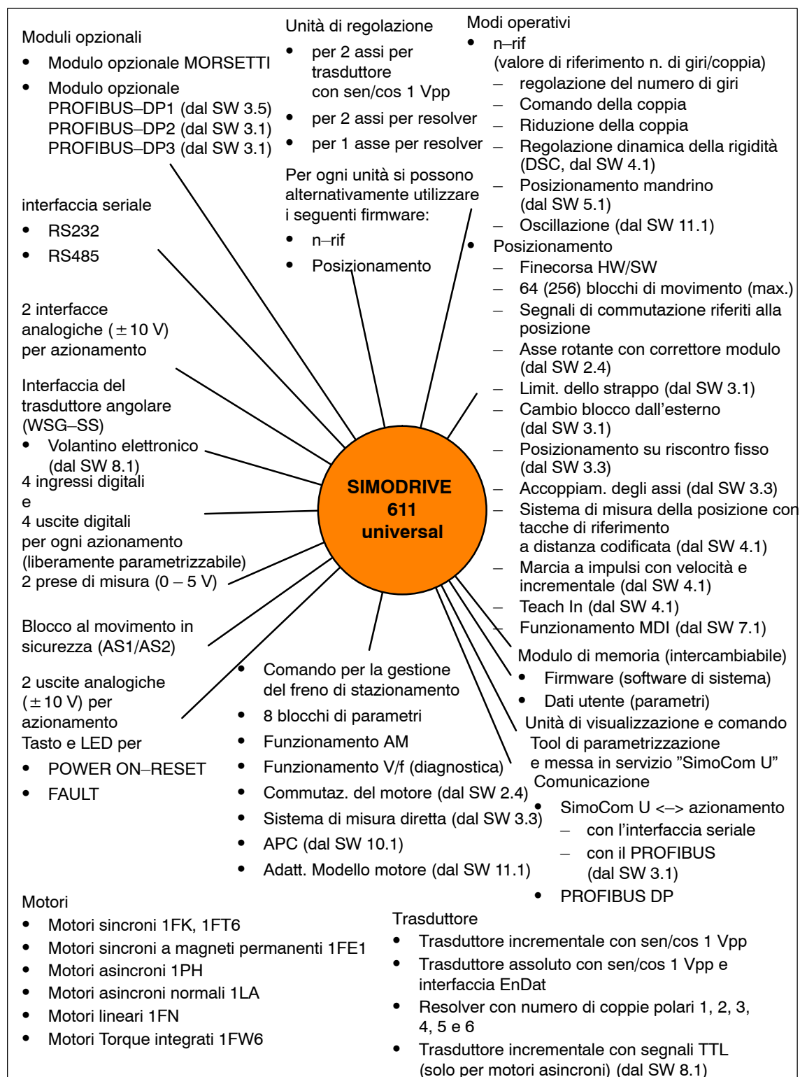
Fig. 1-1 Panoramica delle funzioni con il "SIMODRIVE 611 universal"
