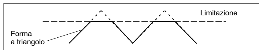
Fig. 7-5 Forma della curva a "triangolo" con picchi recisi
