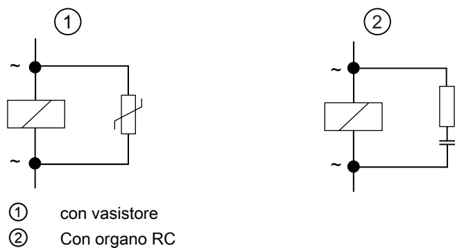
Figura 3-3 Circuito di bobine alimentate in corrente alternata
