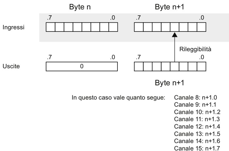
Figura 3-9 Rileggibilità delle uscite dell'SM 327; DI 8/DO 8 x DC 24 V/0,5 A
