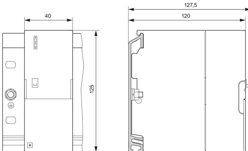
Figura C-10 Alimentatore PS 307; 2 A
