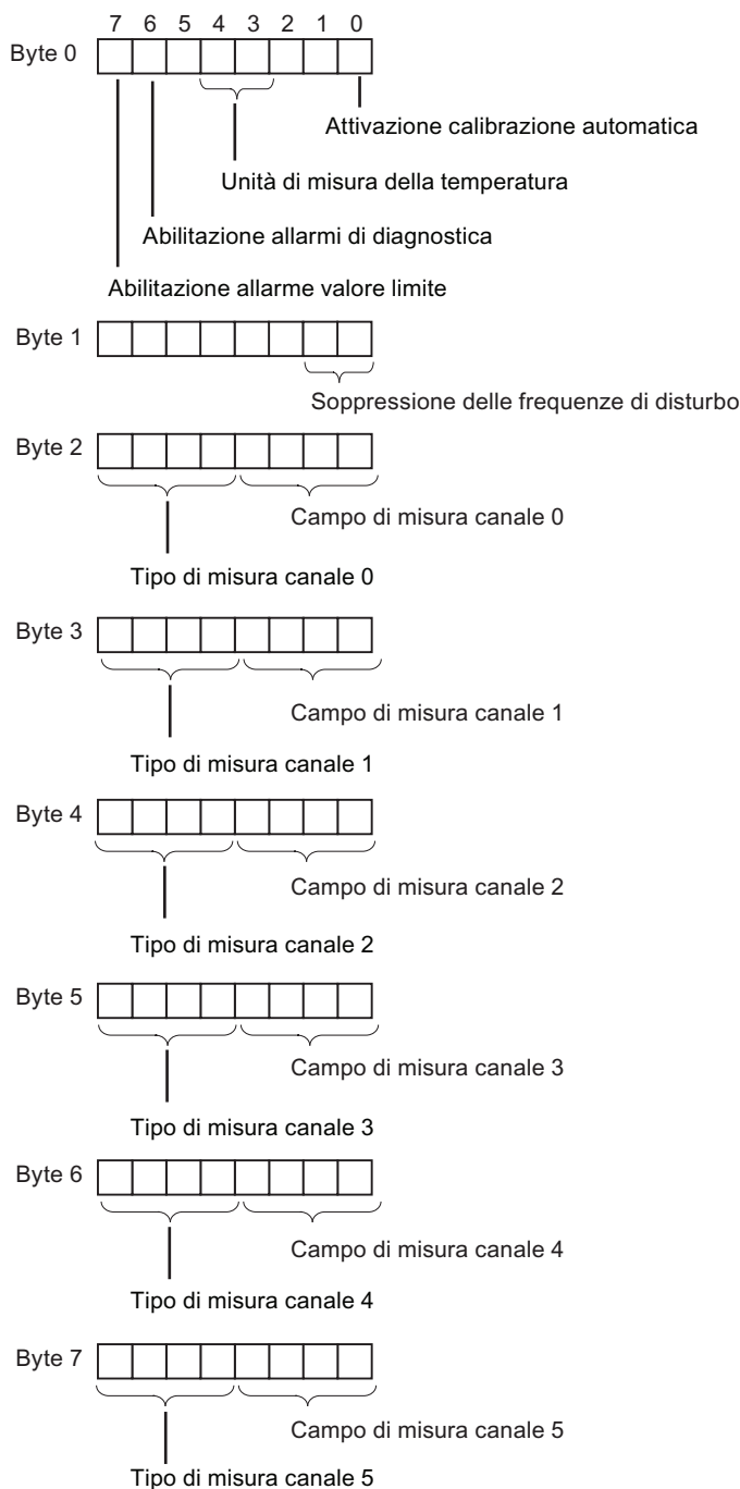
Figura A-21 Struttura del set di dati 1 per l'AI 6 x TC
