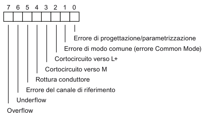
Figura B-7 Byte di diagnostica per un canale di ingresso analogico di un SM 331 con funzioni di diagnostica
