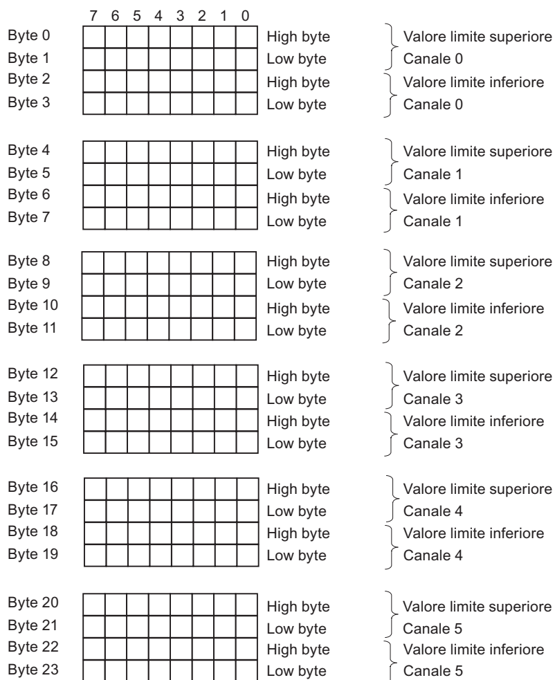
Figura A-23 Set di dati 128 per AI 6 x TC
