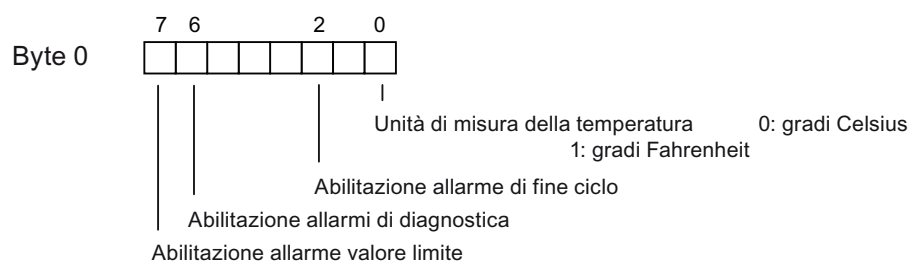
Figura A-5 Set di dati 1 dei parametri della SM 331; AI 8 x RTD
