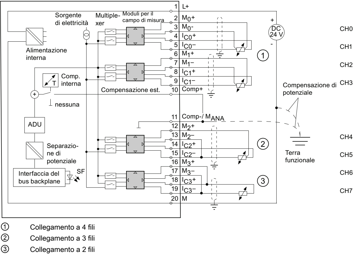
Figura 6-15 Schema di principio e di collegamento
