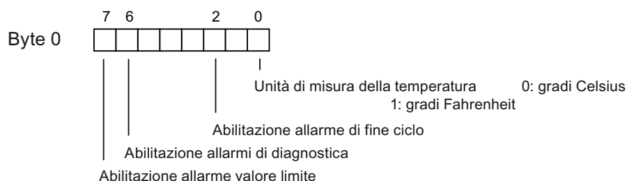
Figura A-10 Set di dati 1 dei parametri dell'SM 331; AI 8 TC
