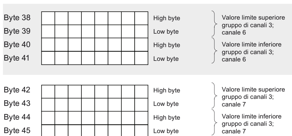
Figura A-20 Set di dati 128 per i parametri dell'SM 331; AI 8 x 16 bit (continuazione)
