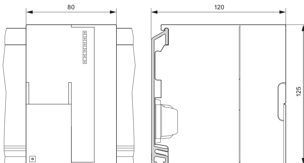
Figura C-16 Unità di interfaccia IM 361
