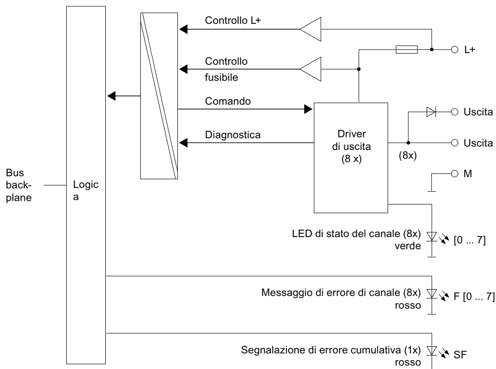
Figura 3-7 Schema di principio dell' SM 322; DO 8 x DC 24 V/0,5 A
