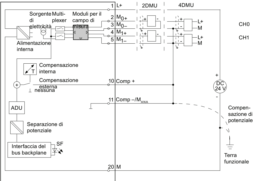
Figura 6-20 Schema di principio e di collegamento
