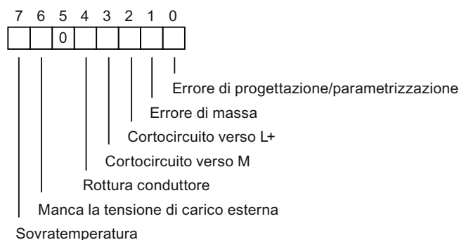
Figura B-6 Byte di diagnostica per un canale di uscita digitale dell'SM 322; DO 8 x DC 24 V/0,5 A
