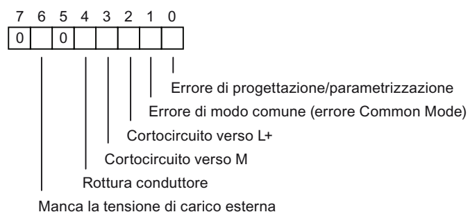
Figura B-8 Byte di diagnostica per un canale di uscita analogico dell' SM 332 con funzioni di diagnostica
