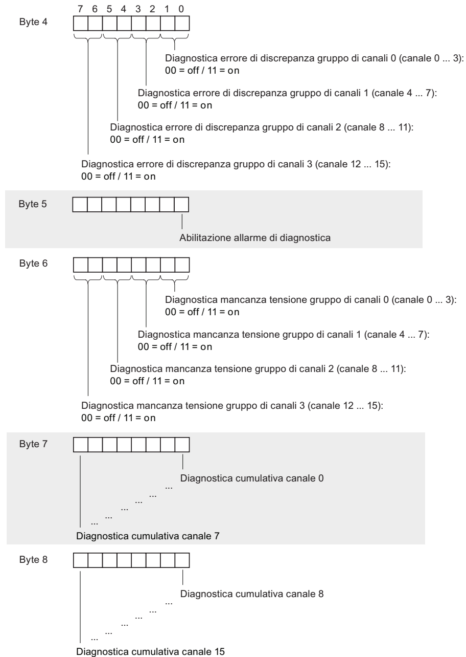
Figura A-3 Struttura del set di dati 1
