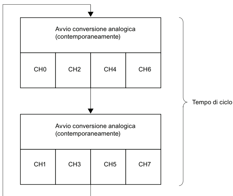
Figura 6-24 Tempo di ciclo modo a 8 canali (filtro software)
