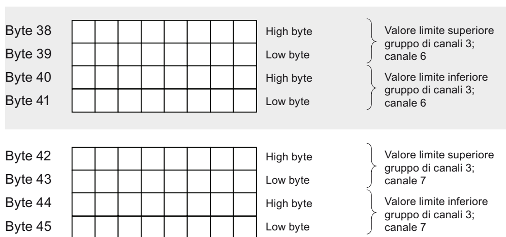
Figura A-9 Set di dati 128 dell'SM 331; AI 8 x RTD (continuazione)
