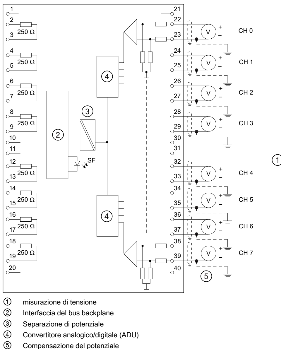
Figura 6-1 Schema di principio e di collegamento
