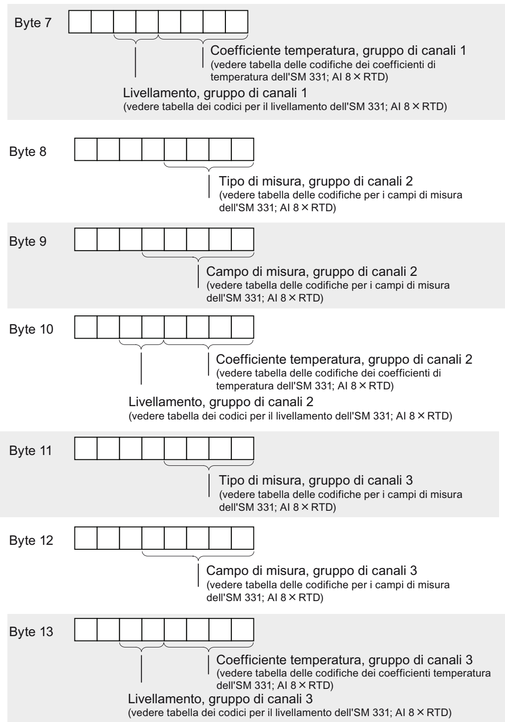
Figura A-7 Set di dati 128 dell'SM 331; AI 8 x RTD (continuazione)
