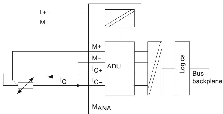
Figura 4-10 Collegamento a 3 fili di termoresistenze ad un'unità di ingresso analogica a separazione di potenziale
