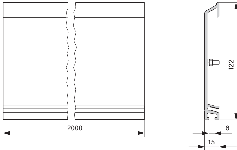
Figura C-9 Disegno quotato della guida profilata da 2000 mm
