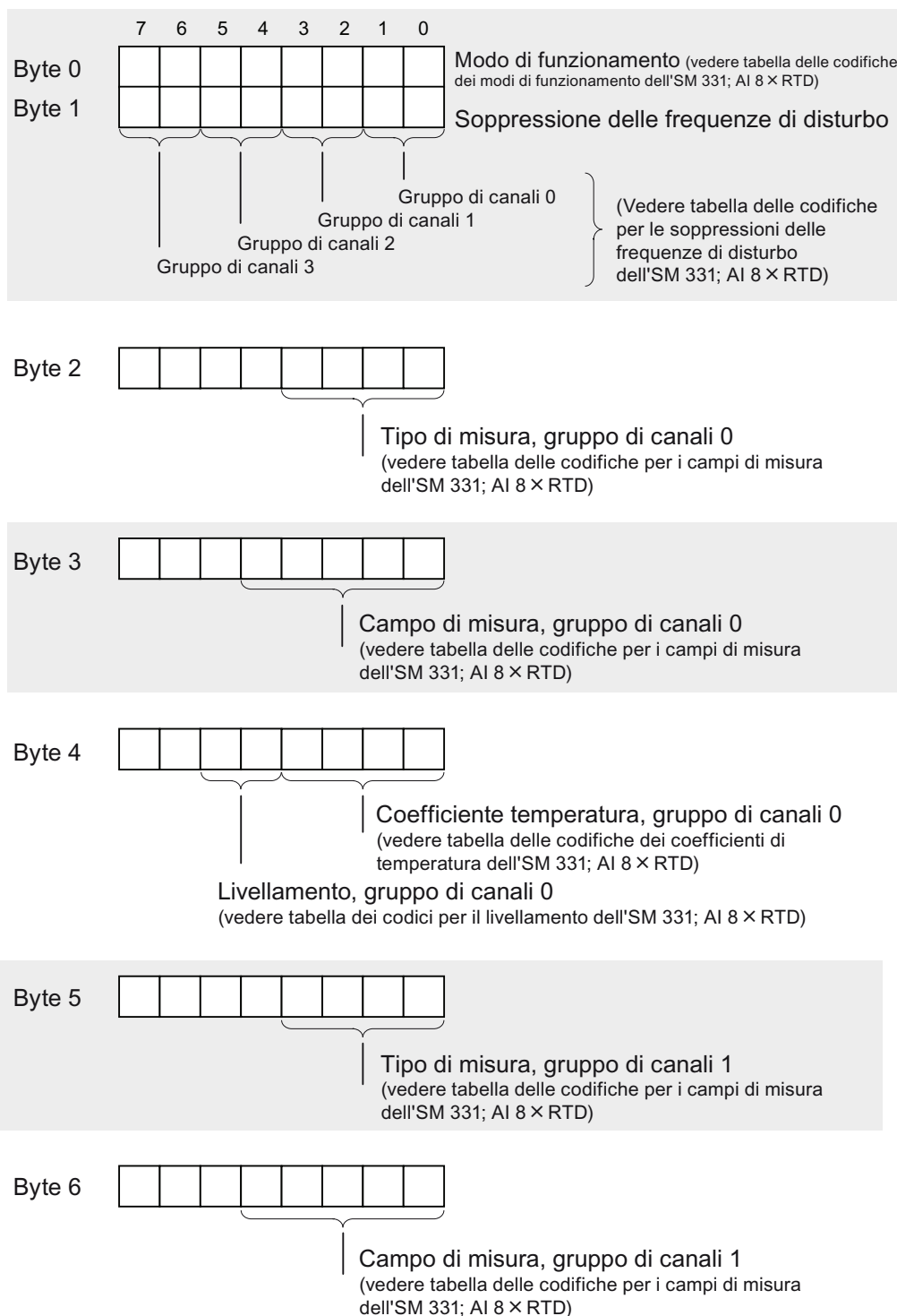
Figura A-6 Set di dati 128 dell'SM 331; AI 8 x RTD
