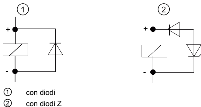
Figura 3-2 Circuito di bobine alimentate in continua
