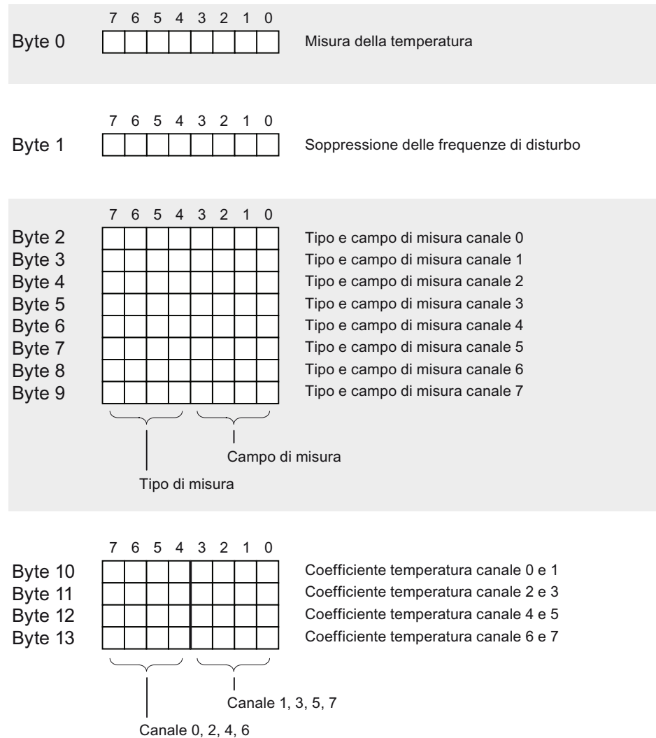
Figura A-15 Record di dati 1 per i parametri delle unità di ingresso analogiche
