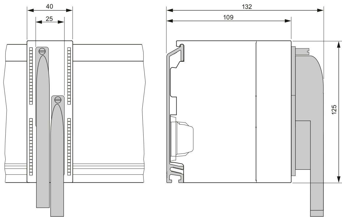
Figura C-19 Unità di ingresso/uscita a 64 canali
