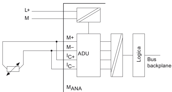
Figura 4-11 Collegamento a 2 fili di termoresistenze ad un'unità di ingresso analogica a separazione di potenziale
