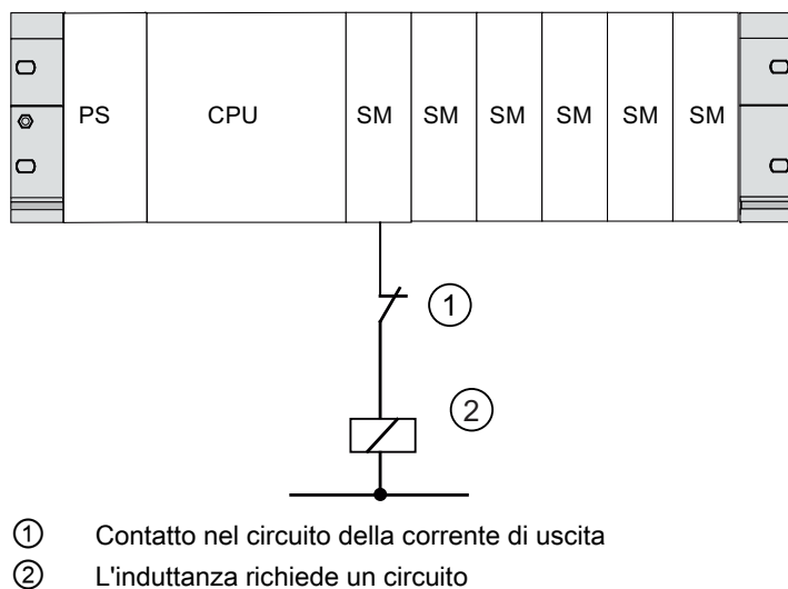
Figura 3-1 Contatto a relè per il circuito di corrente di uscita ARRESTO DI EMERGENZA
