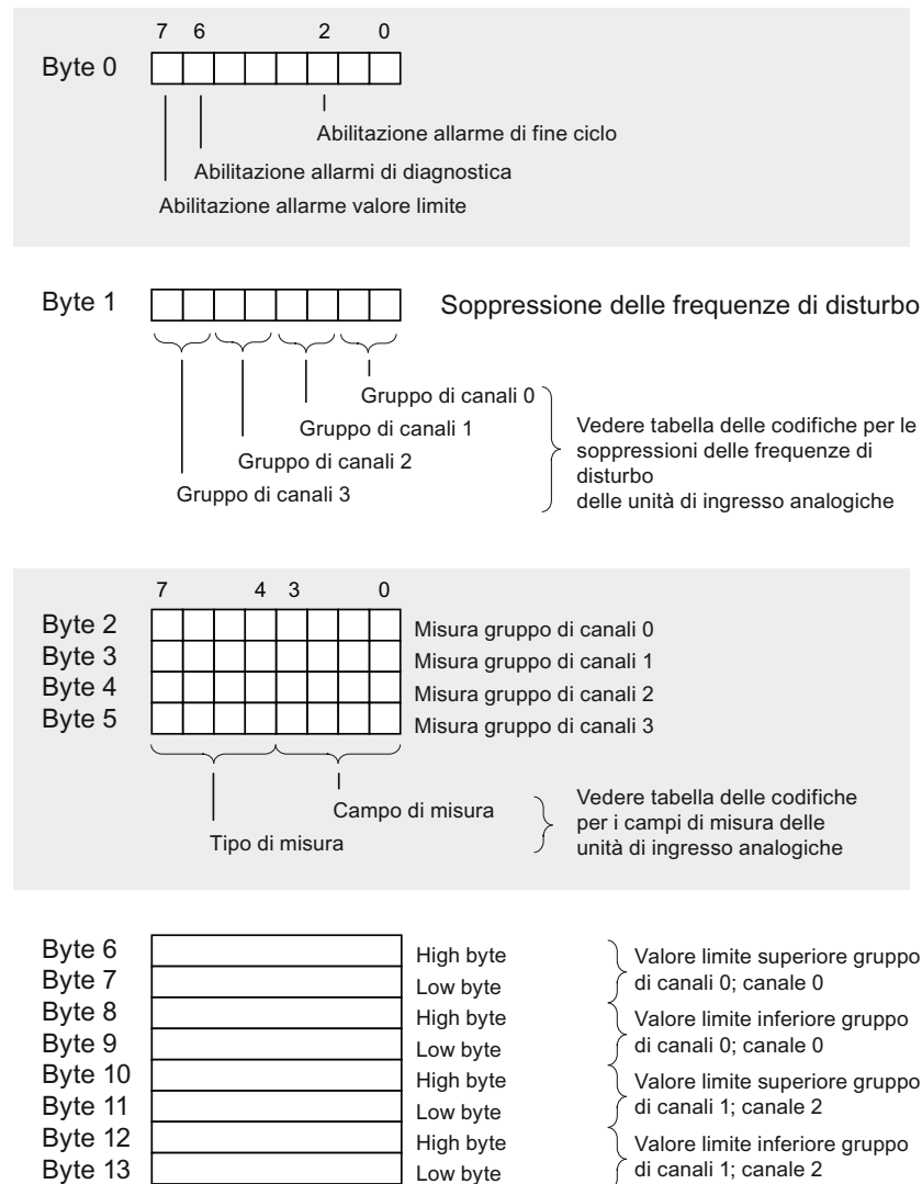
Figura A-4 Record di dati 1 per i parametri delle unità di ingresso analogiche
