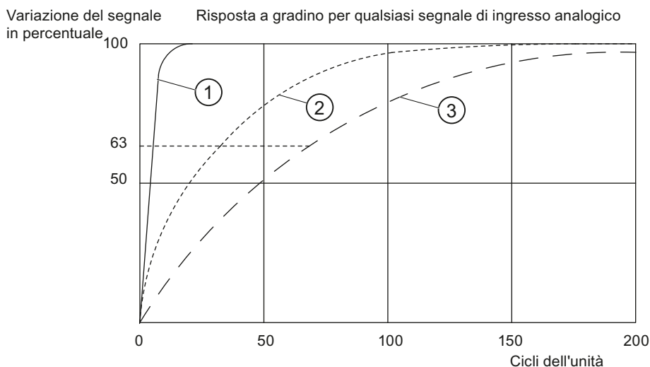
Figura 5-5 Esempio dell'influenza del livellamento sulla risposta a gradino del bit AI 8 x 14
