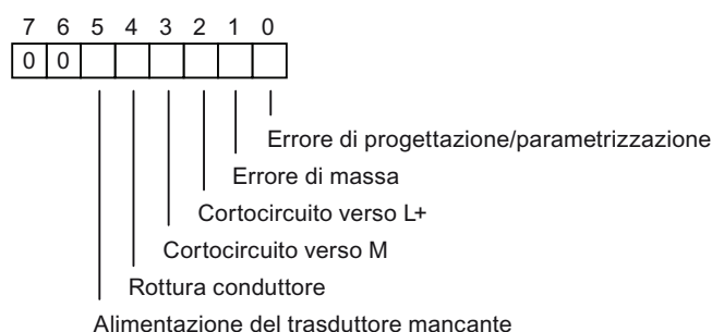
Figura B-5 Byte di diagnostica per un canale di ingresso di diagnostica dell'SM 321; DI 16 x DC 24 V
