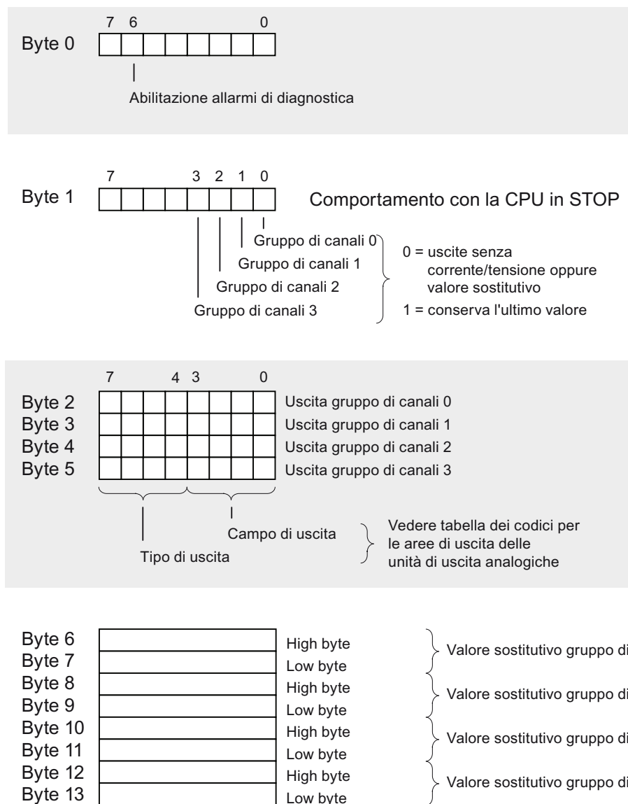
Figura A-24 Set di dati 1 dei parametri delle unità di uscita analogiche
