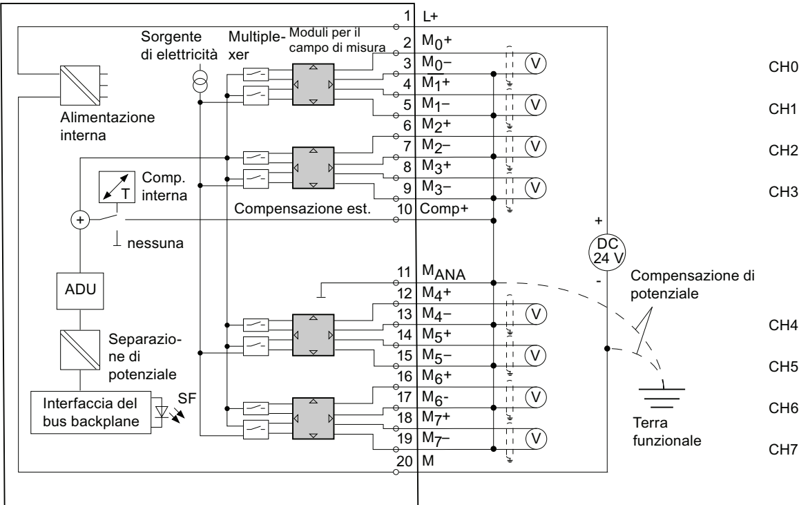
Figura 6-13 Schema di principio e di collegamento
