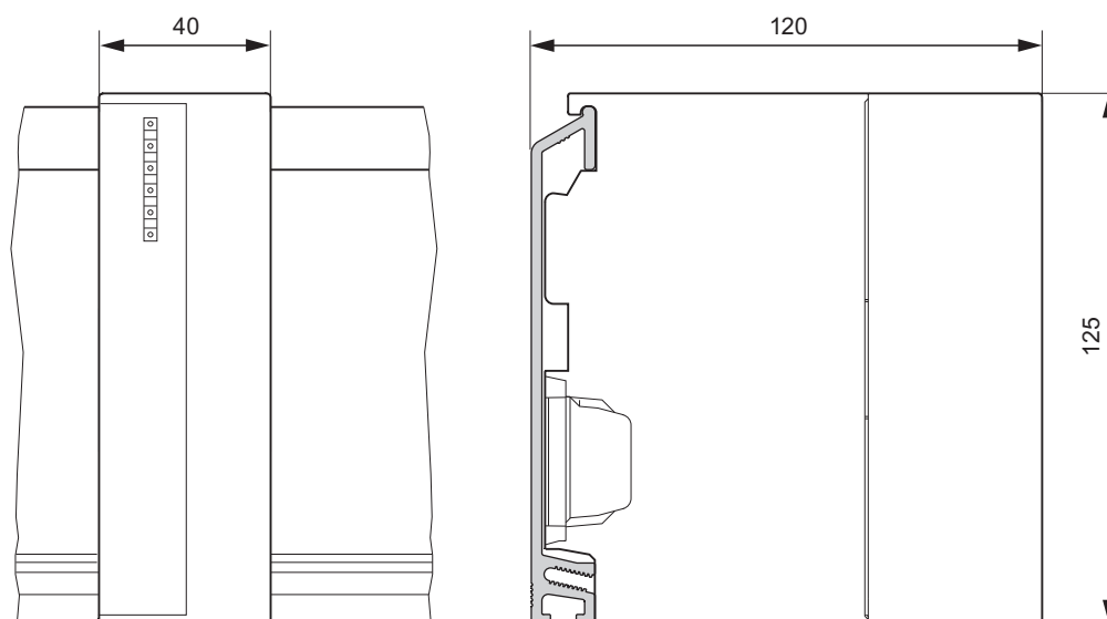
Figura C-15 Unità di interfaccia IM 360
