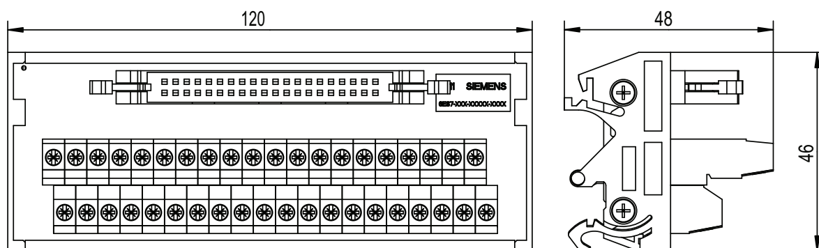
Figura C-21 Blocco terminale a 40 poli
