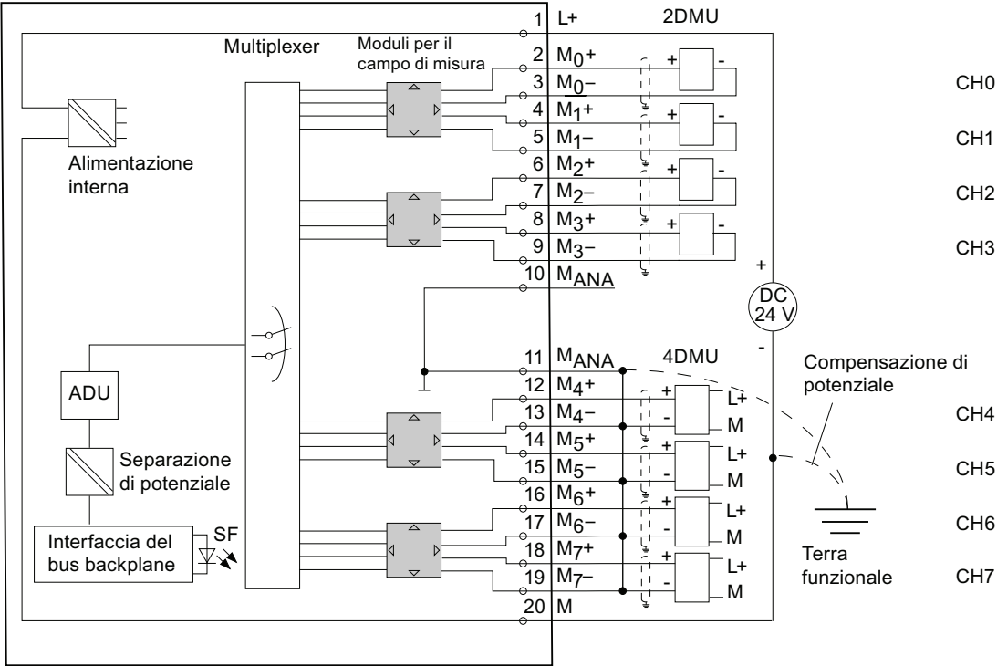
Figura 6-8 Schema di principio e di collegamento
