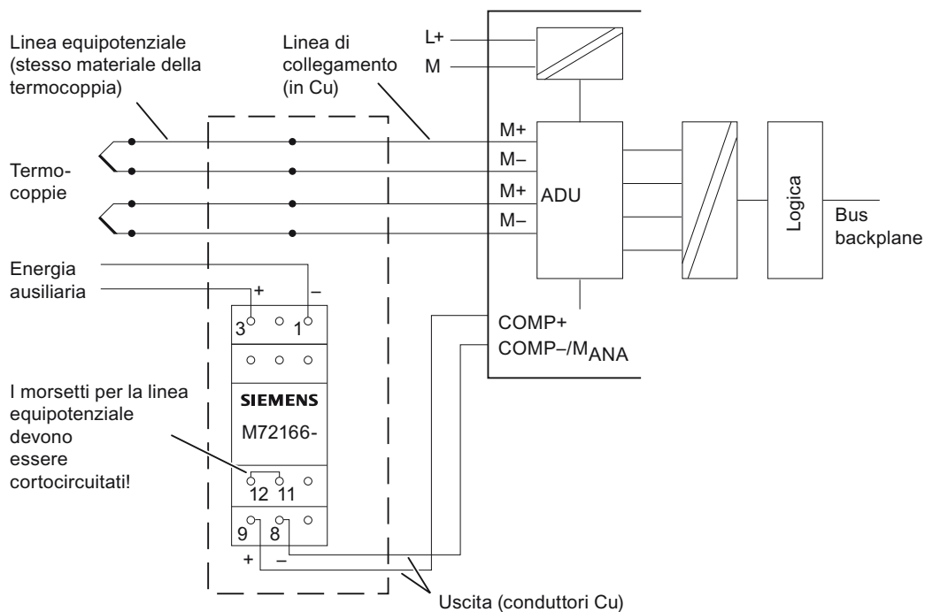
Figura 4-16 Collegamento di termocoppie con giunto freddo (N. di ordinazione M72166-xxx00)
