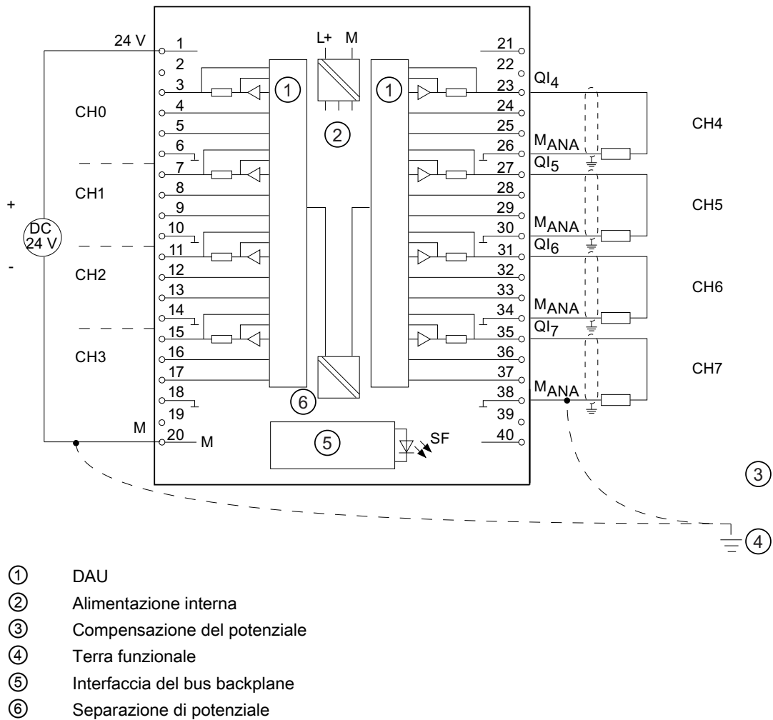
Figura 6-42 Schema di principio e di collegamento
