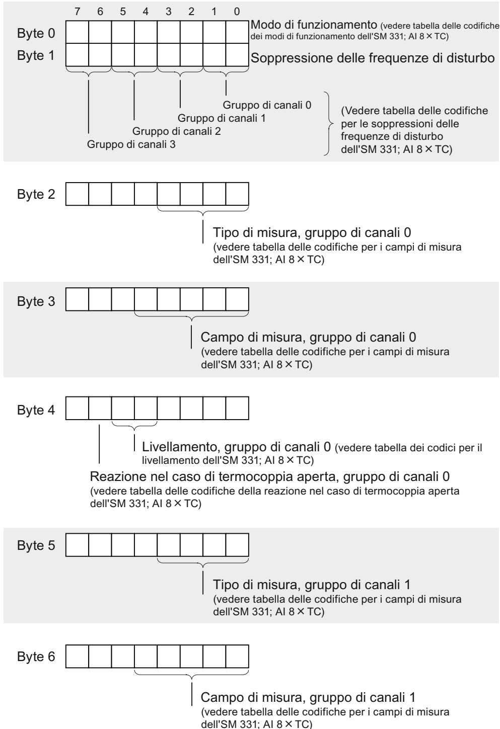
Figura A-11 Figura A-10 Set di dati 128 dell'SM 331; AI 8 x TC
