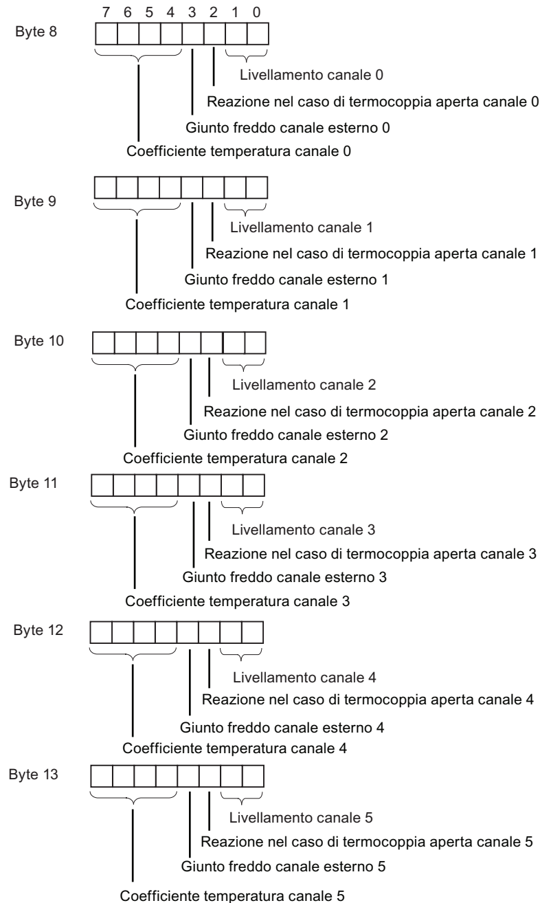
Figura A-22 Struttura del set di dati 1 per l'AI 6 x TC (seguito)
