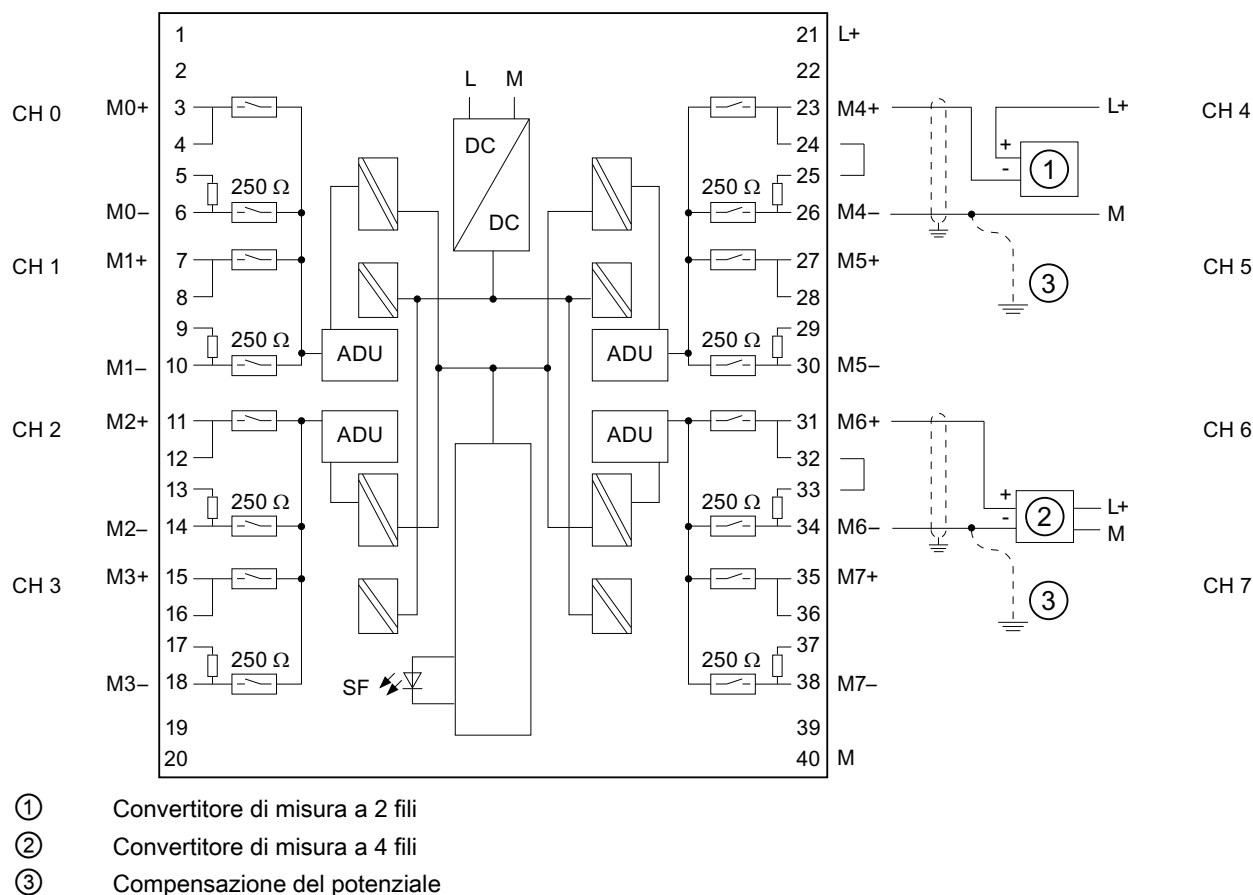
Figura 6-4 Schema di principio e di collegamento
