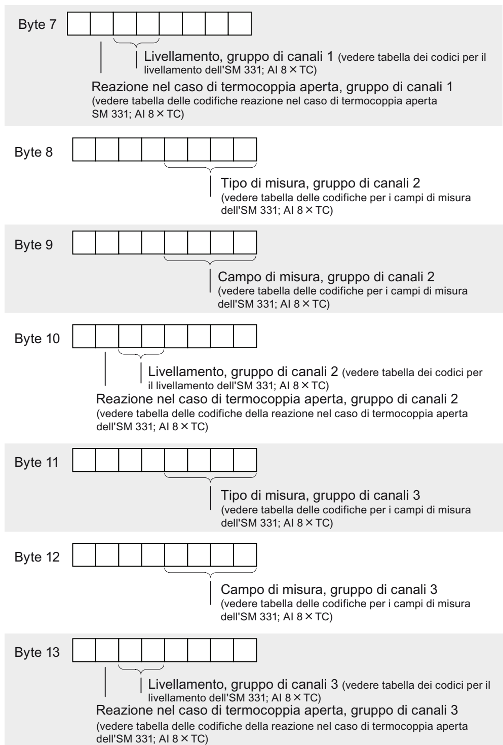
Figura A-12 Set di dati 128 dell'SM 331; AI 8 x TC (continuazione)
