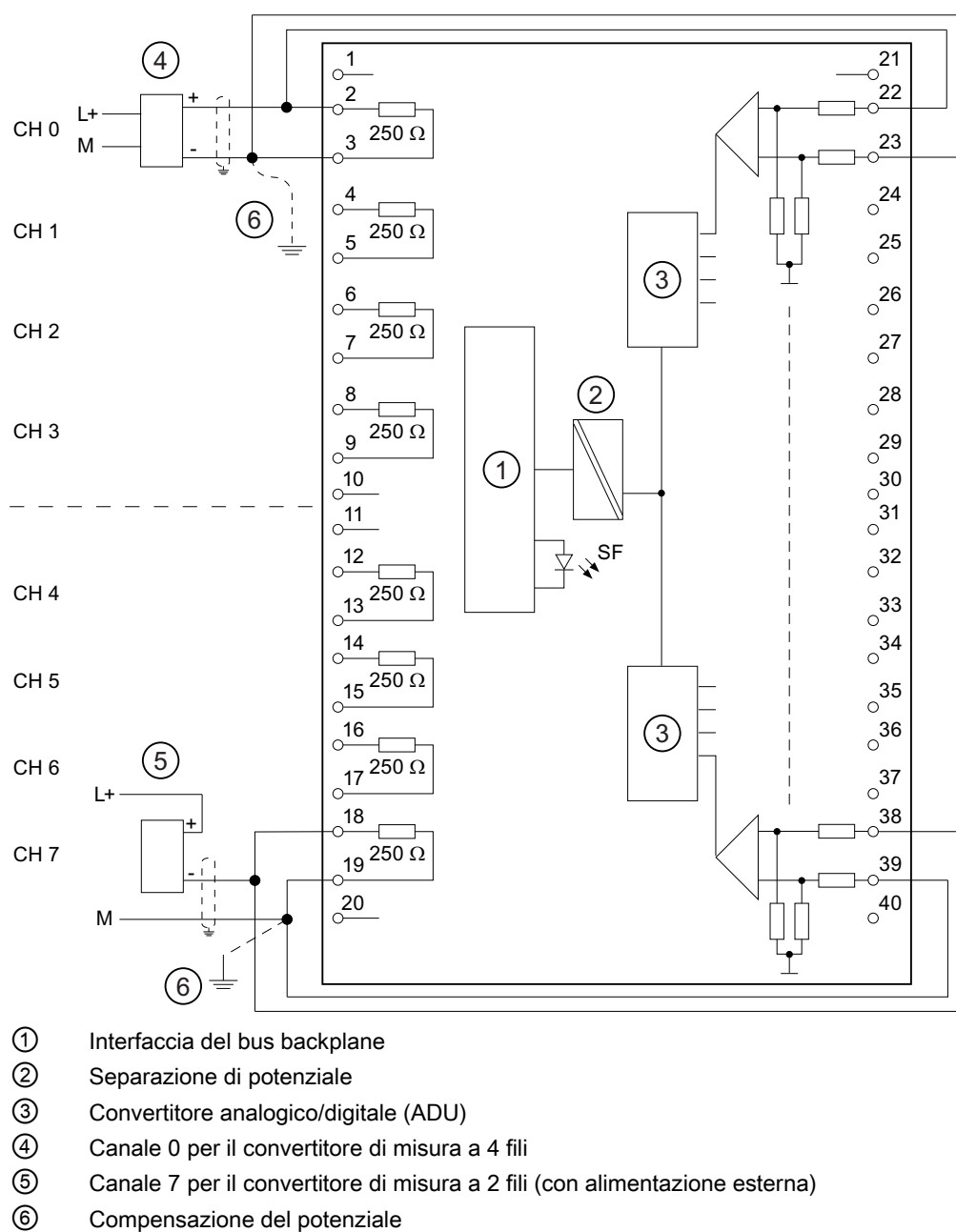
Figura 6-2 Schema di principio e di collegamento
