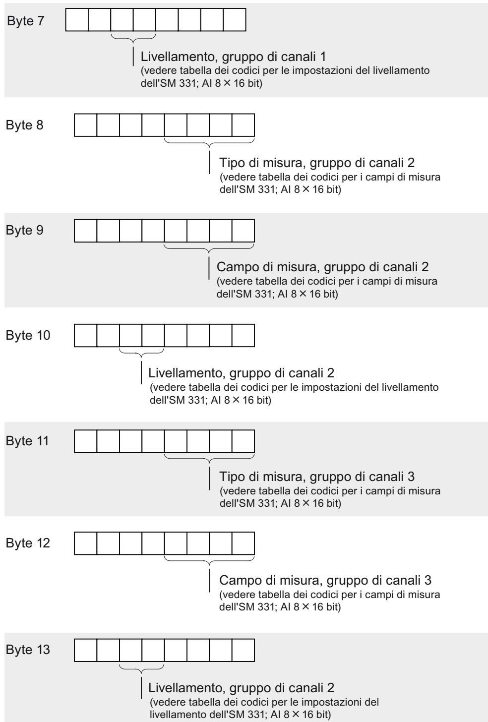
Figura A-18 Set di dati 128 per i parametri dell'SM 331; AI 8 x 16 bit (continuazione)
