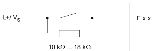
Figura 3-5 Schema di collegamento per il circuito delle resistenze dei trasduttori SM 321; DI 16 DC 24 V
