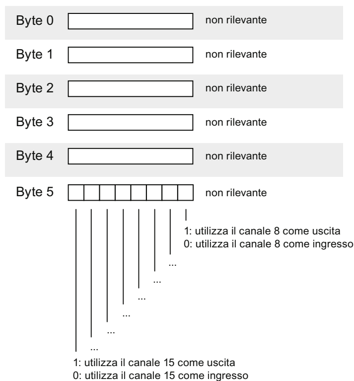
Figura 3-8 Set di dati 1 dell'SM 327; DI 8/DO 8 x DC 24 V/0,5 A
