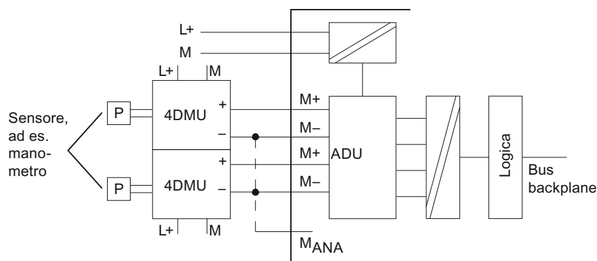
Figura 4-8 Collegamento di convertitori di misura a 4 fili ad un'unità di ingresso analogica a separazione di potenziale
