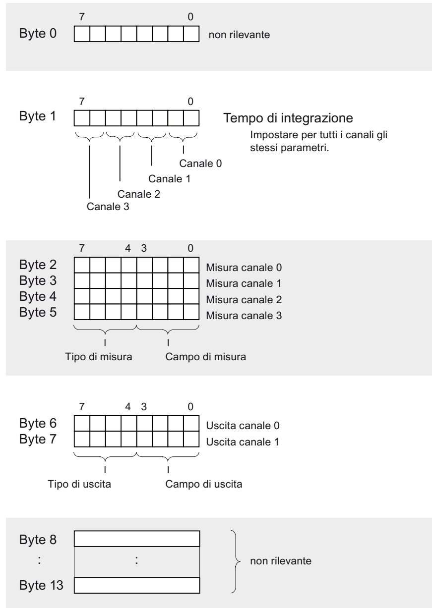
Figura A-26 Set di dati 1 dei parametri delle unità di ingresso/uscita analogiche
