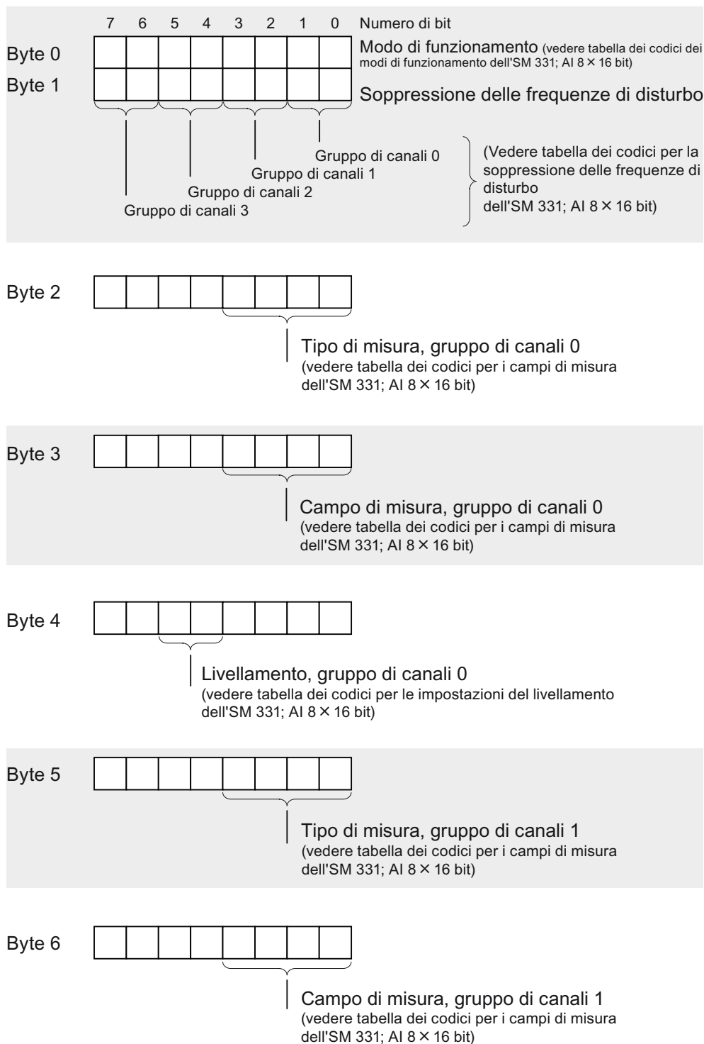
Figura A-17 Set di dati 128 per i parametri dell'SM 331; AI 8 x 16 bit
