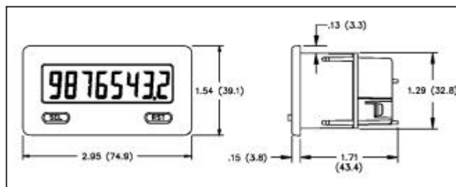
Abmessungen
