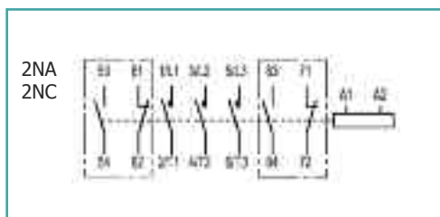
Schema elettrico contattori SC E5, E6, E7, N8, N10, N11, N12, N14, N16
