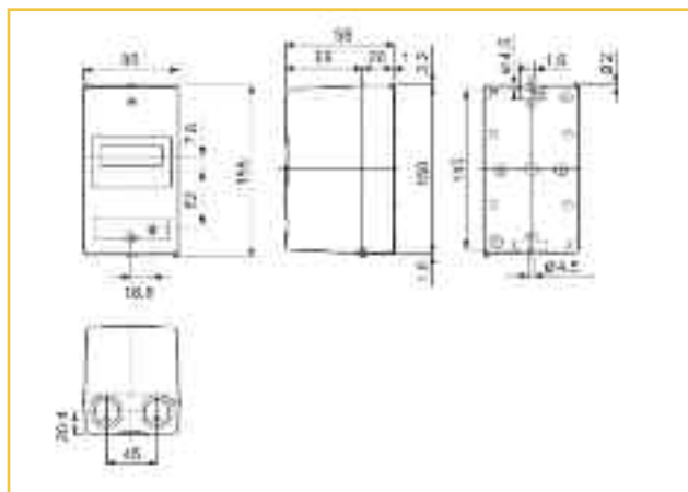
Custodia montaggio piastra CSBM3-41, CSBM3-55
