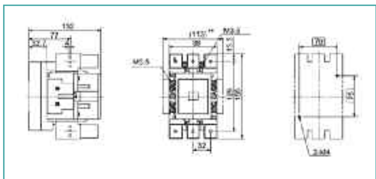
SC E5 AC/DC
