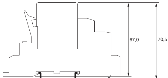
P2RF-□-E
