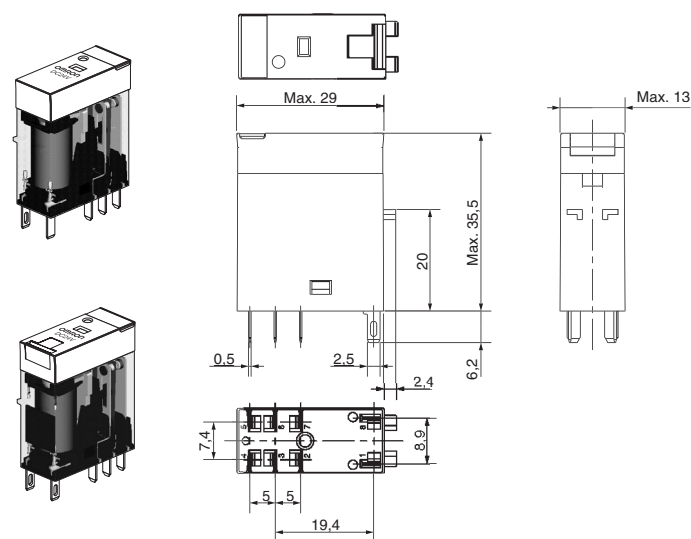
G2R-2-S
