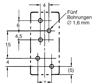
Befestigungsbohrungen
