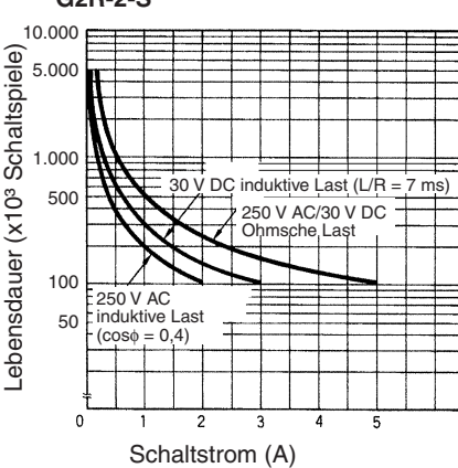
G2R-2-S
