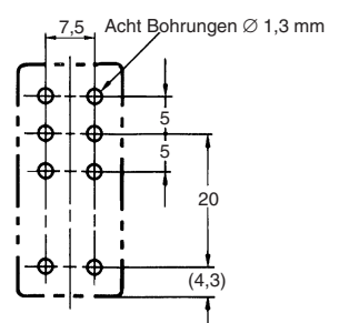
Befestigungsbohrungen
