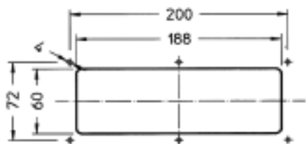
Particolare della foratura delle flange.
