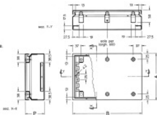
Posizione dei fori nella parte posteriore.
