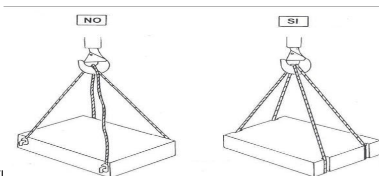
FIG.3 TIRANTI INCROCIATI
