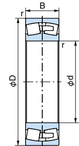
Foro interno cilindrico
