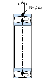
Con fori e scanalature per l'olio (W33)
