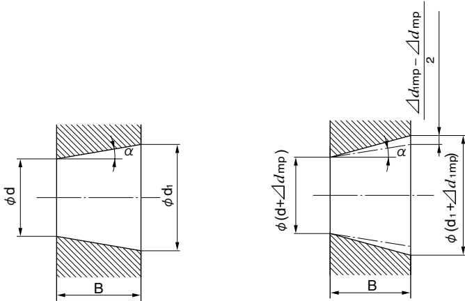
Foro interno conico teorico
