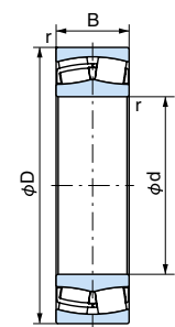
Foro interno cilindrico
