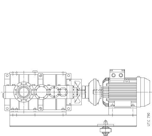
Sistema di reazione (cap. 15) semielastico ed economico: con bullone a molle a tazza, con bullone a molle a tazza con forcina.
