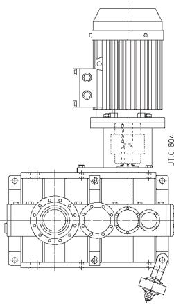
Sistema di reazione (cap. 15) semielastico ed economico: con bullone a molle a tazza, con bullone a molle a tazza con forcina.
